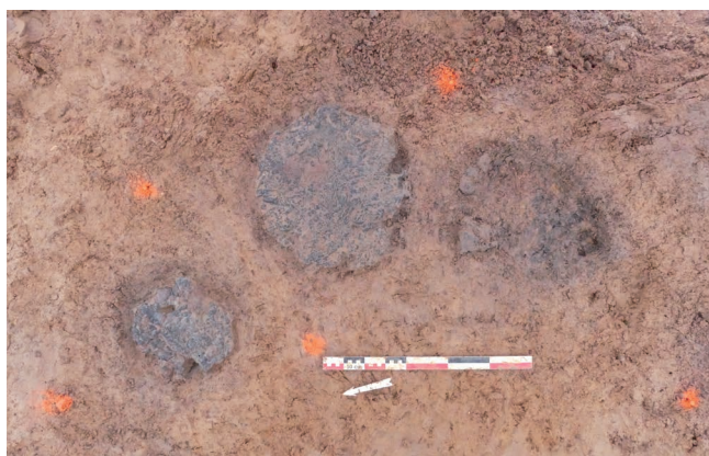
Fig.2 : Donnemain-Saint-Mamès (Eure-et-Loir) la Bruyère-Ouest : scories en place au fond des fours de réduction. (R. Wassong, Éveha)
