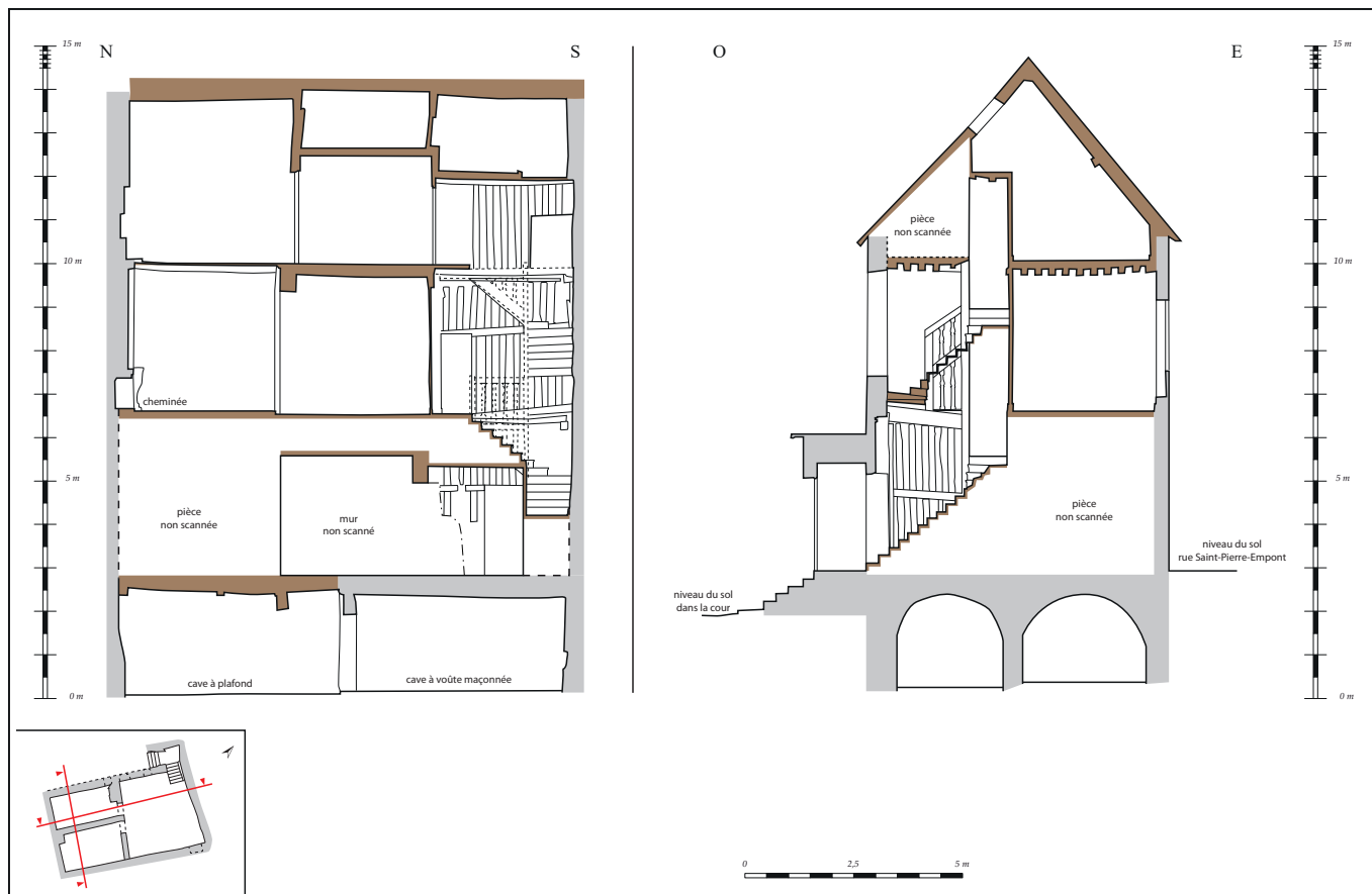
Fig. 3 : Orléans (Loiret) caves du centre-ville : coupes transversale et longitudinale de la maison 10 rue des Pastoureaux / 9 venelle Saint-Pierre-Empont (SICAVOR n° 409) édifée vers 1174. (D. Morleghem, Pôle d'Archéologie d'Orléans)
