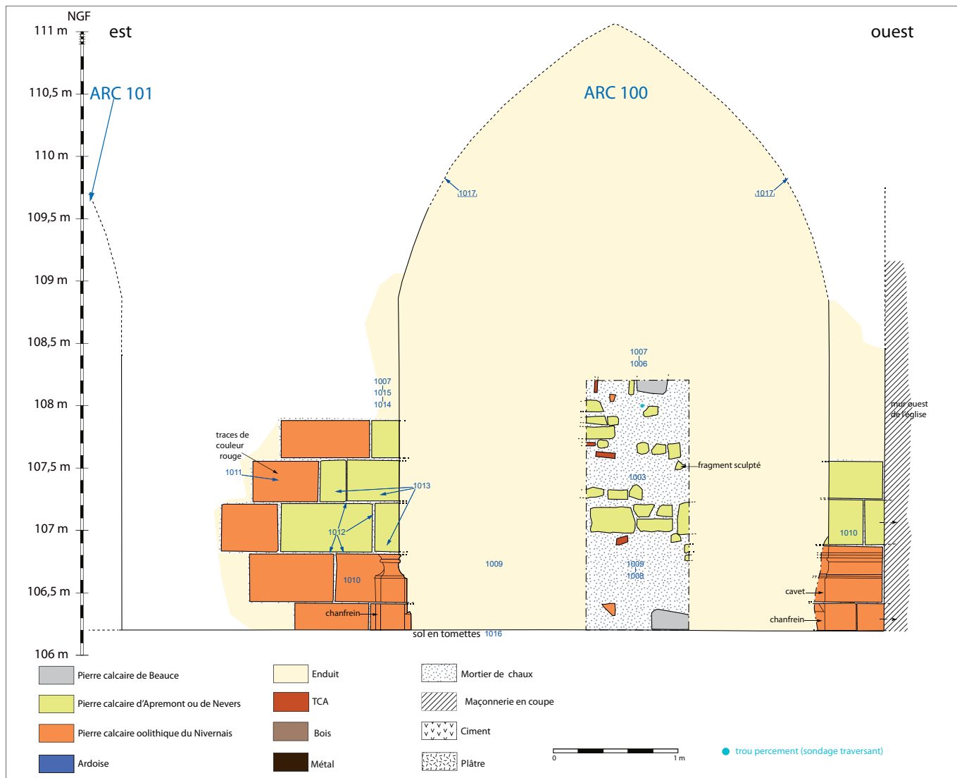
Fig. 2 : Orléans (Loiret) cloître Saint-Aignan : relevé en élévation de la face nord du mur (arcade ouest ARC 100) depuis l'intérieur du transept et caractérisation des matériaux. (C. Alix, A. Ladam, Pôle d'Archéologie d'Orléans)
