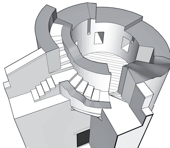
Fig. 2 : Dordives (Loiret) château de Mez-le-Maréchal : restitution écorchée des paliers et des volées de marches. (Michel Piechaczyk, ADM)
