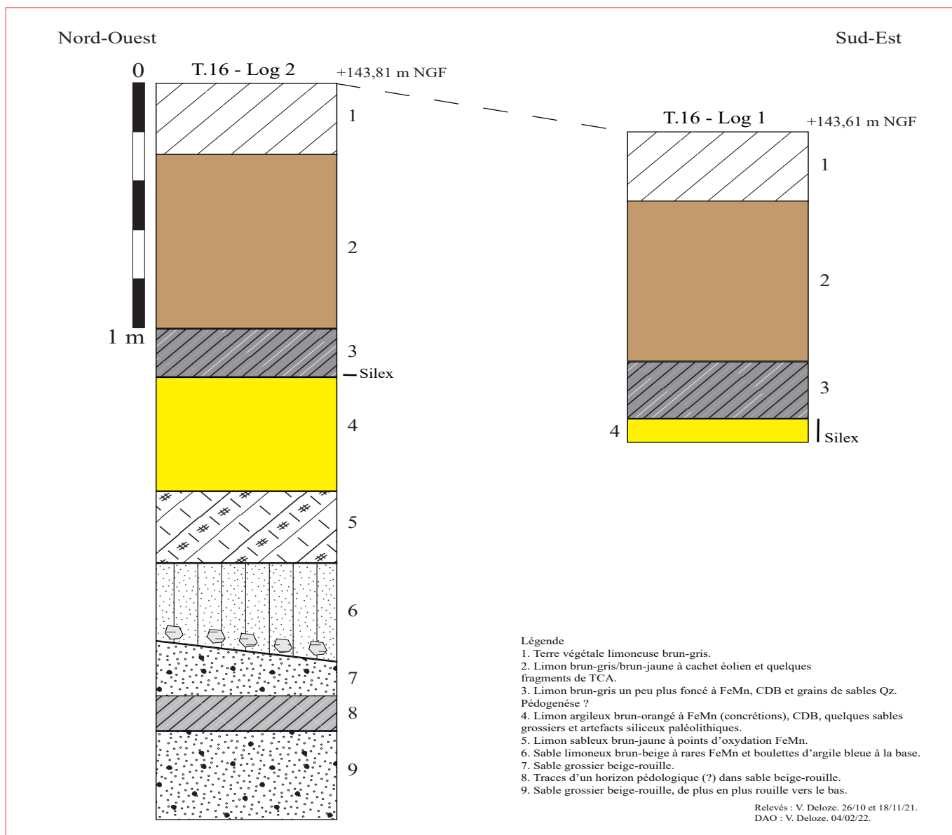
Beauvilliers (Eure-et-Loir) La Fosse-Aubert, tranche 5 B : transect géologique de la tranchée 16. (V. Deloze, Inrap)
