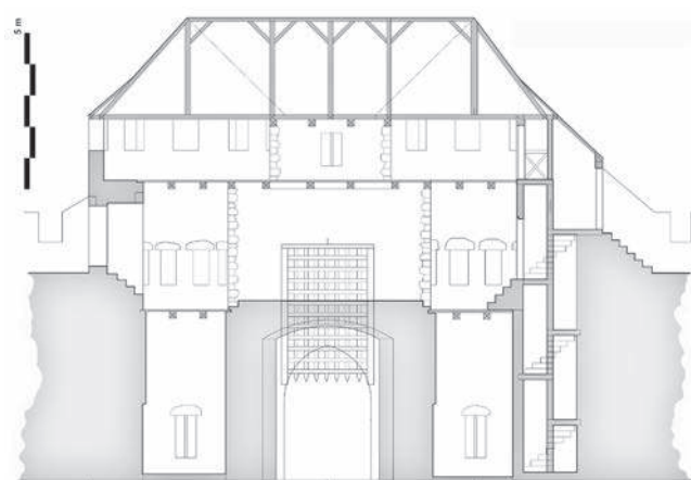
Fig. 3 : Dordives (Loiret) château de Mez-le-Maréchal : coupe frontale restitutive de la porterie (tours T5 et T6). (Michel Piechaczyk, Les Amis du Mez)
