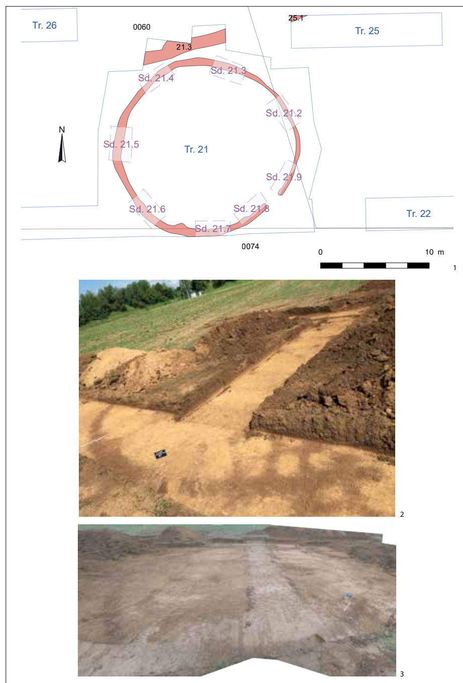
BUCHÈRES, Seyemont, chemin rural 11 Enclos circulaire de la tranchée 21. 1 : plan général ; 2 : vue en direction du nord-ouest ; 3 : vue en direction du nord, après décapage intégral (clichés : S. GRISARD, M. KASPRZYK)
