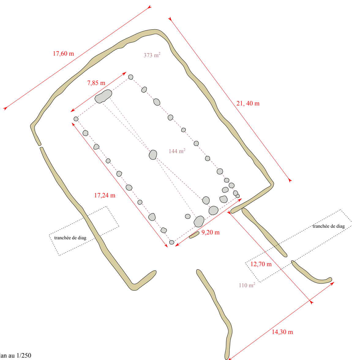
LA-VILLENEUVE-AU-CHÂTELOT, Les Communes, Les Grands Hauts du Frêne, phases 2b1, 3-1 et 3-2 Localisation du bâtiment monumental UA 20 en zone 3-2 (cliché : Drone-Developpement, DAO : S. POIRIER, C. CHOIMET)
