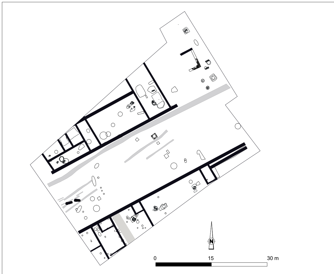
TROYES, 94 mail des Charmilles, 5 rue André Mutter Levé topographique (relevé : S. GRISARD, Inrap ; DAO : E. CHIRON)
