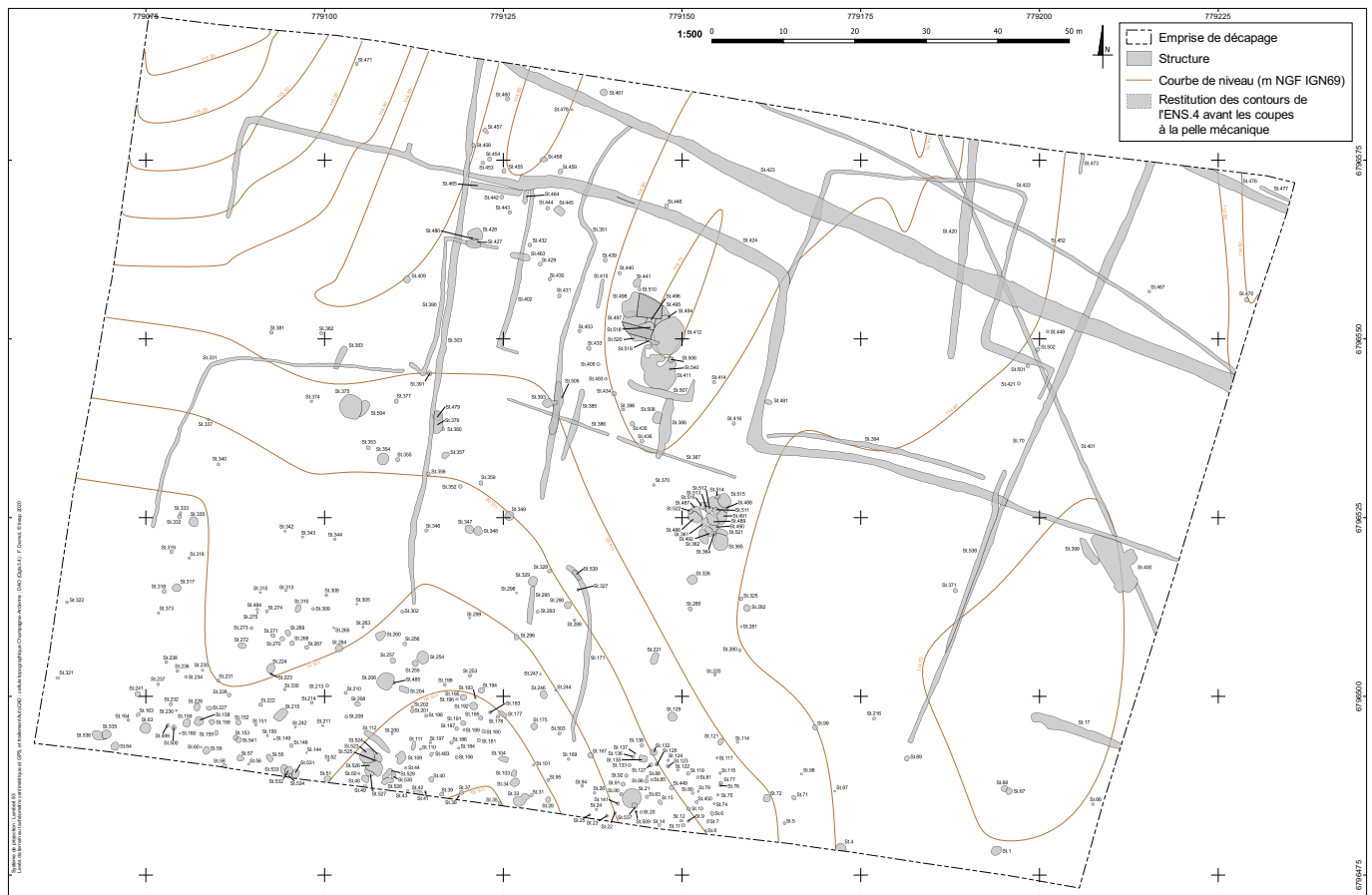
ROSIÈRES-PRÈS-TROYES, La Bouverie Plan général de la fouille (DAO : F. DEMOL)
