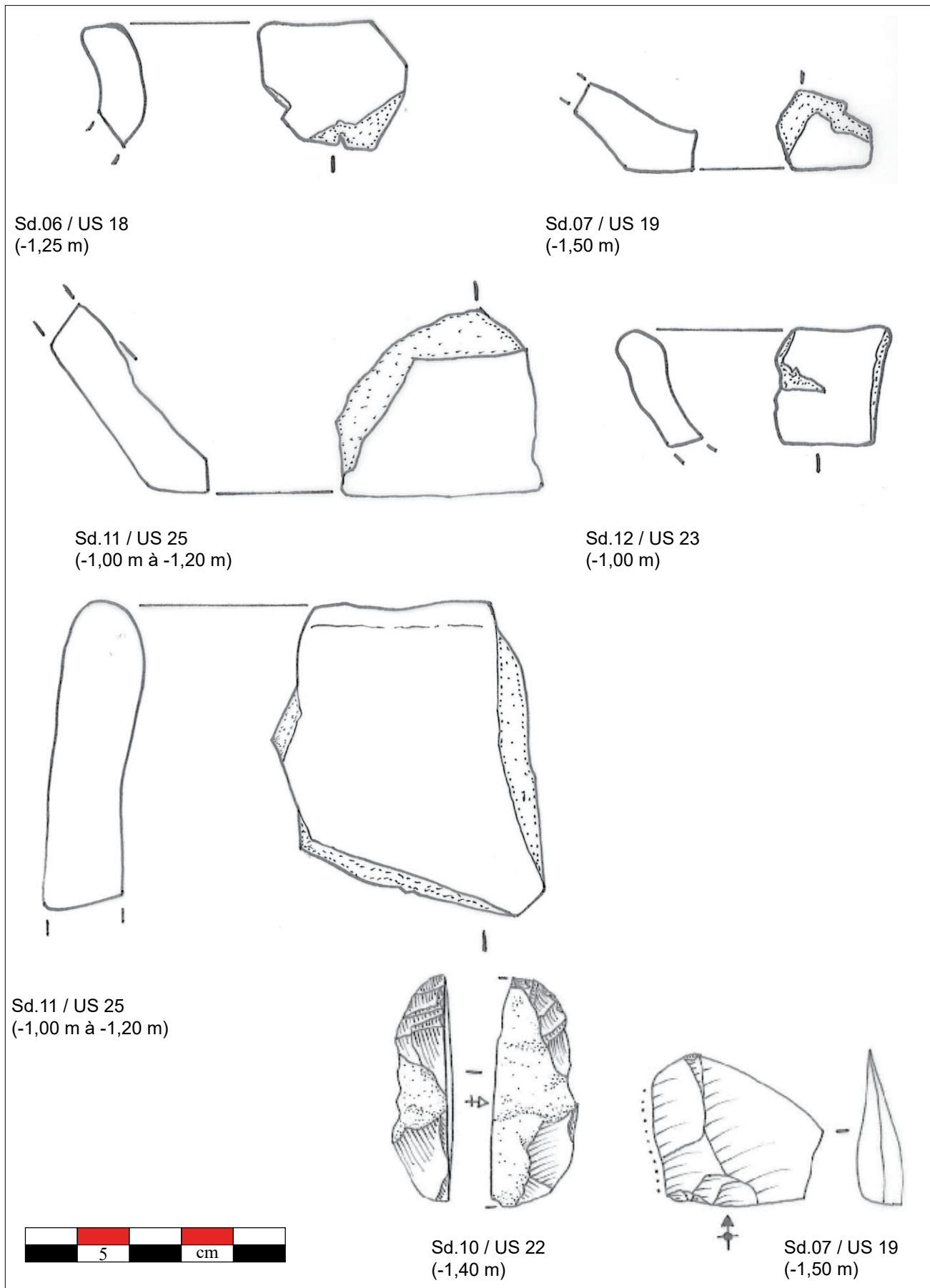
RENWEZ, Le Chemin des Écoliers, phase 2 Bords et fonds du mobilier céramique (dessin : S. BINDER), et outillage en silex (dessin : M. ETCHART-SALAS)
