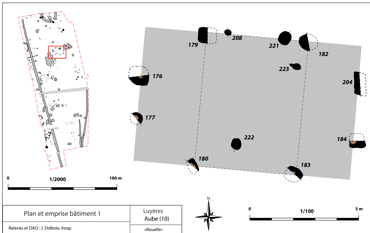
LUYÈRES, Rouelle Localisation et plan du Bâtiment 1, La Tène D1 (DAO : J. DOLBOIS)
