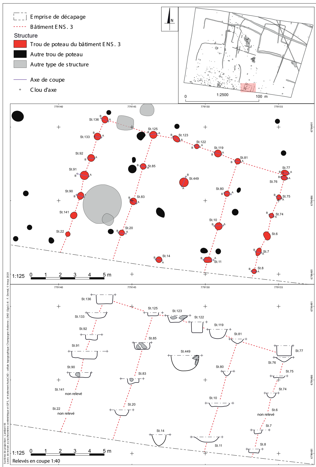
ROSIÈRES-PRÈS-TROYES, La Bouverie Plan du bâtiment du sud-est de l'emprise (DAO : F. DEMOL)
