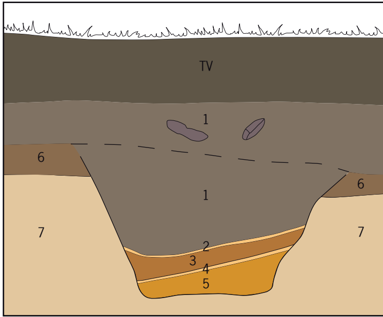
F. 202 Coupe NO/SE
