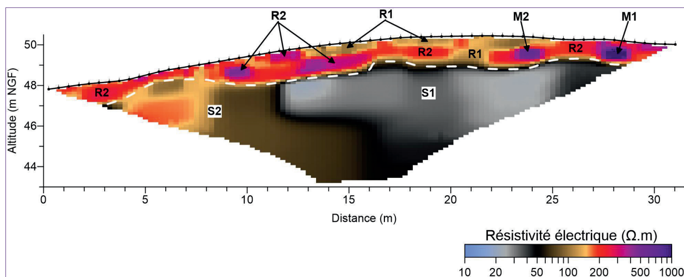
LOUDUN, Pé de Jojo, fig. 2 : section de résistivité électrique réalisée sur le monticule du Pé-de-Jojo (G. Bruniaux).
