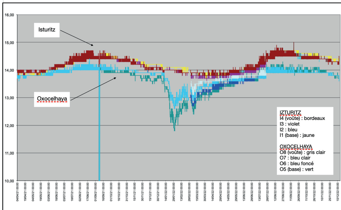
SAINT-MARTIN-D'ARBEROUE ET ISTURITZ, Les grottes d'Isturitz, d'Oxocelhaya et du Figuier - Suivi des températures dans les grottes d'Isturitz (courbes hautes) et d'Oxocelhaya (courbes basses), avril 2021- décembre 2022 (L. Magne et N. Vanara).
