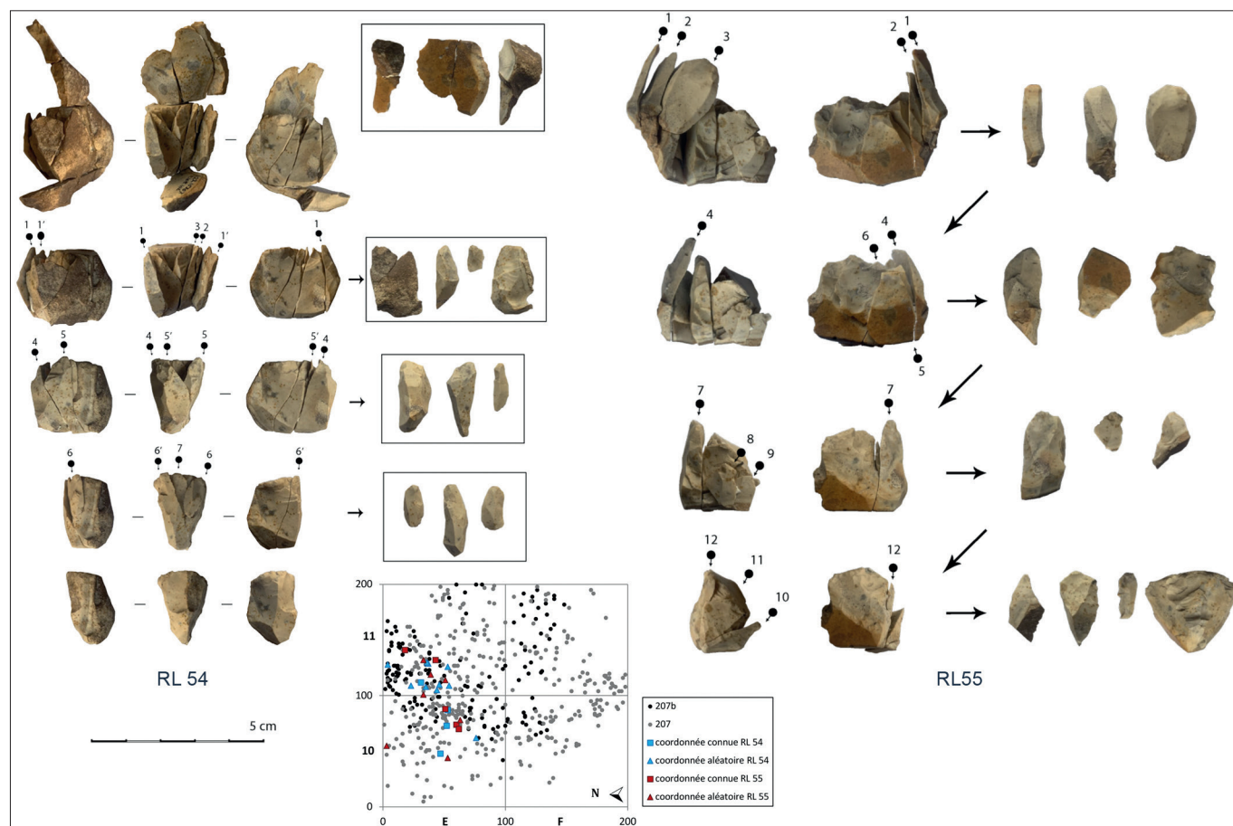
SAINTE-COLOME, Grotte Tastet - Remontage de deux séquences de production lamellaire (RL) et projection des pièces en plan (US 207-207b ; remontages, clichés et traitement M. Grubert).
