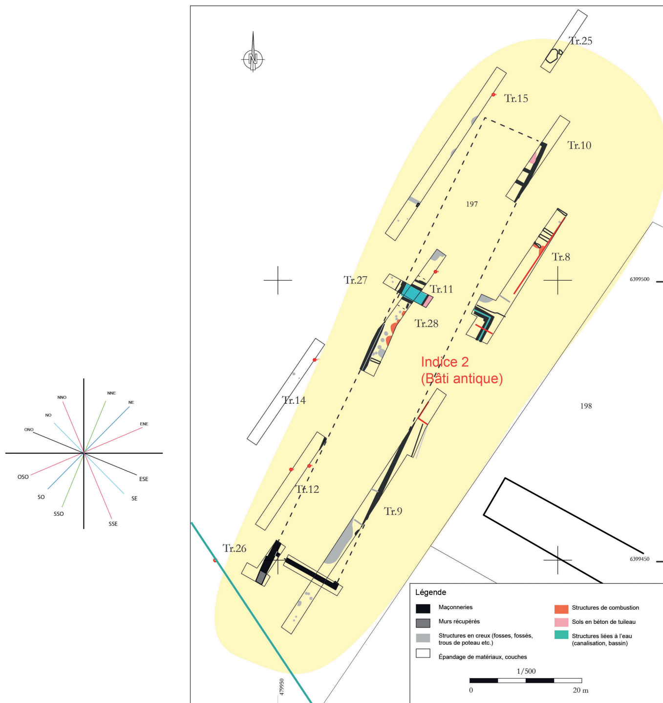
DURAS, Le Petit Sainte-Foy - Plan général de l'indice antique. Ech. : 1/500. © Bernard et C. Etrich, Inrap.
