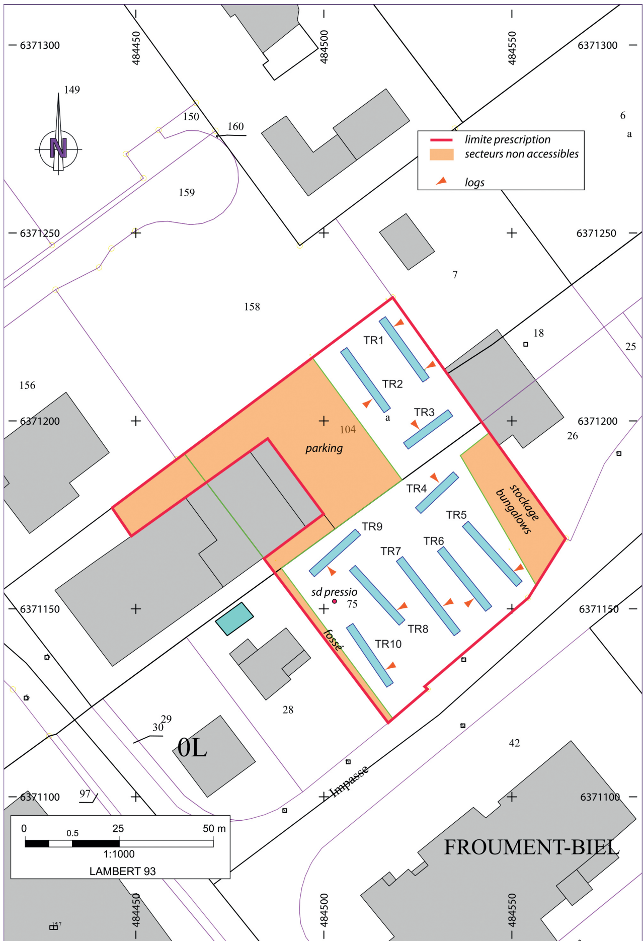
TONNEINS, 12 Rue de Suriray - Plan de répartition des sondages et des structures © S. Boulogne et P. Fouéré Inrap.
