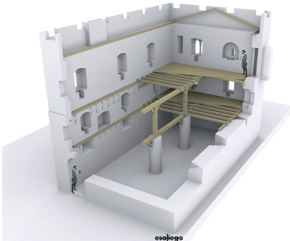
HONTANX, Château de Hontanx - Dessin d'évocation de l'état primitif.
