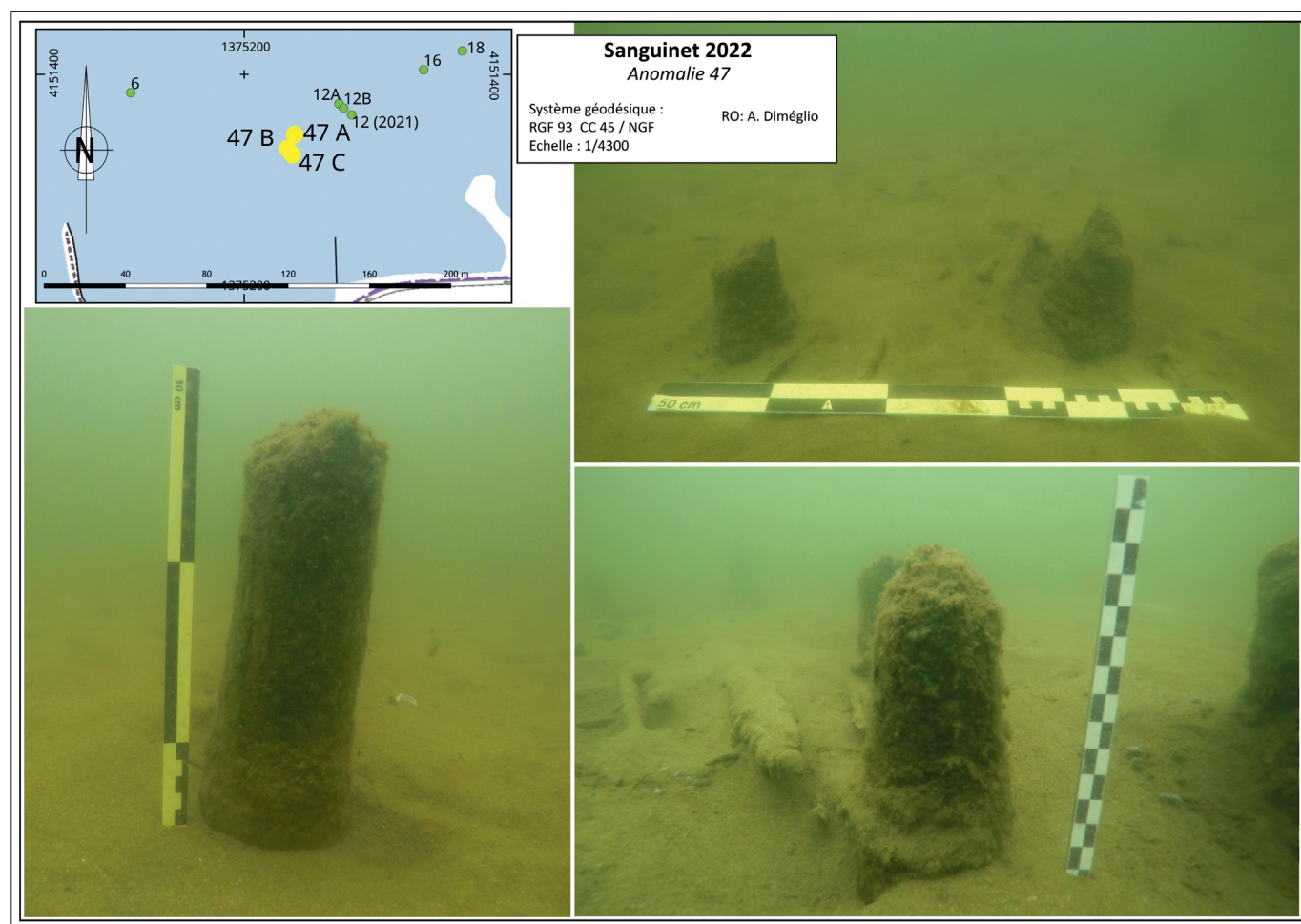
SANGUINET, Le Lac - Anomalie 47 - localisation - image sonar - photos in situ (DAO : A. Diméglio © Éveha, 2022. Source : IGN / QGIS. Reefmaster. Photo : C. Fretaud © Éveha, 2022).
