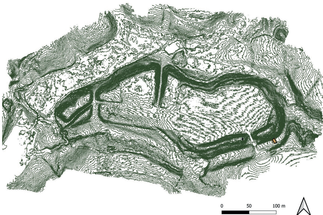
SAINT-JUSTIN, Arouille - Bialé - Plan général du site de Bialé en courbes de niveau, généré à partir du levé LiDAR. DAO Ch. Viaut.
