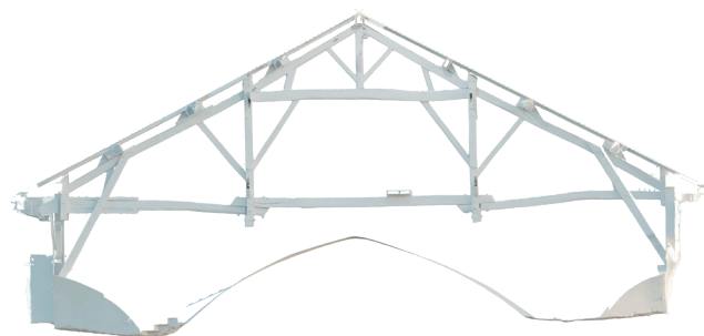
Bordeaux, Cathédrale Saint-André - Coupe de la ferme n° 5 de la charpente de la nef de la cathédrale, Evéha 2022.
