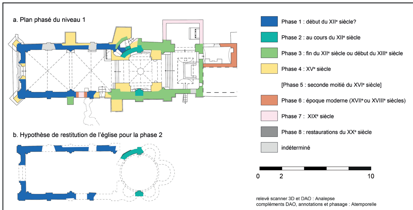
MONTILS, église Saint-Sulpice, fig. 1 : Plan phasé de l'église et restitution du plan en rotonde (DAO : E. Marot, fond de plan : Analepse)
