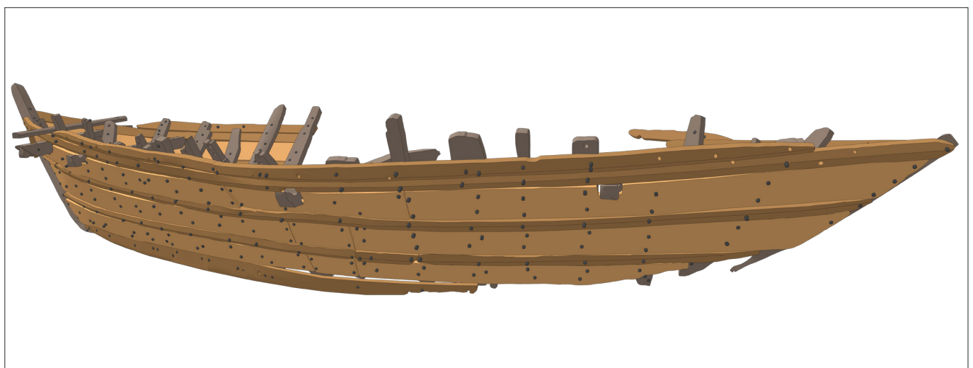
PORT-D'ENVAUX, le Priouté, fig. 2 : restitution 3D d'EP3 du Priouté a l'issu de sa fouille (DAO : P. Moyat).
