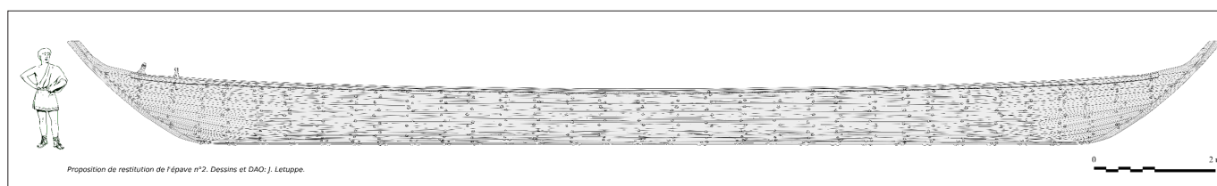
SAINTES ET FONTCOUVERTE, Courbiac, proposition de restitution de l'épave n°2 de Courbiac (Dessin et DAO : J. Letuppe)
