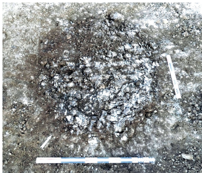
CHÂTELAILLON-PLAGE, rue du Canal, fig. 1 a et b : Vue en plan et en coupe de la structure 4.21 (relevé et clichés : V. Audé ; DAO : M. Coutureau)
