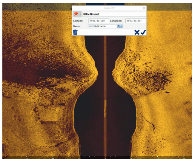
SAINT-VAIZE, fig.2 seuil
