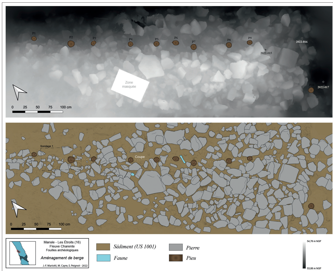
MANSLE, Les Étroits, plan de l'aménagement de berge (DAO : J.-F. Mariotti, M. Cayre, S. Peignot)
