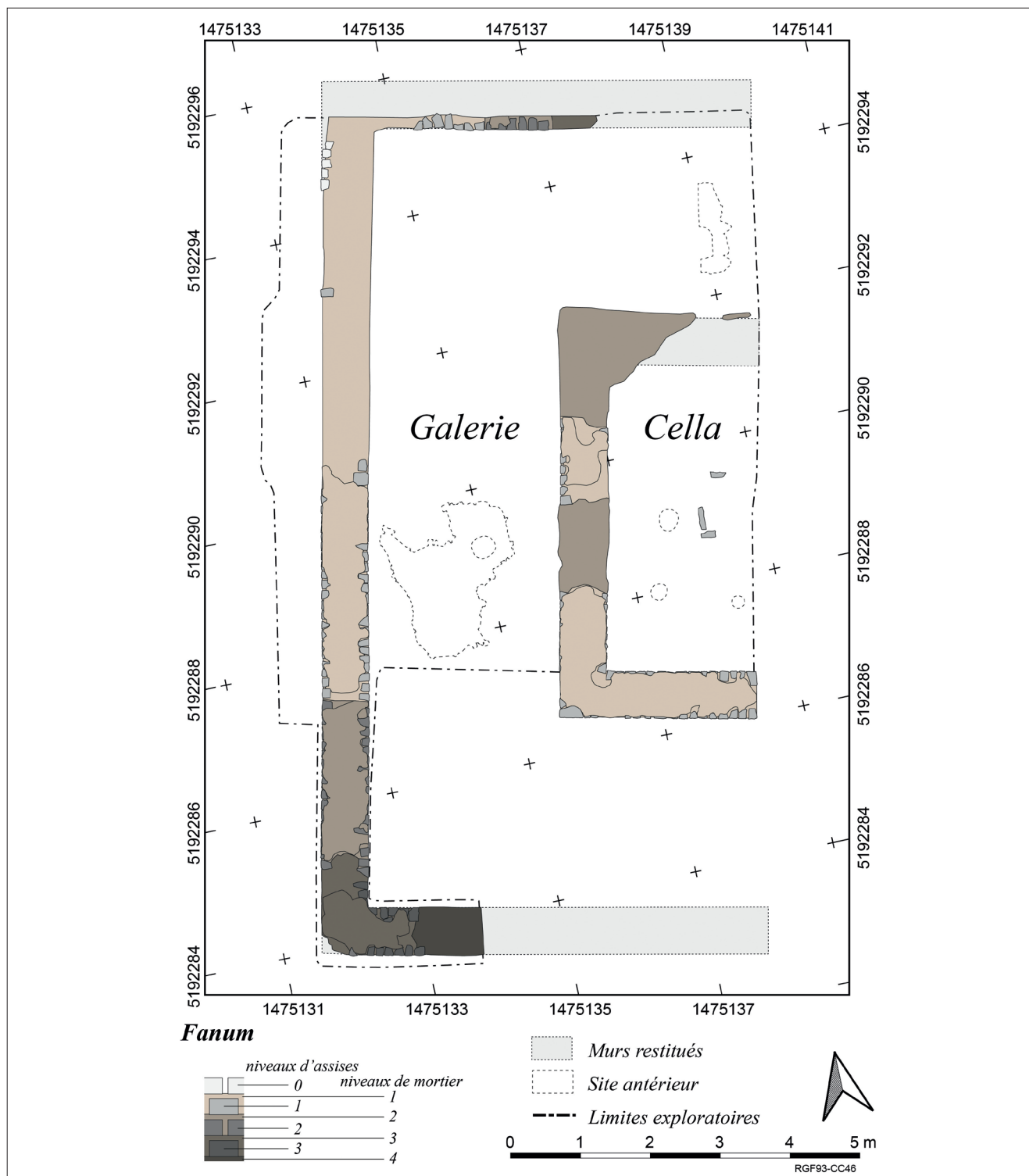
LUXÉ, La Terne, plan des structures du sanctuaire maçonné. (DAO : S. Peignot)
