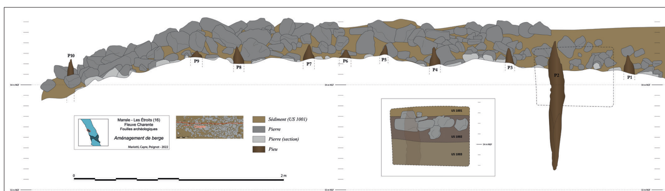
MANSLE, Les Étroits, Coupe projetée de l'aménagement de berge. (J.-F. Mariotti, M. Cayre, S. Peignot)
