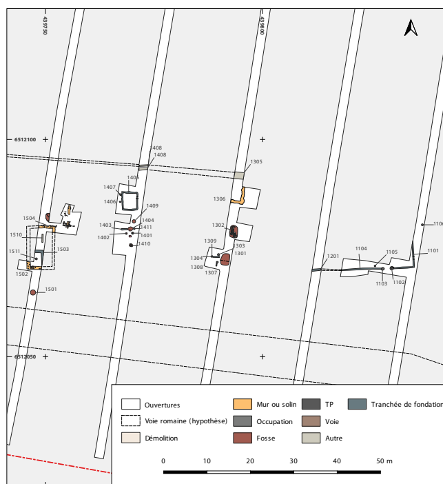
CHATEAUBERNARD, dix-huit-un, plan du secteur sud-est (DAO : P. Maguer)
