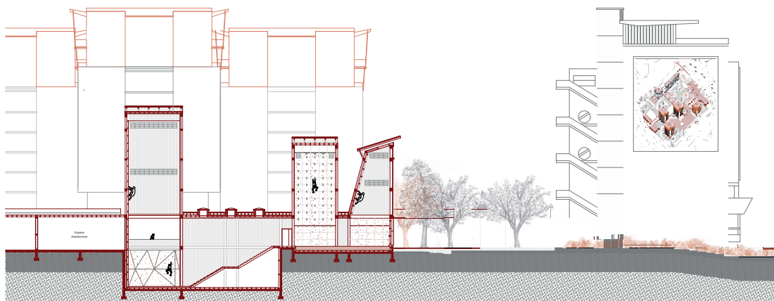
Coupe longitudinale dans la salle d'escalade - 100mm
