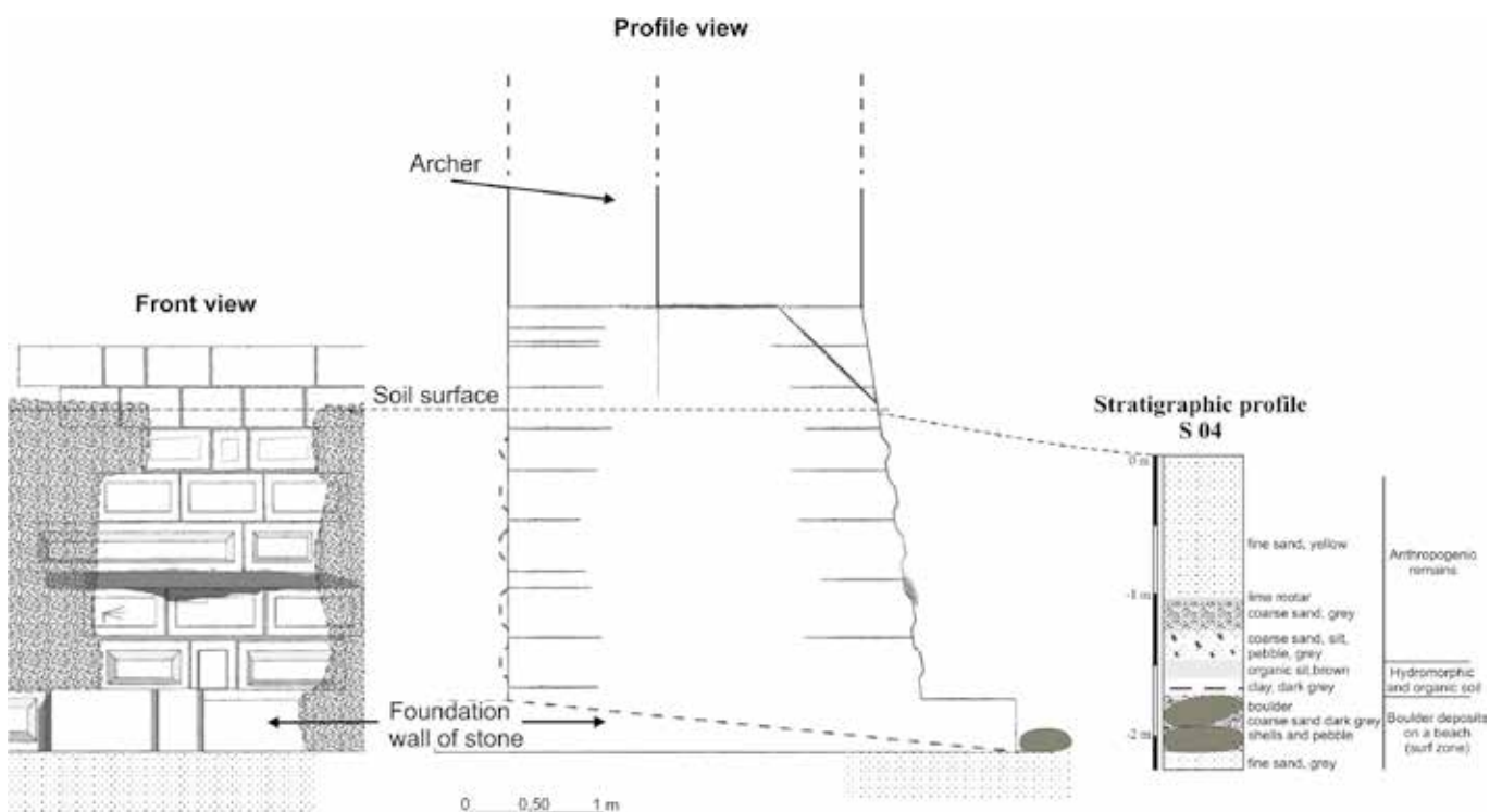
Fig. 1 : rempart sud d'Aigues-Mortes. Vue de face et de profil entre la Porte de l'Arse-
