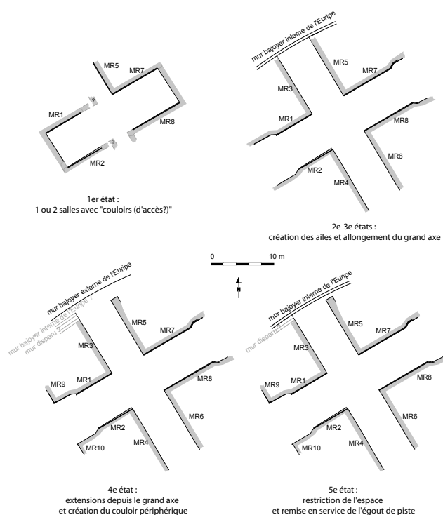
Fig. 2 : plans phasés.
