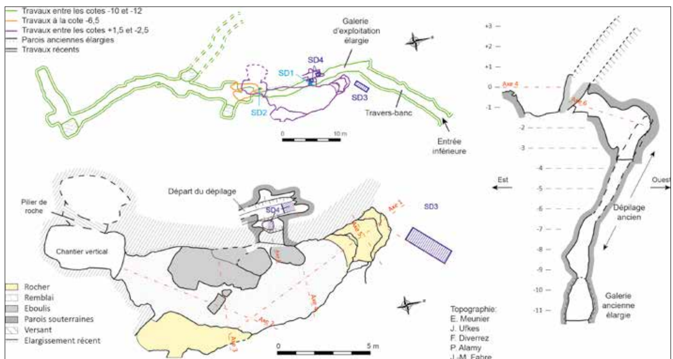
Plan des travaux et coupe du défilé incliné.
