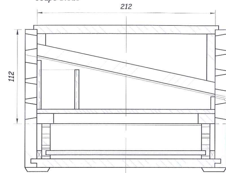
Coupe bleue
