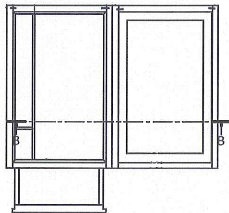
B-B (1 : 4)
