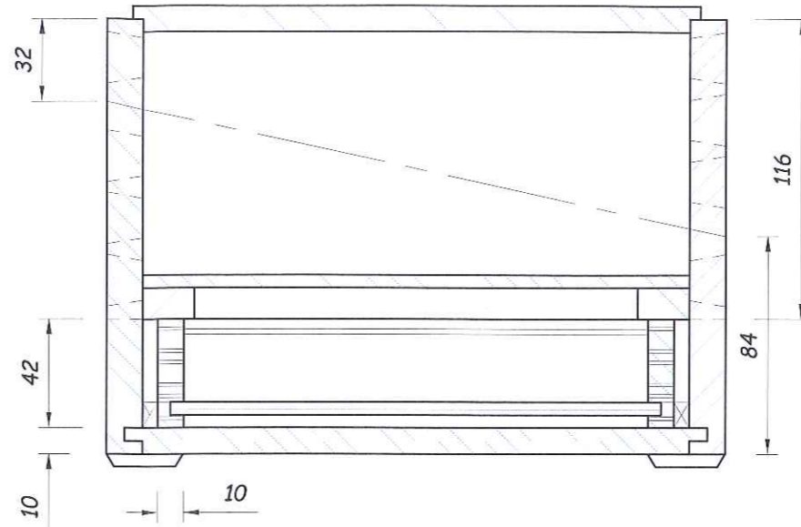
Coupe bleue avant la coupe à la scie circulaire
