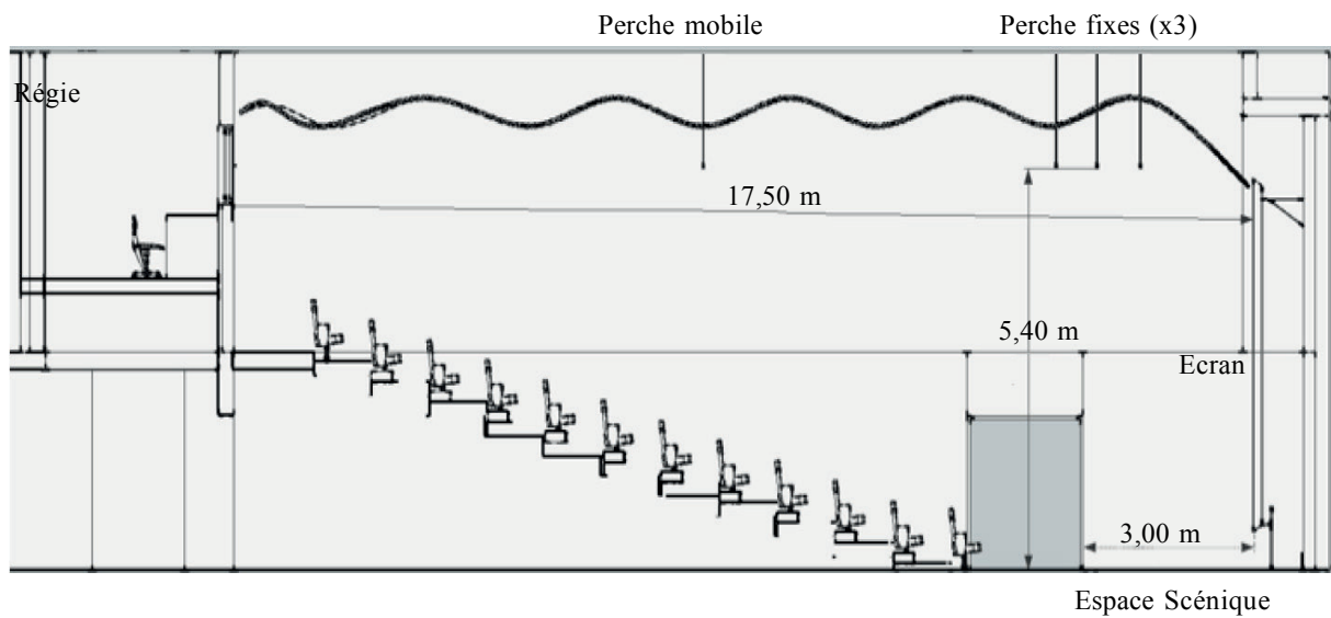
Plan 1.2 : Dimensions de l'Auditorium. Vue de côté.
