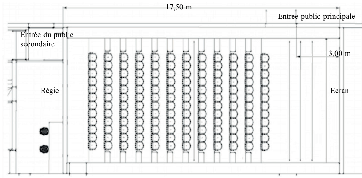
Plan 1.1 : Dimensions de l'auditorium. Vue de dessus.
