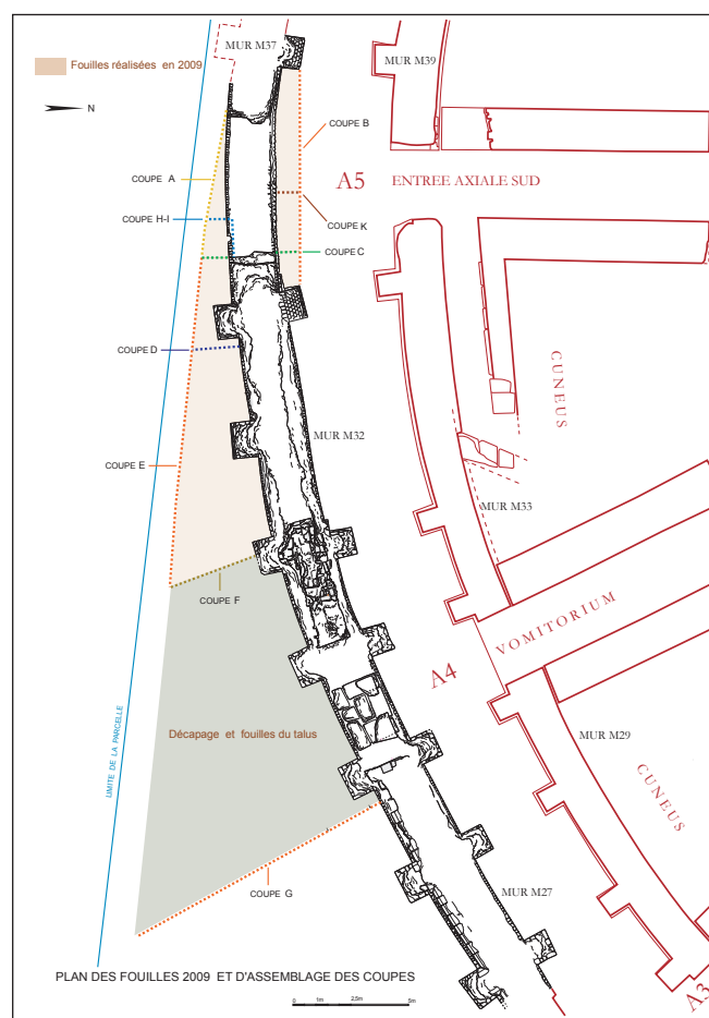
Lillebonne, Théâtre romain, fig. 1 : plan de la zone sud-est (V. Mutarelli)
