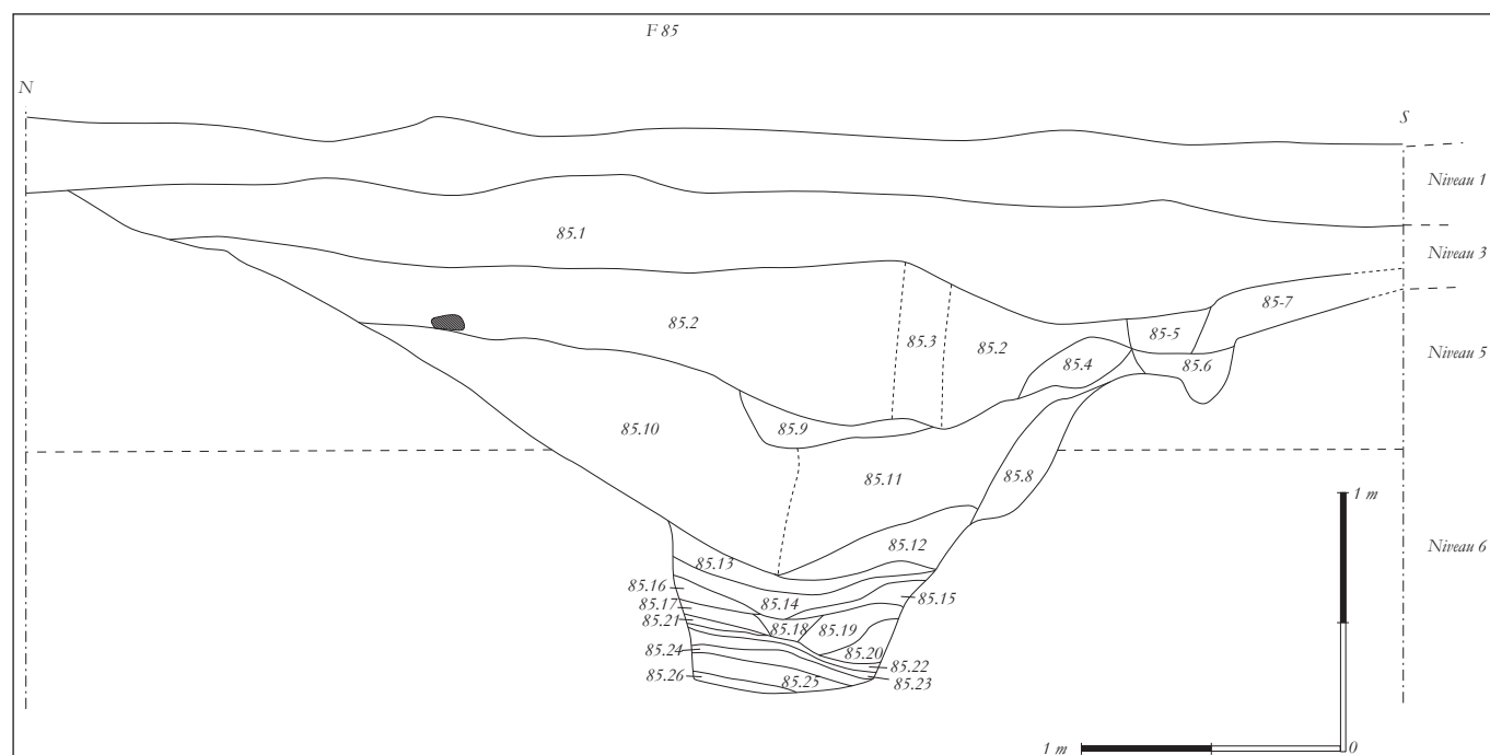
Le Tréport, Entre les deux Chemins : profil du fossé d'enclos circulaire (relevé : L. Feret, D. Lukas ; DAO : V. Théron.)
