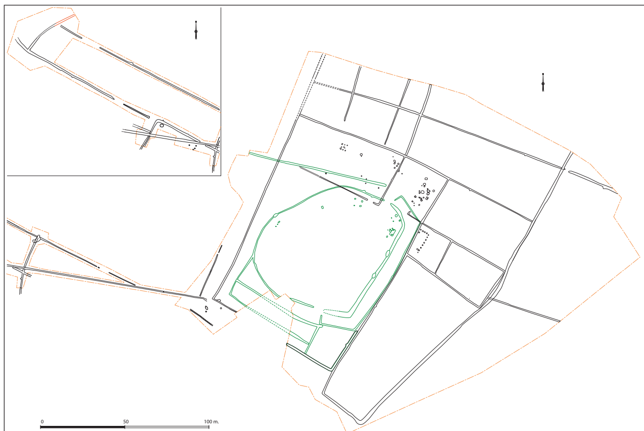
Isneauville / Saint-Martin-du-Vivier, Plaine de la Ronce : plan général des vestiges gaulois (zone A) (S. Le Maho, Y.-M. Adrian)
