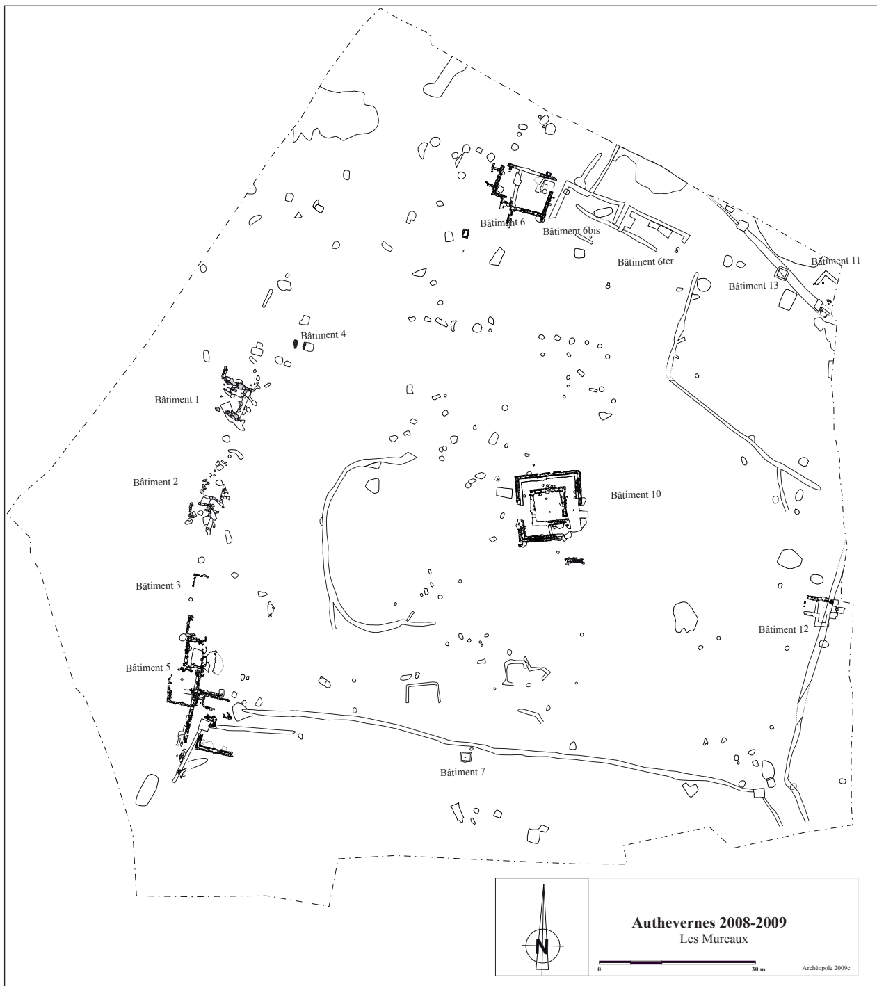
Authevernes, Les Mureaux : plan général des vestiges (J. Boisson et M. Michel)
