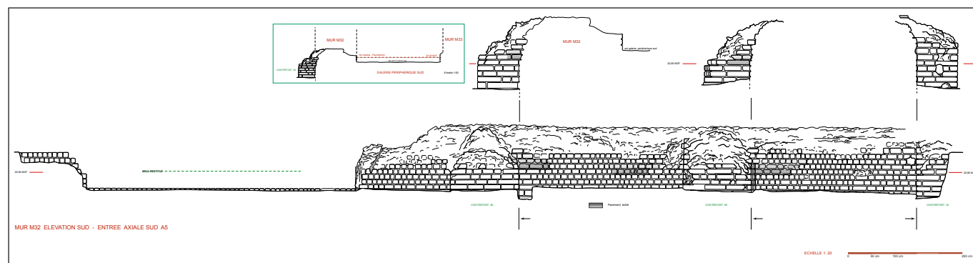
Lillebonne, Théâtre romain, fig. 4 : relevé de l'élévation de la façade du mur M32 et de l'entrée axiale sud (V. Mutarelli)
