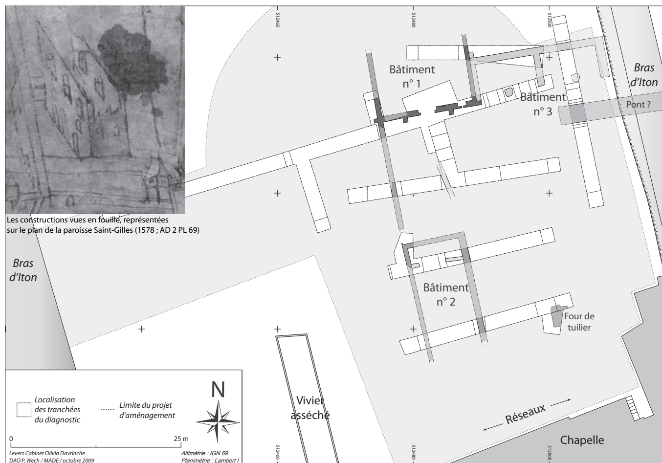
Évreux, 7 rue Joséphine : plan des principaux éléments bâtis médiévaux mis au jour lors du diagnostic (P. Wech)
