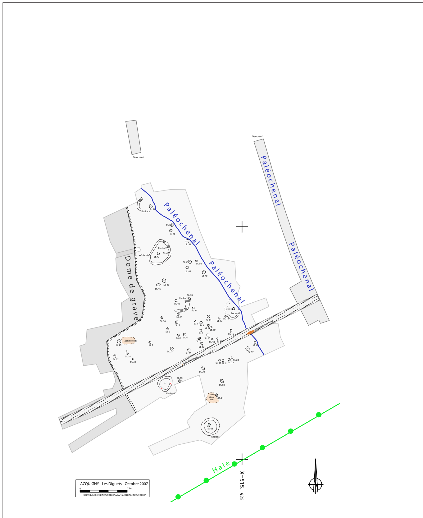
Acquigny, Les Diguets : plan général de la zone protohistorique (E. Leclercq, C. Rapine)
