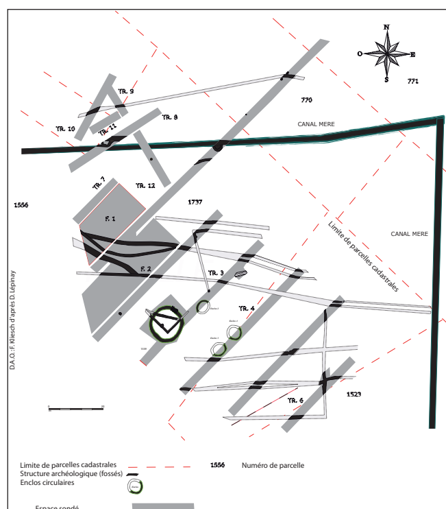
Nonancourt, La Potinière : plan de l'occupation protohistorique (F. Kliesch)
