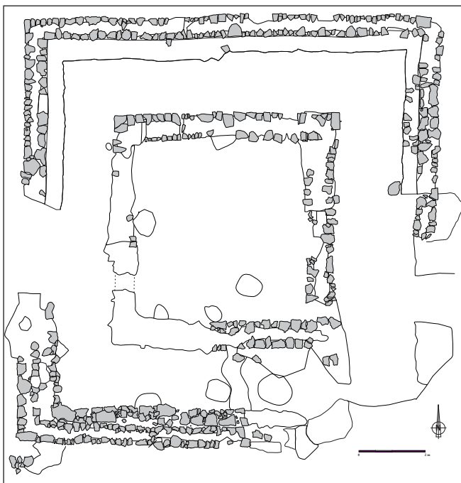
Authesvernes, Les Mureaux : plan du fanum (J. Boisson et M. Michel)
