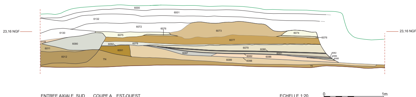
Lillebonne, Théâtre romain, fig. 2 : entrée axiale sud. Coupe avec les séquences de voies (V. Mutarelli)
