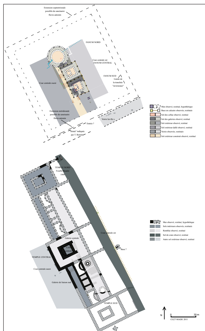
Le Vieil-Évreux, Le Grand Sanctuaire : plan du monument claudio-antonin et du monument sévérien (MADE)
