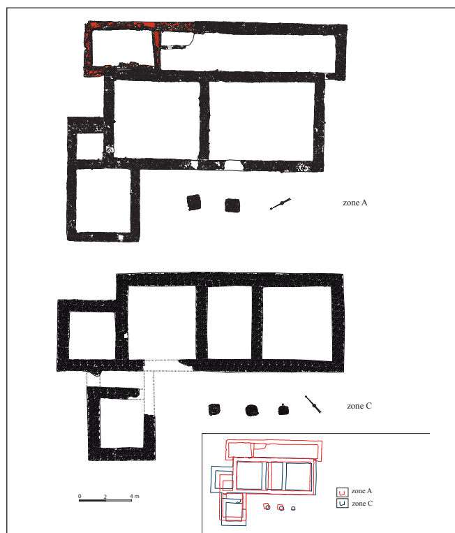
Isneauville / Saint-Martin-du-Vivier, Plaine de la Ronce : comparatif des deux bâtiments résidentiels fouillés sur les zones A et C. (S. Le Maho, Y.-M. Adrian)
