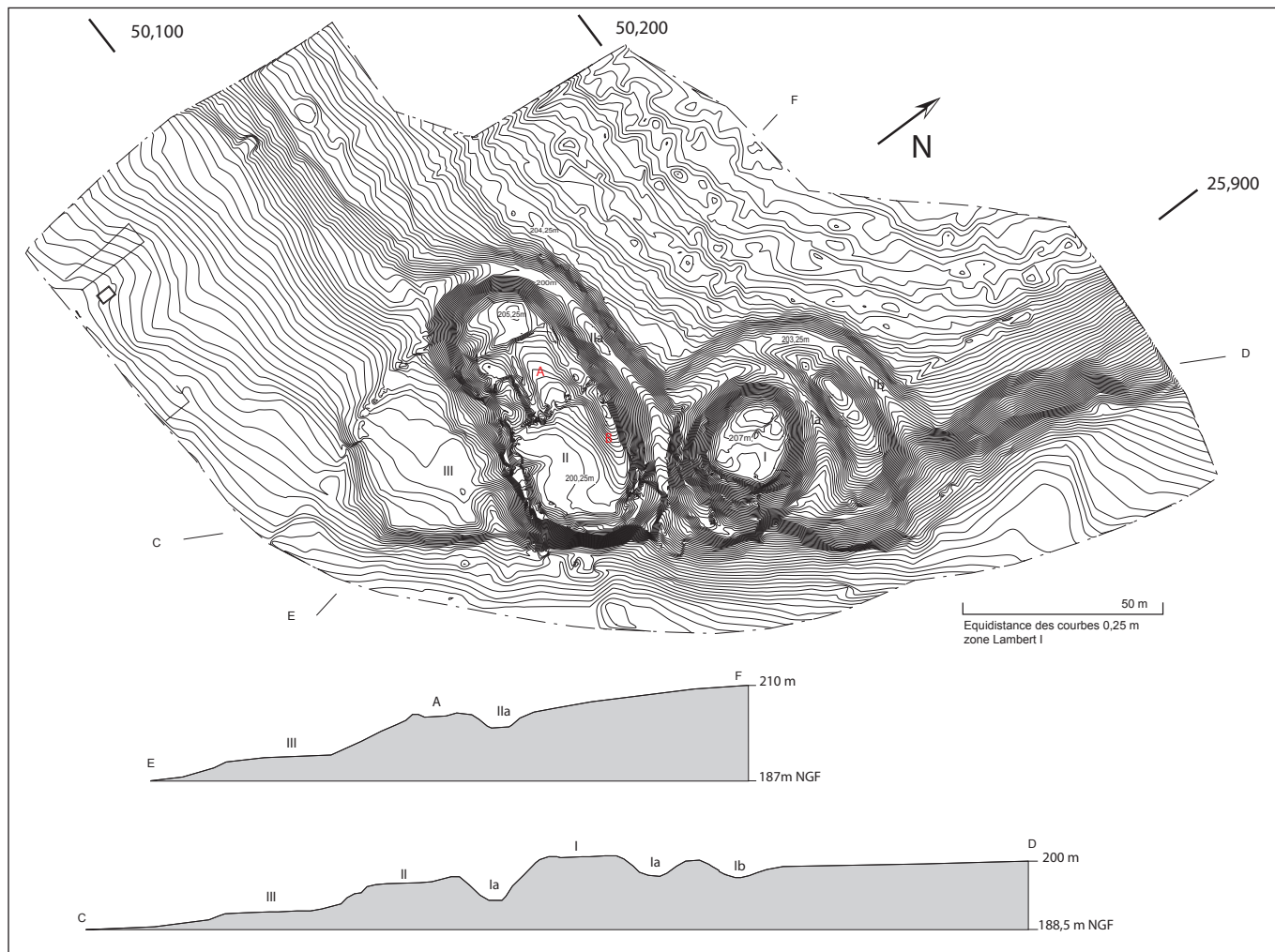
Notre-Dame-du-Hamel (27), Échanfray : plan topographique et coupe (relevé : T. Debaene, F. Épaud, D. Étienne, T. Guérin, J. Le Maho, B. Lepeuple, A. Painchault ; mise au net : A. Painchault)
