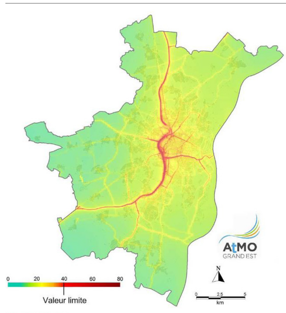
CARTE N°6 PLU : Concentration moyenne annuelle de NO2 en 2016
