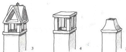
1. Assemblage tuiles et briques 2. Assemblage en simples tuiles 3. Mitre 4. Assemblage à dalette 5. Chapeau en pyramide tronquée.
