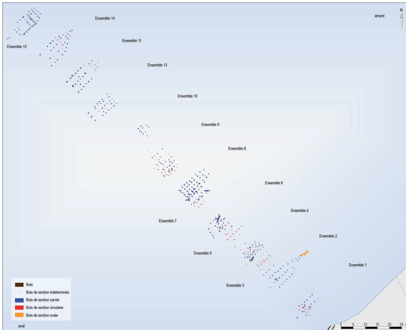
Fig. 1 : Blois (Loir-et-Cher) PCR ville et territoire : plan des vestiges des franchissements de La Tène finale ou changement de notre ère, et de la deuxième moitié du II e s., section des bois. (Viviane Aubourg, DRAC CVL)
