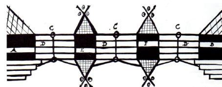
Plan du pont de la Clapière d'Embrun
