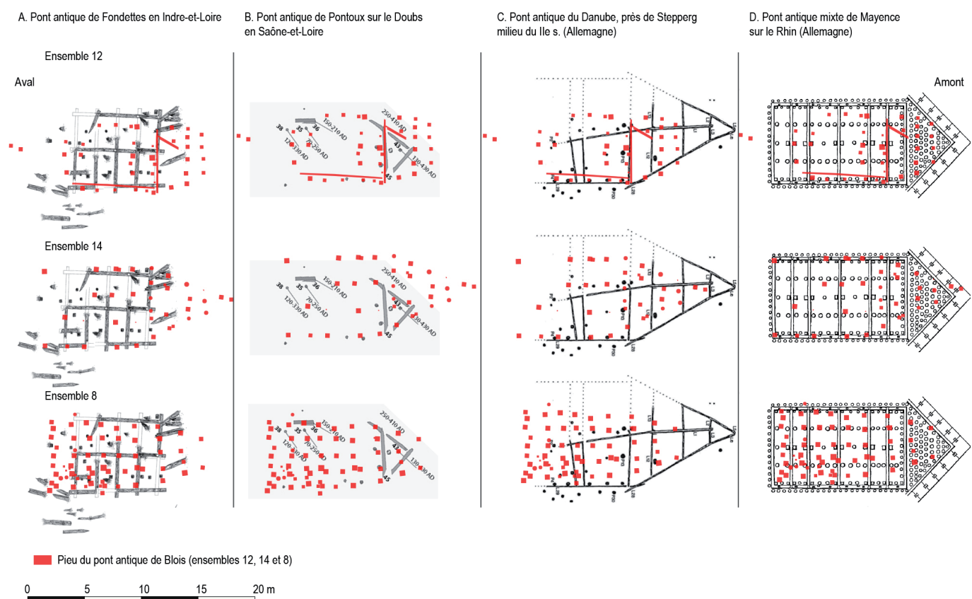
Fig. 2 : Blois (Loir-et-Cher) PCR ville et territoire : superposition des plans de trois piles du pont antique de Blois sur des plans de vestiges d'ouvrages de même période étudiés en France et en Allemagne. (Viviane Aubourg, DRAC CVL)
