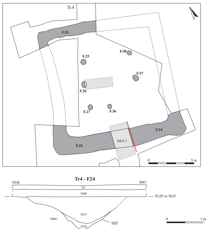
Fig. 2 : Cheverny (Loir-et-Cher) RD 765 – RD 102 : plan de l'enclos quadrangulaire Ile-ler av.-J.-C. et relevé stratigraphique de son tronçon sud. (Véronique Chollet, Inrap)
