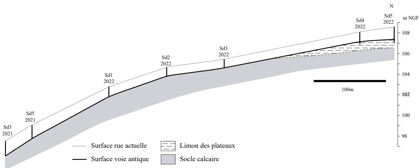
Blois (Loir-et-Cher) rue du Bourg-Neuf : coupe schématique de la rue du Bourg-Neuf. (Philippe Gardère, Inrap)
