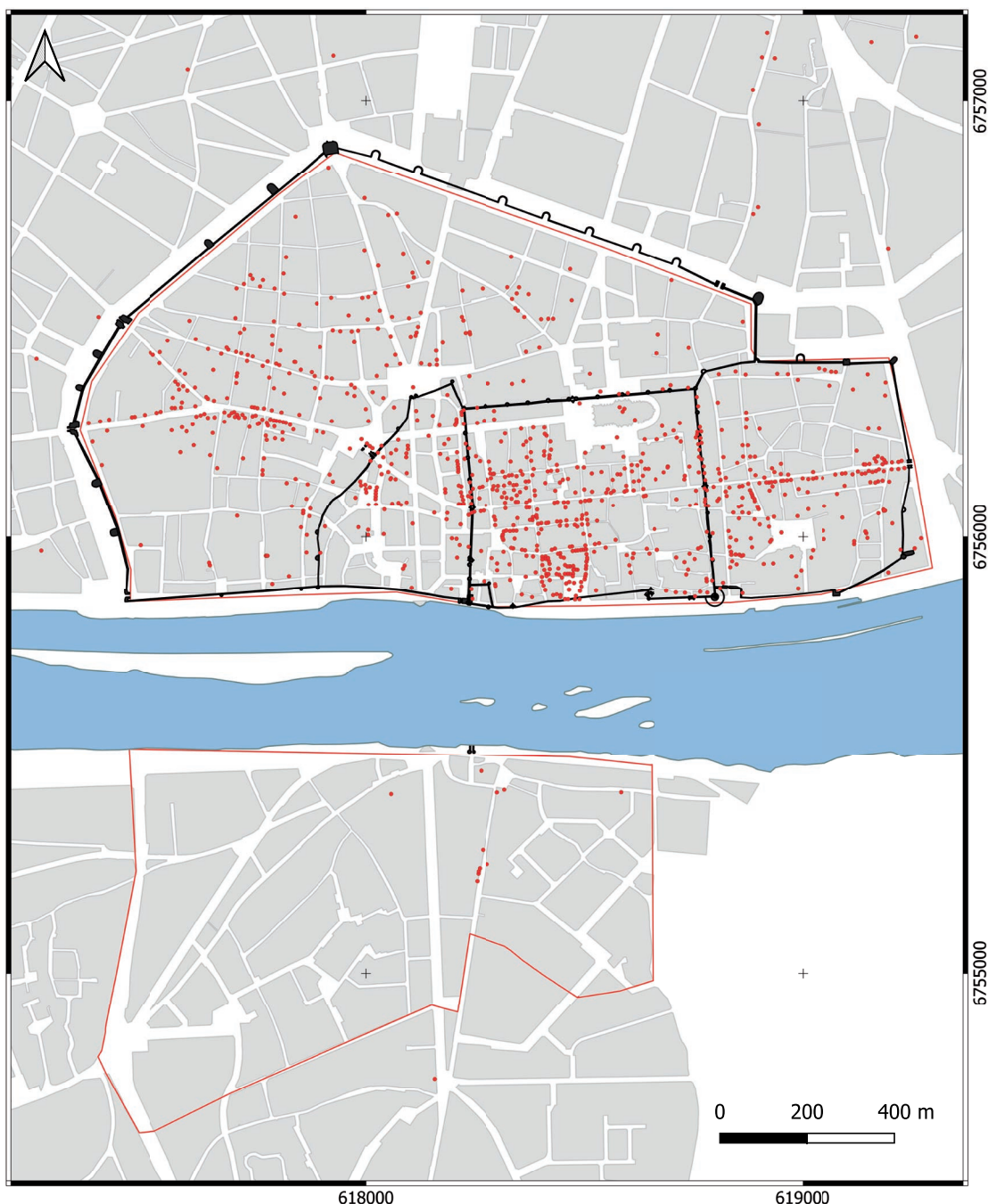
Fig. 1 : Orléans (Loiret) caves du centre-ville : extrait du SIG, état de la prospection des cavités dans « l'intra-muros » (« intra-mails ») et au sud de la Loire. (Daniel Morleghem)
