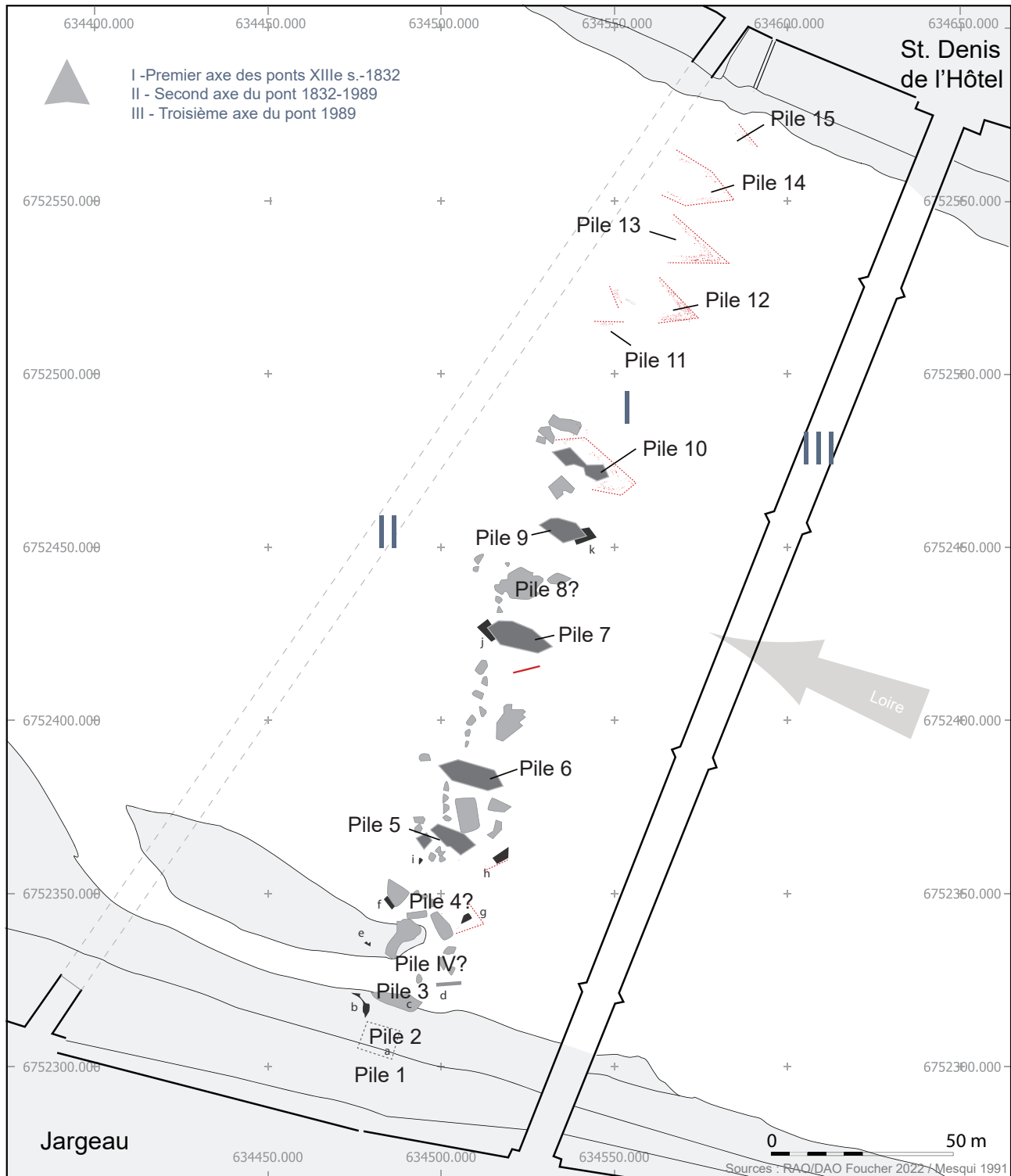
Pont de Jargeau d'après les campagnes de 1987 (gris) et 2022 (rouge). Les piles identifiées par J. Mesqui apparaissent en gris foncé, les massifs maçonnés issus d'effondrements en gris clair. (d'après Mesqui 1991, Marion Foucher, Université de Bourgogne)
