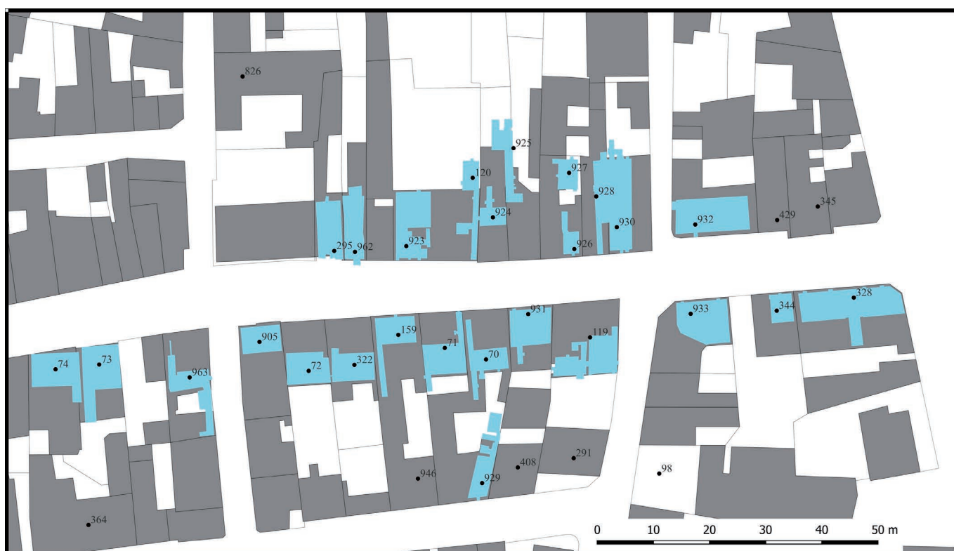
Fig. 3 : Orléans (Loiret) caves du centre-ville : extrait du SIG, plans des cavités relevées en 2022 à l'extrémité orientale de la rue de Bourgogne. (Clément Alix, Daniel Morleghe, Pôle d'archéologie de la ville d'Orléans)
