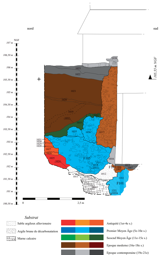
Fig. 4 : Orléans (Loiret) 4 rue Coligny : coupe de l'extrémité orientale de la tranchée de démolition avec vestiges des fondations de l'édifice du premier Moyen Âge. (Clément Alix, Pôle d'Archéologie de la Ville d'Orléans)
