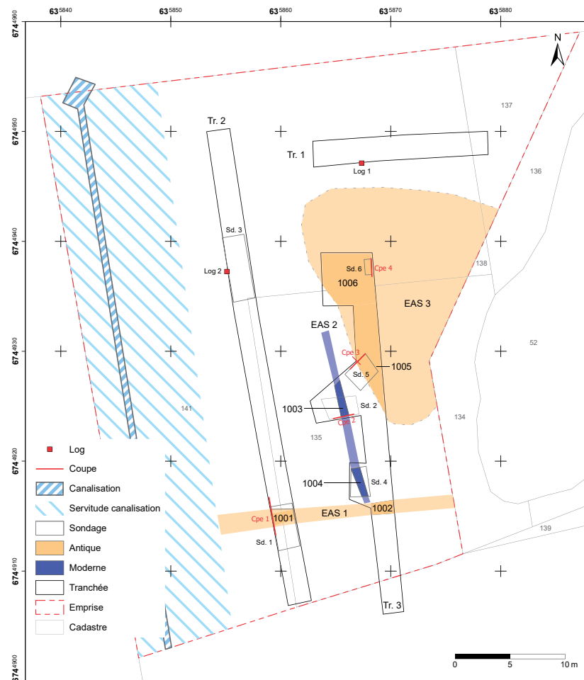
Vienne-en-Val (Loiret) la Monardière, le Chapeau-à-Trois-Cornes : plan synthétique de l'organisation des vestiges. (Karine Payet-Gay, Service d'archéologie préventive du Département du Loiret)
