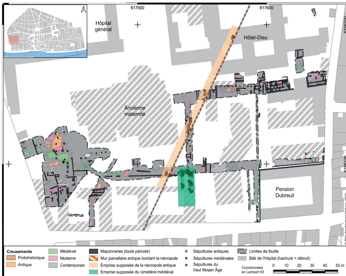
Orléans (Loiret) 1 rue Porte-Madeleine : plan général de la fouille réalisée en 2022. (Julien Courtois, Pôle d'archéologie de la ville d'Orléans)
