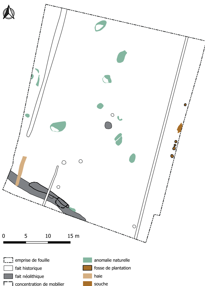
Mardié (Loiret) l'Aumône : plan général des vestiges. (Olivia Dupart, Inrap)
