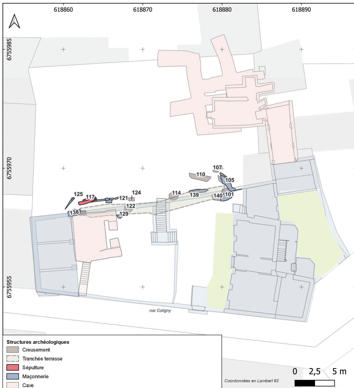
Fig. 1 : Orléans (Loiret) 4 rue Coligny : plan de la parcelle avec localisation de la tranchée de démolition du mur de terrasse et emprise des caves. (Clément Alix, Pôle d'Archéologie de la Ville d'Orléans)
