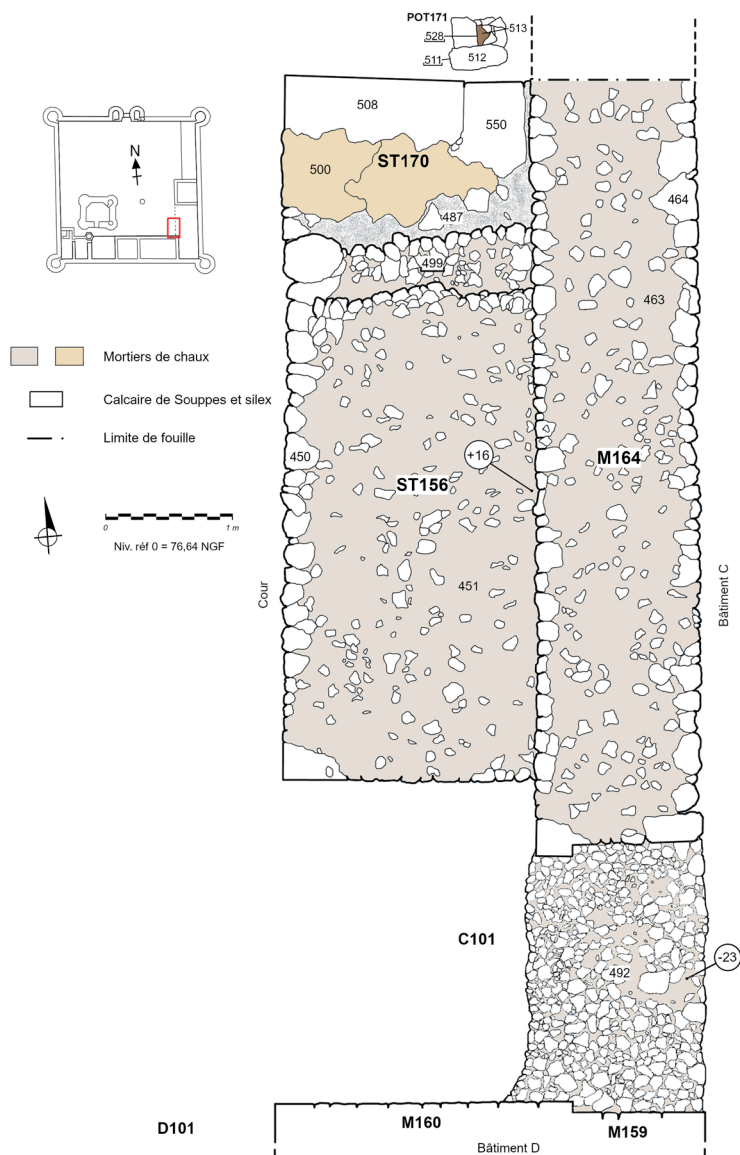
Fig. 2 Dordives (Loiret) château de Metz-le-Maréchal : relevé du mur de façade du bâtiment C et des fondations de l'escalier accolé. (Edwige Borel, ADM)
