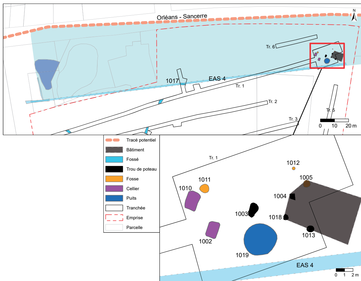
Vienne-en-Val (Loiret) la Monardière, route de Tigy : proposition d'interprétation de l'occupation antique. (Dany Souchet, Service d'archéologie préventive du Département du Loiret)
