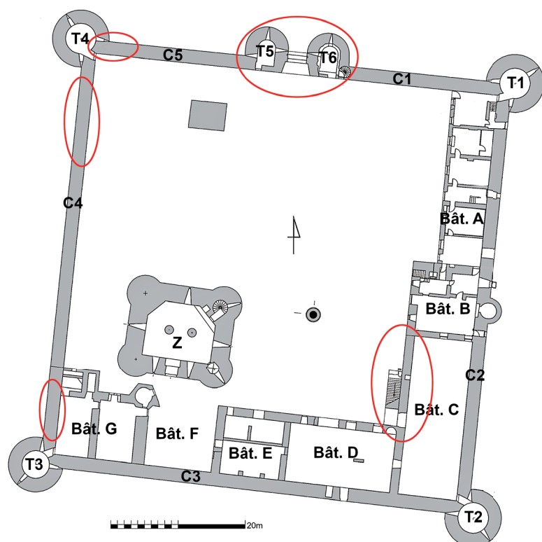
Fig. 1 Dordives (Loiret) château de Metz-le-Maréchal : plan général du château et localisation des zones d'études. (Michel Piechaczyk, ADM)
