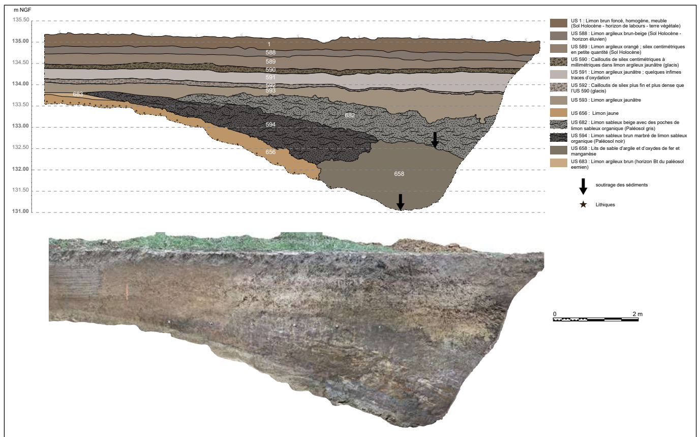
Guichainville, Le Long-Buisson 3 : relevé et photogrammétrie de la coupe ouest-sud-ouest du Log 41, SD 8, tranchée 70 (topographie : M. Osmond ; infographie : MADE).
