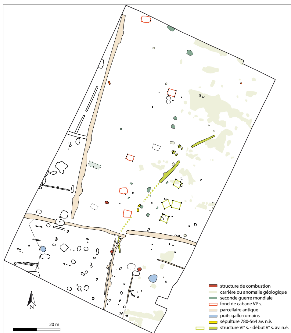
Frénouville, rue Fred Scamaroni, fig. 1 : plan général de la fouille (J.-M. Palluau).
