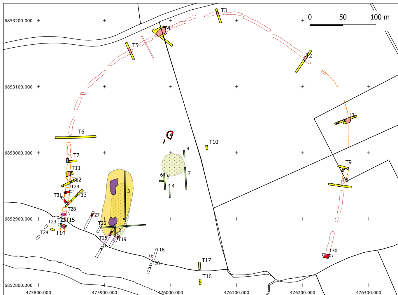
Moulins-sur-Orne, Argentan, Brûle-Piquet, Les Hogues, Le Grand Beaulieu : plan général issu des sondages et des prospections géophysiques (DAO C. Billard).
