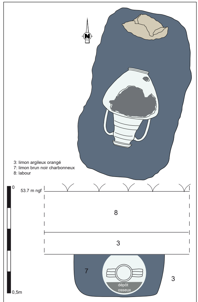
Biéville-Beuville, Aménagement Boulevard Urbain Nord : plan et coupe de l'incinération du Haut-Empire (DAO E. Ghesquière).
