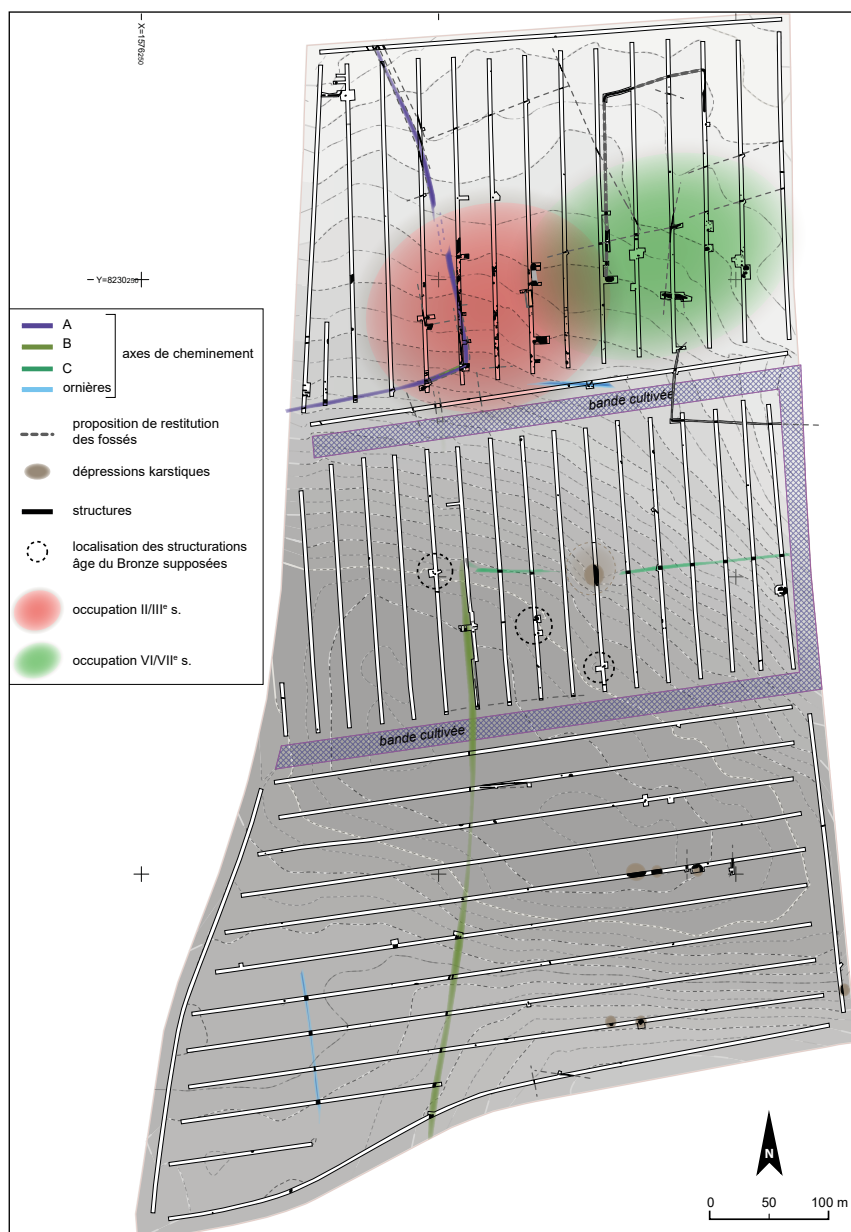
Daubeuf-près-Vatteville, Les Champs de Senneville : plan des résultats et propositions de restitution des tracés (topo : M. Osmond, DAO : N. Gautier).
