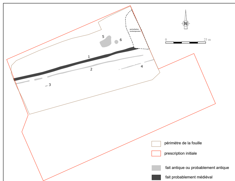
Saint-Pierre-de-Varengeville, chemin de la Messe : plan des vestiges (S. Calduch / Y.-M. Adrian).
