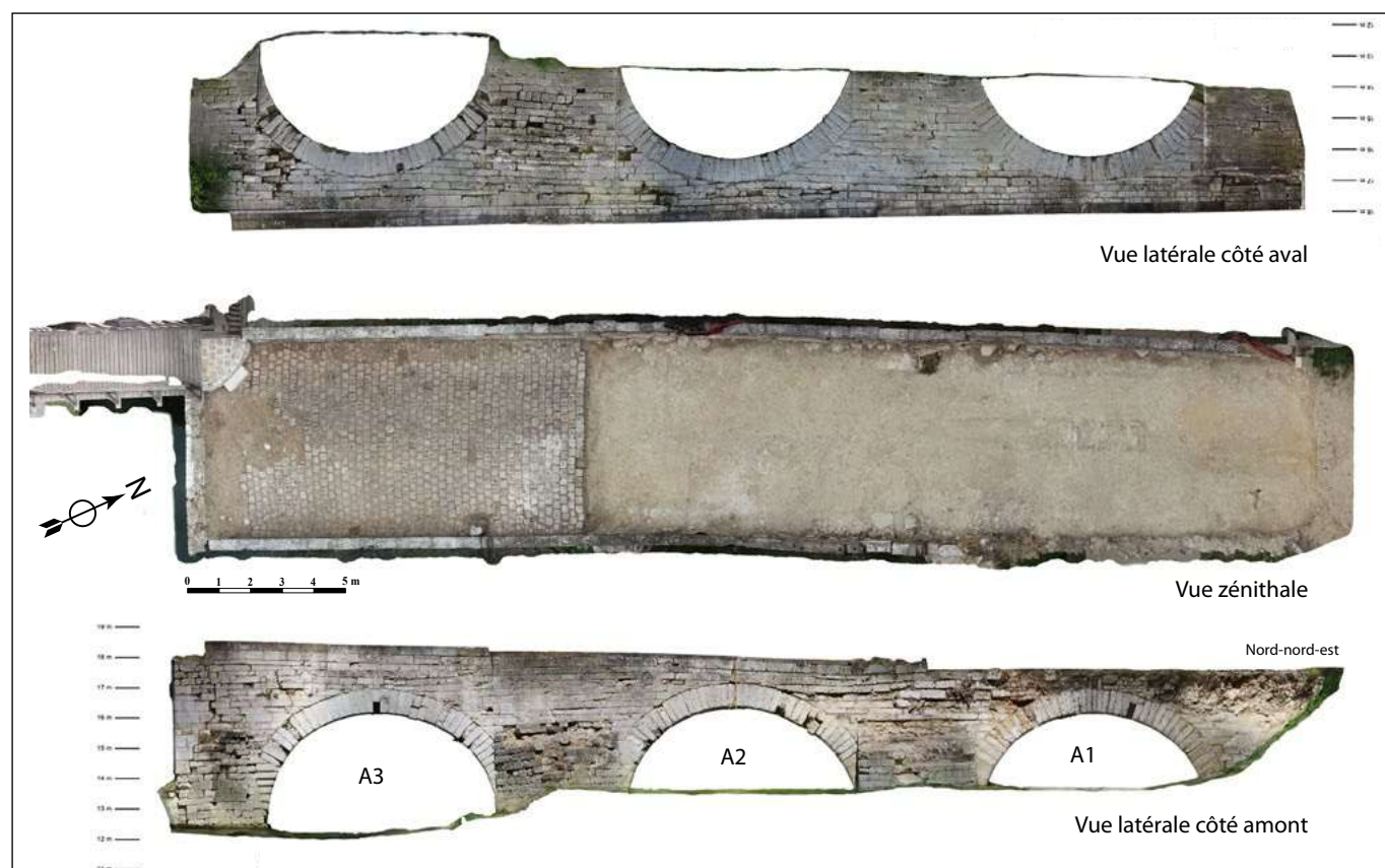
VERNON, Vieux pont : orthophotographies des trois arches A1, A2 et A3 - vue zénithale, faces aval et amont (orthophotographies : N. Wasylyszyn, DAO : P. Fajon).
