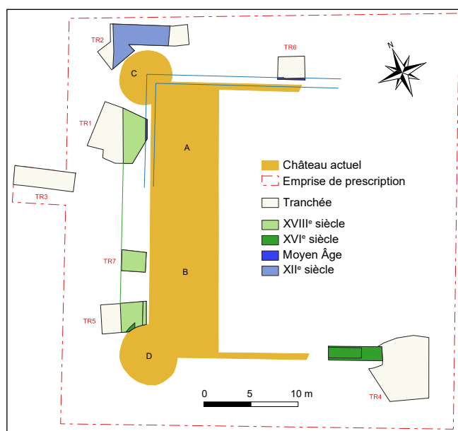
Les Monts-du-Roumois, château d'Houlbec-près le Gros Theil, fig. 2 : plan phasé des structures du diagnostic (B. Guillot).
