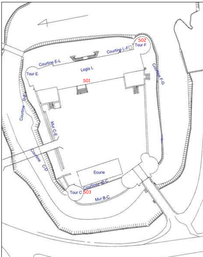
Saint-Martin-du-Bec, château du Bec-Crespin : plan du château, localisation des sondages (J.-F. Legembre).
