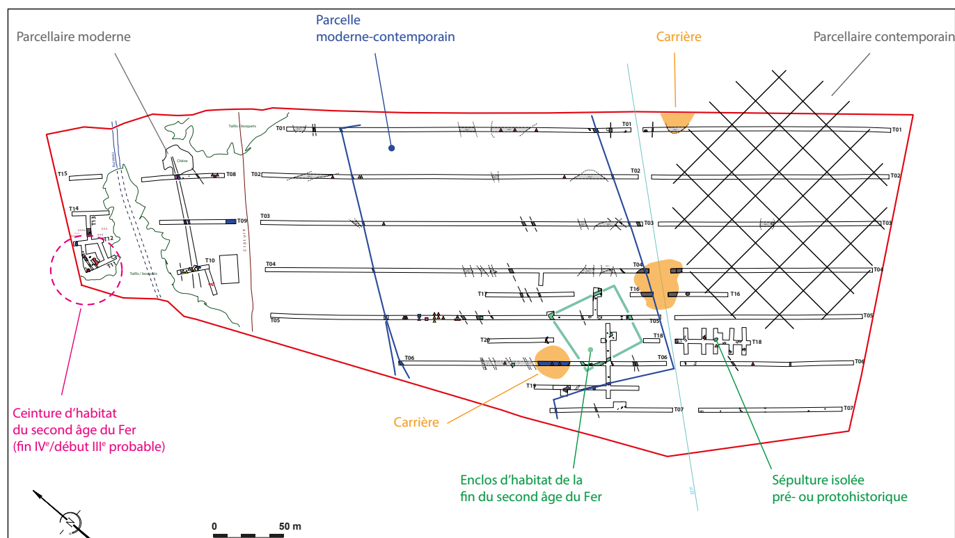
Nécý, La Martinière : organisation des sondages et des vestiges dans l'emprise du projet (I. Jahier).
