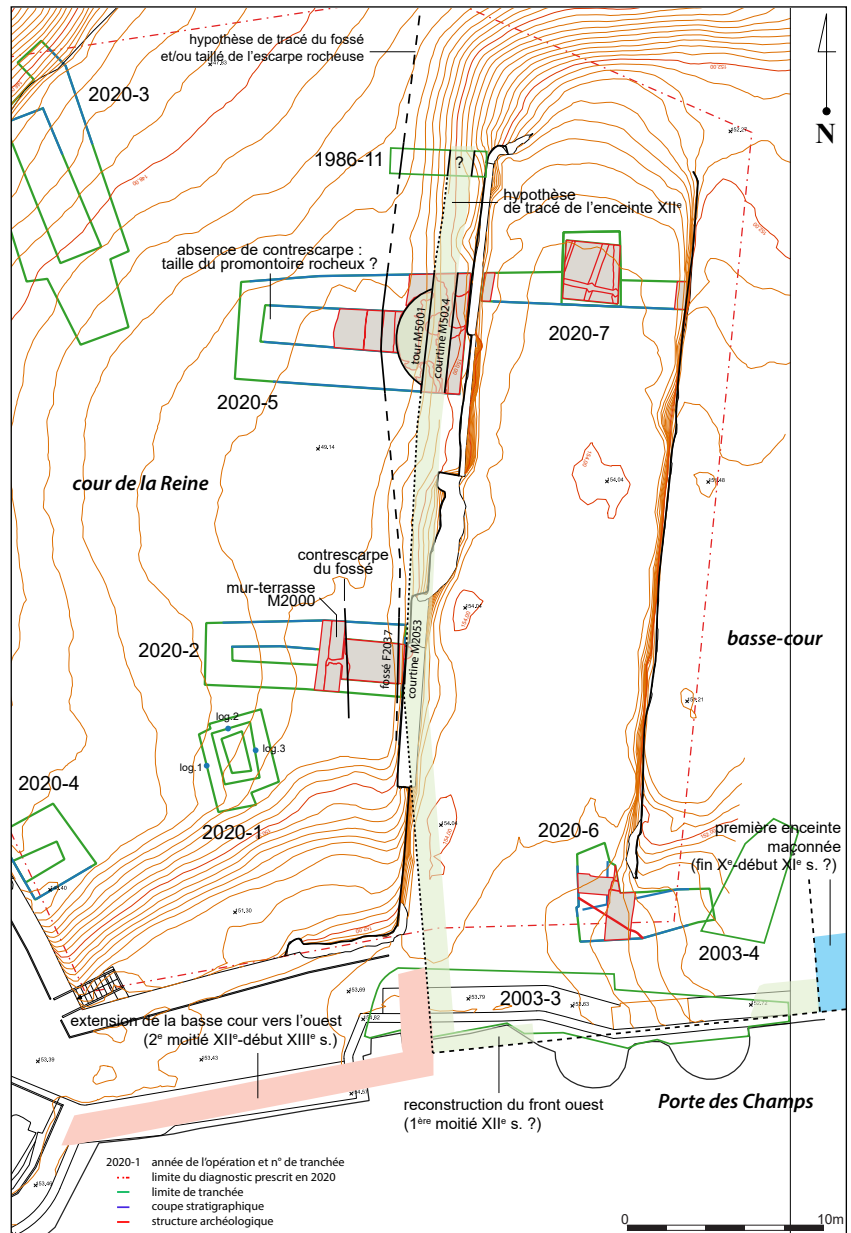
Falaise, Château, Cour de la Reine : détails des vestiges liés à l'évolution du front occidental de la cour et hypothèses de restitution (SIG : J.-M. Palluau-Inrap ; DAO : M. Lallauret d'après Brown et al. , fig. B-1 ; Carré 2003, fig. 5 ; Couesnon 1986, fig. 81 et plan de situation ; Mastrolorenzo 2012a, pl. 00 ; Saint Jores 1998, fig. 6).
