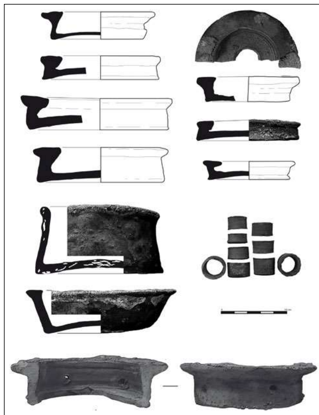
Le Tronquay, Le Pré de la Tuilerie : pièces techniques d'enfournement découvertes dans les fosses-carrières qui ont servi de dépotoirs (É. Gallouin).
