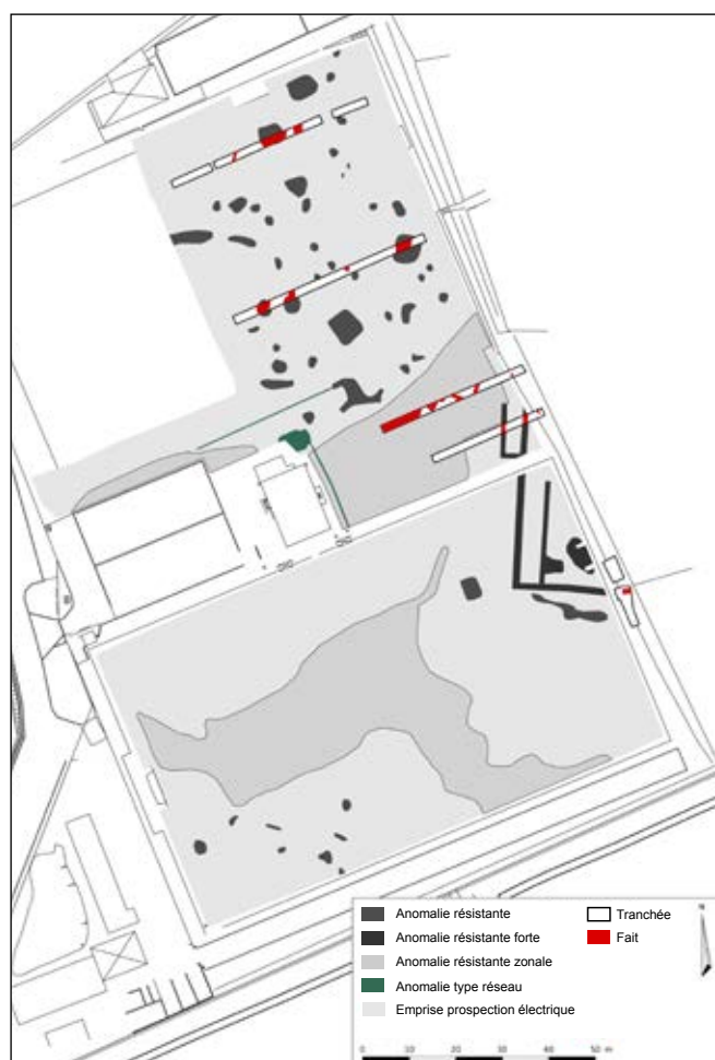
Saint-Pierre-de-Varengeville, chemin de la Messe : plan général des vestiges avec la géophysique (G. Hulin, S. Calduch, G. Gadebois).
