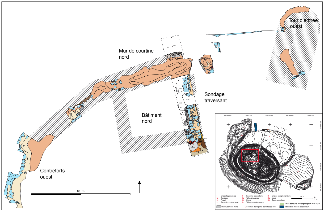
Maulévrier-Sainte-Gertrude, La Butte au Diable, fig. 1 : plan des sondages 2018 (A. Painchault).
