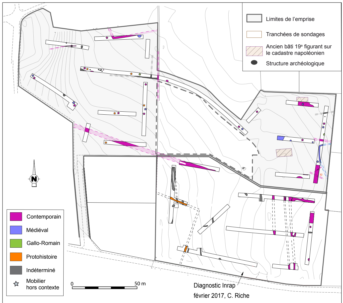
Saint-Romain-de-Colbosc, route de Saint-Laurent : plan général des vestiges (topographie : S. Calduch, DAO : C. Beurion).
