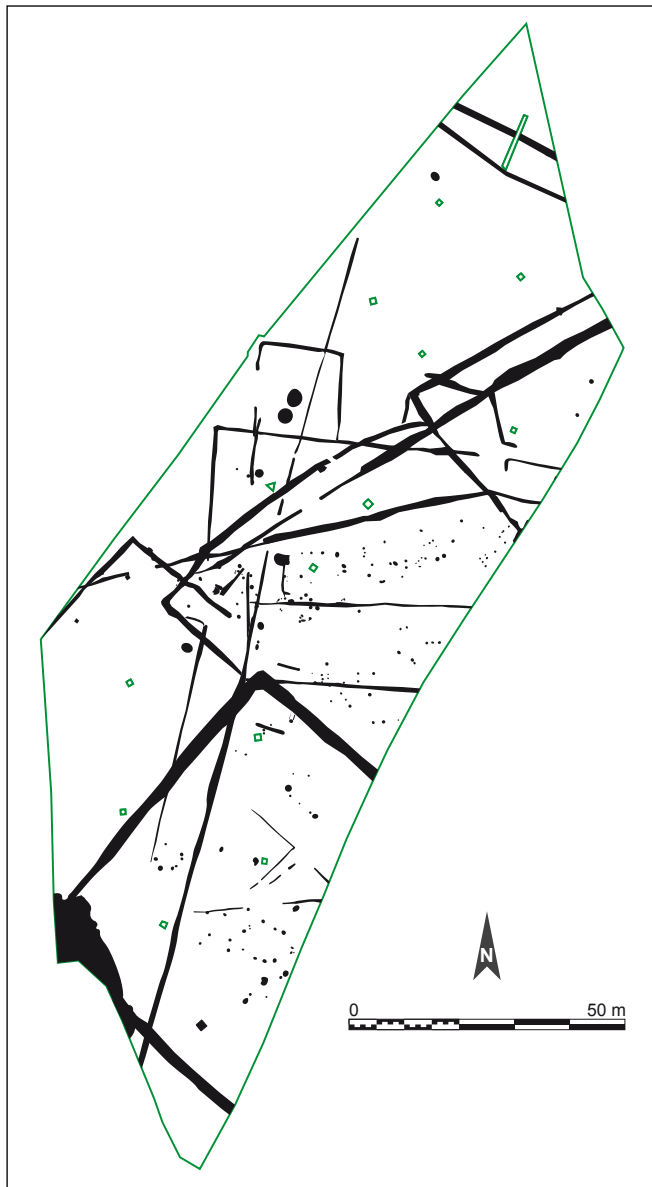
Heudebouville, ZAC Écoparc 3, fig. 2 : plan des découvertes de la zone 2 (V. Dartois).
