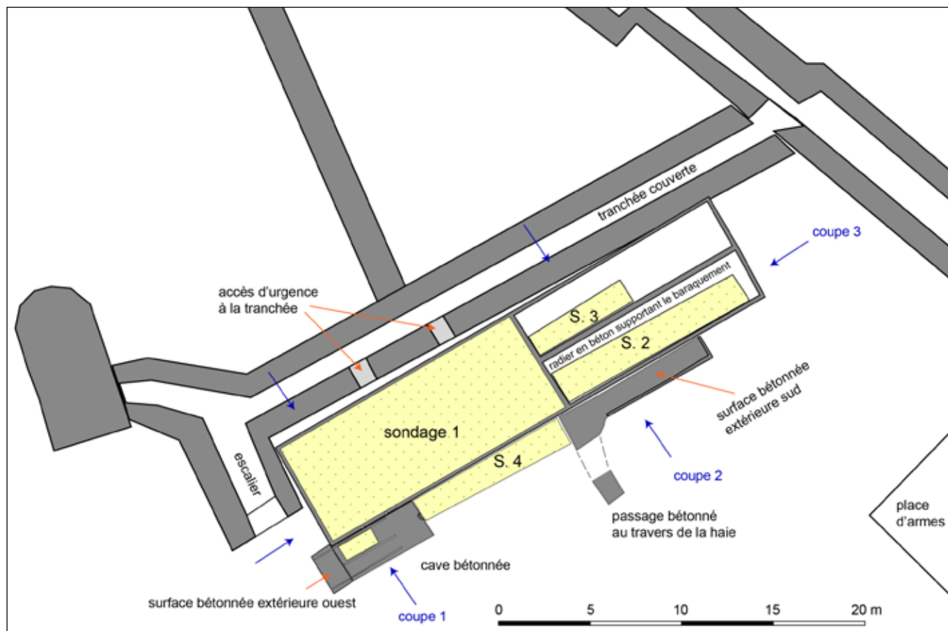
Azeville, batterie, le casino : plan général de la batterie et localisation des sondages (C. Billard).
