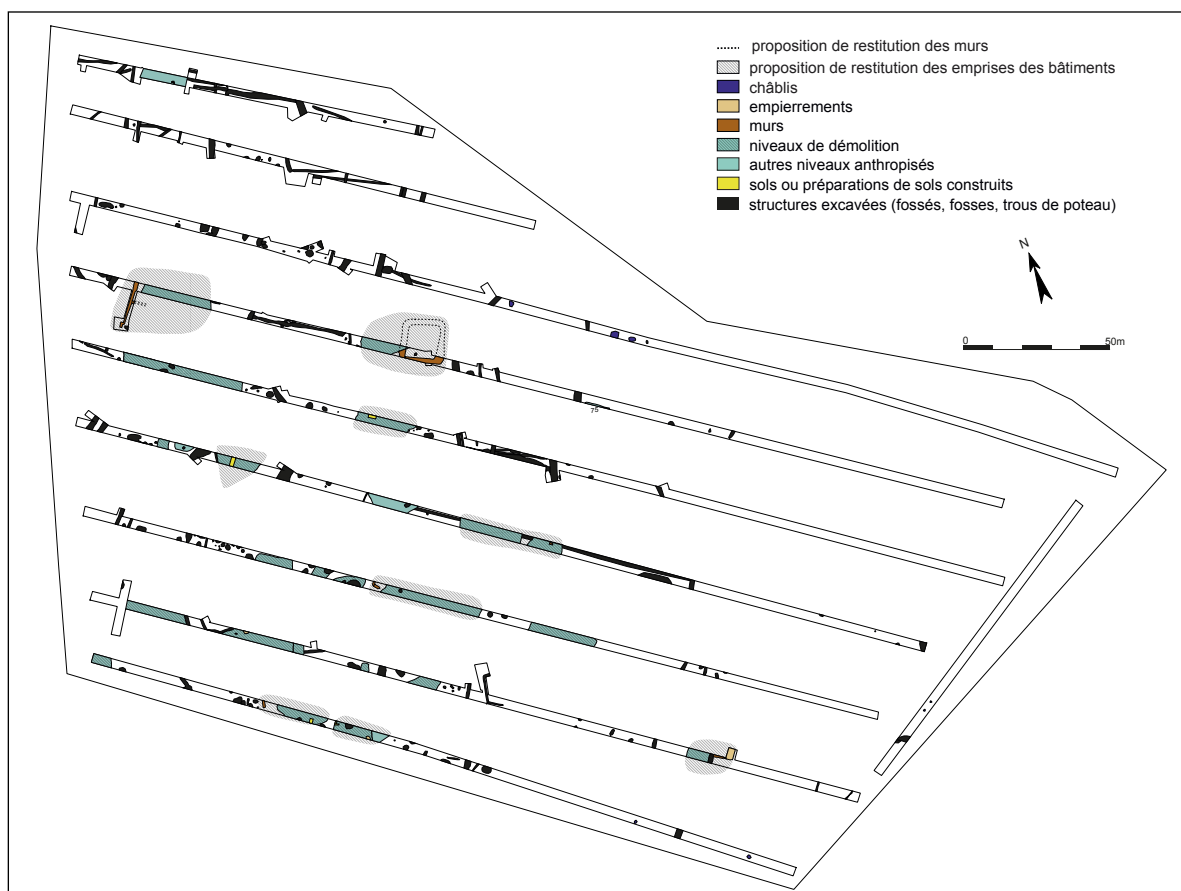
Cagny, Les Hameaux du Bois : plan de masse avec typologie des structures (J. Veron).
