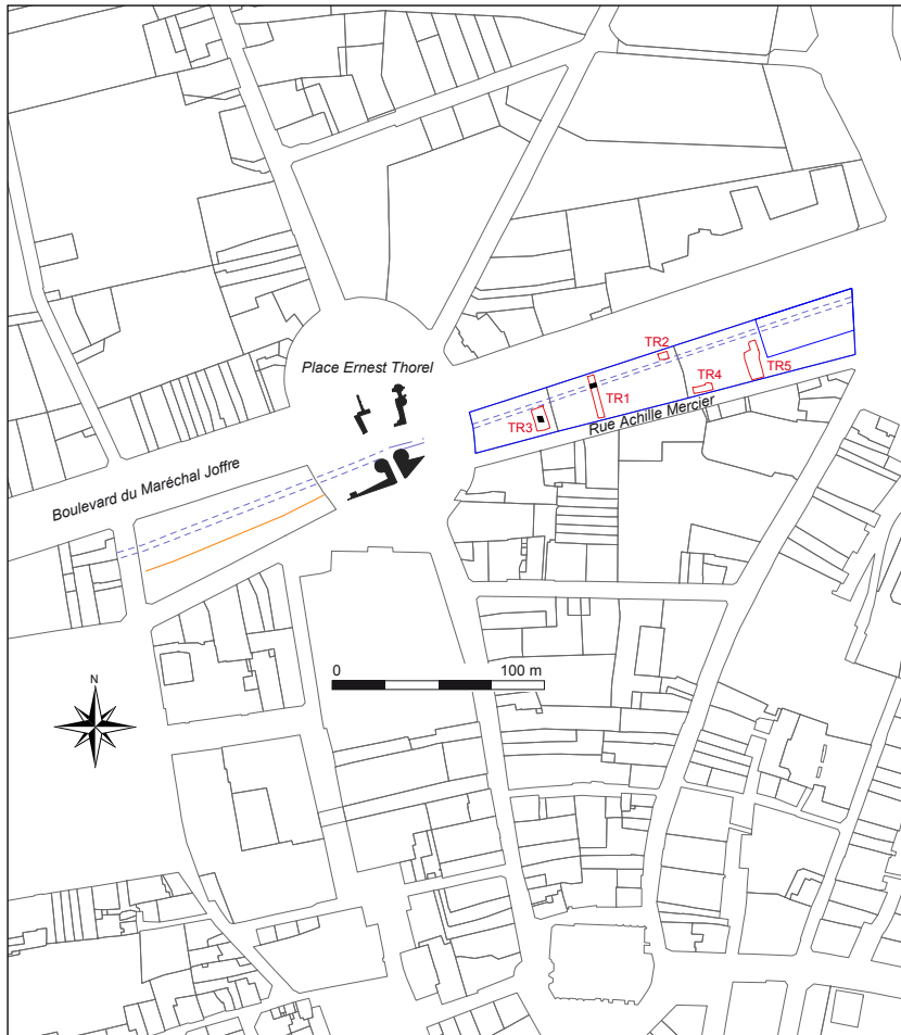
Louviers, 8 place Ernest Thorel : recalage des tranchées et maçonneries sur le cadastre actuel avec les portions connues de la Porte de Rouen sur la place Ernest Thorel (Le Cain 2002), en orange le tracé du fossé observé lors du diagnostic de 2009 (Guillot 2009) et en pointillé la Ravine (B. Guillot).
