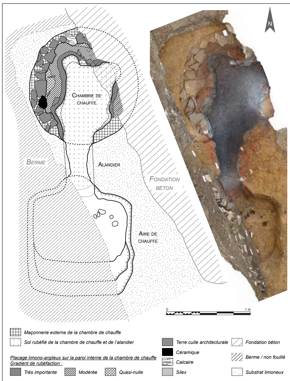
Évreux, 7 rue du Capitaine Herriot, fig. 1 : plan et orthophotogrammétrie du four de potier (P. Wech).
