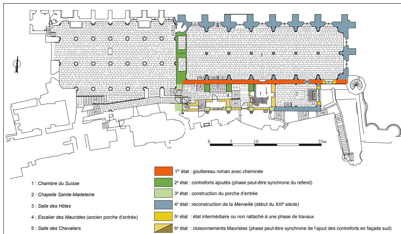
Le Mont-Saint-Michel, La Chambre du Suisse, fig. 2 : les principales phases de construction (E. Esnault d'après un fond de plan d'AGP).
