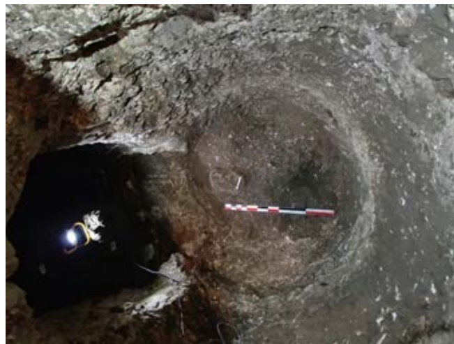
Le Vieil-Évreux, La Basilique, fig. 2 : fond de fouille du puisard. Sur la gauche, l'entrée de la galerie vue de la margelle devant la galerie réduisant le conduit (P. Clerc).
