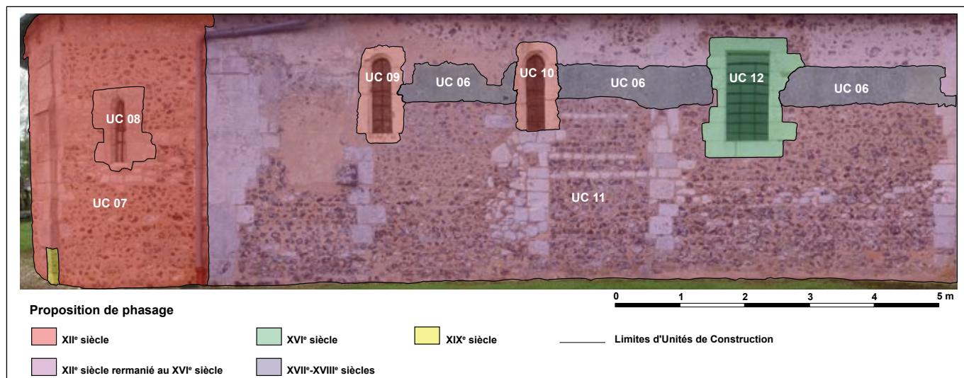
La Trinité-de-Thouberville, Église de La Sainte-Trinité, fig. 4 : façade nord du chœur et de la nef (partie orientale) (N. Wasylszyn).
