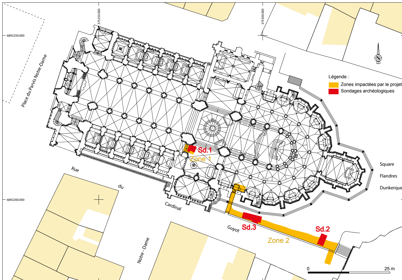
Coutances, Cathédrale : plan de la cathédrale avec la localisation des sondages du diagnostic (plan : CRMH ; DAO : F. Sanz Pascual).
