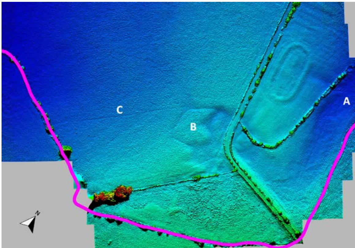
Métallurgie et hydraulique en Pays de Bray : zoom du MNT de 90 ha réalisé au sud de Forges-les-Eaux (C. Colliou, Métascan).
