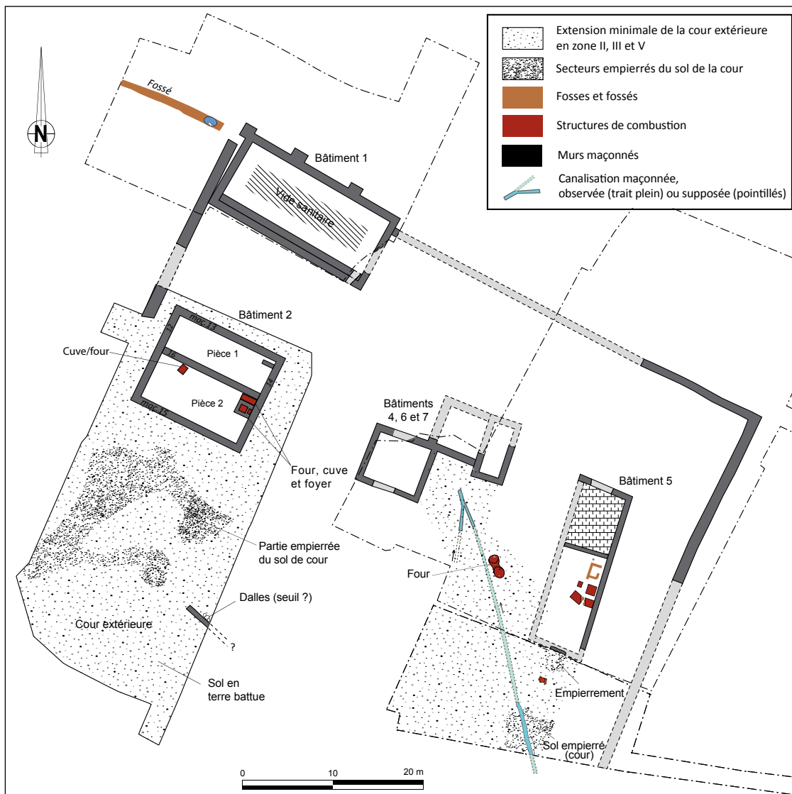
Commes, Le Dessous des Cotis : plan des vestiges de la phase 3-1 (C. Allinne).
