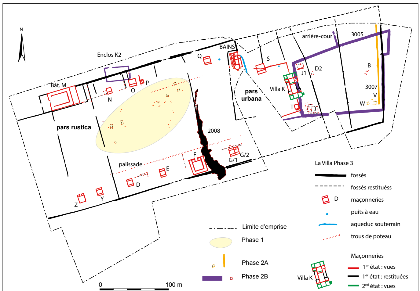
Vire-Normandie, ZAC de la Papillonnière, fig. 1 : plan général simplifié des structures protohistoriques et antiques (G. Guillier, L. Vipard).
