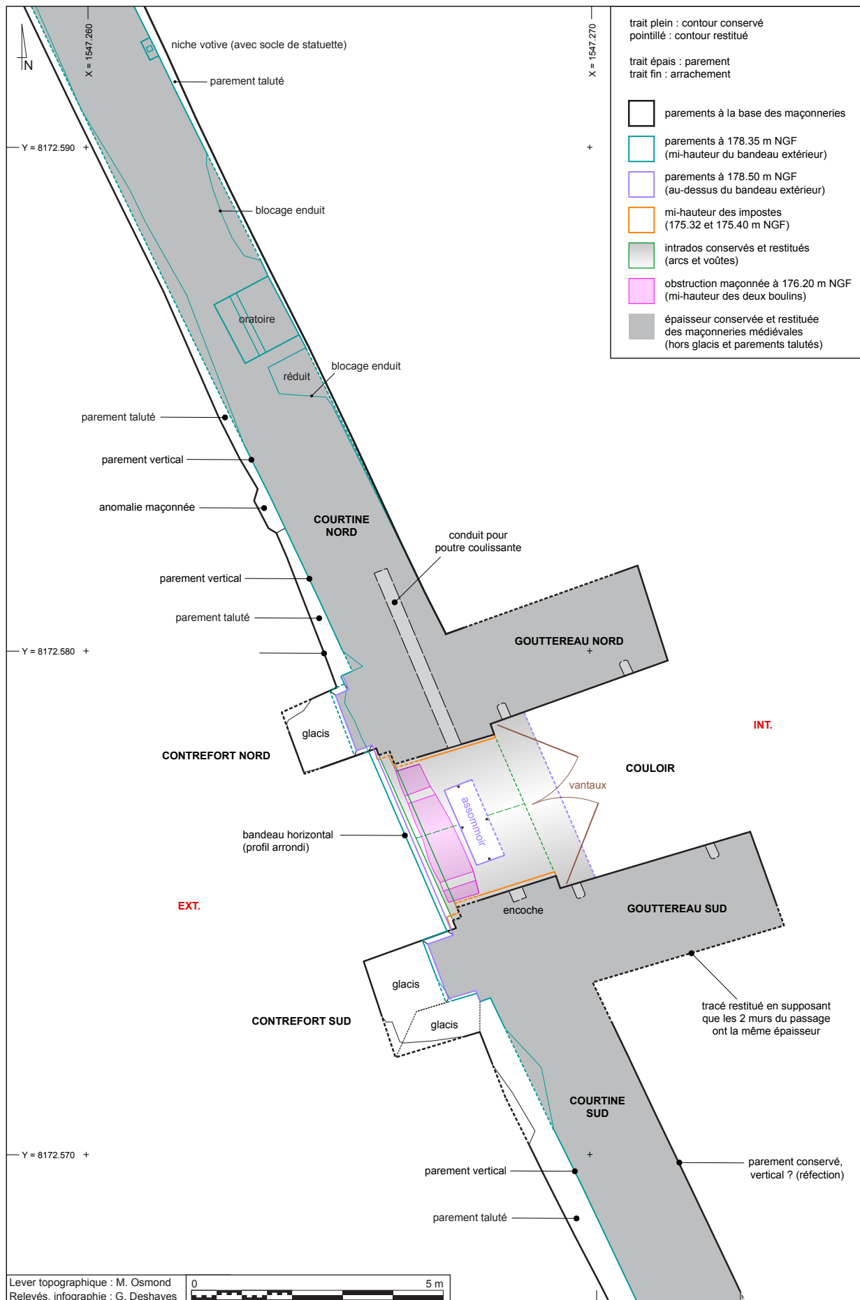
Verneuil-d'Avre-et-d'Iton, abbaye Saint-Nicolas : plan de la Porte d'Armentières et des courtines adjacentes (G. Deshayes).
