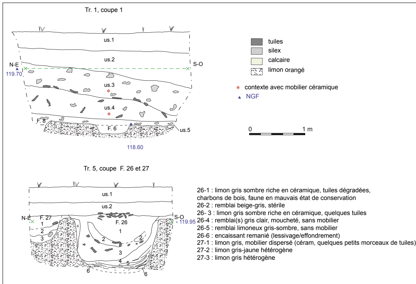
Saint-Pierre-de-Varengville, 41 route du Paulu : coupe stratigraphique (tr. 1) et coupe partielle de deux fosses antiques (Y-M. Adrian, S. Le Maho).
