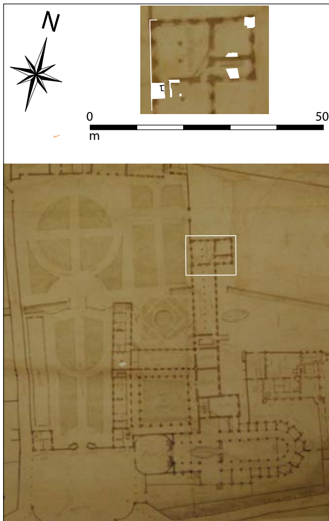
Rives-en-Seine, Abbaye Saint-Wandrille de Fontenelle : recalage des maçonneries mises au jour lors du diagnostic sur un plan de 1756 (documentation CRMH de Normandie coté ADSM n°57).
