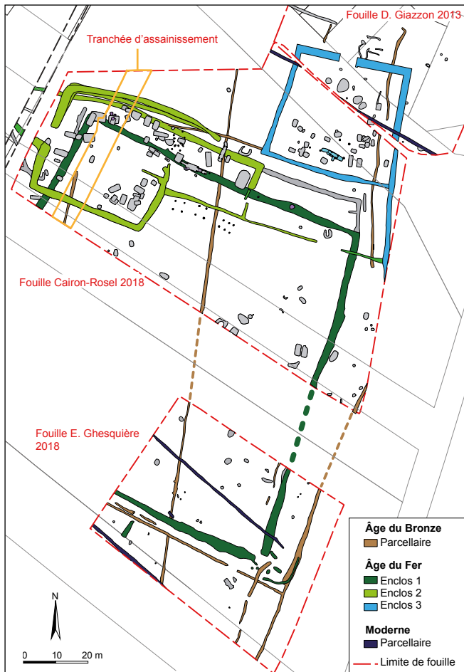
Cairon, Rosel, rue de Rots : plan compilé des opérations de fouille (C.-C. Besnard-Vauterin).
