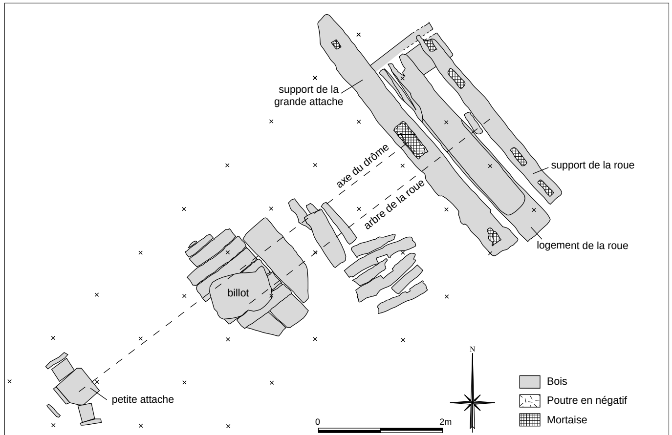
Beaussault / Compainville, « Moulin de Glinet » : Plan interprétatif du gros marteau
