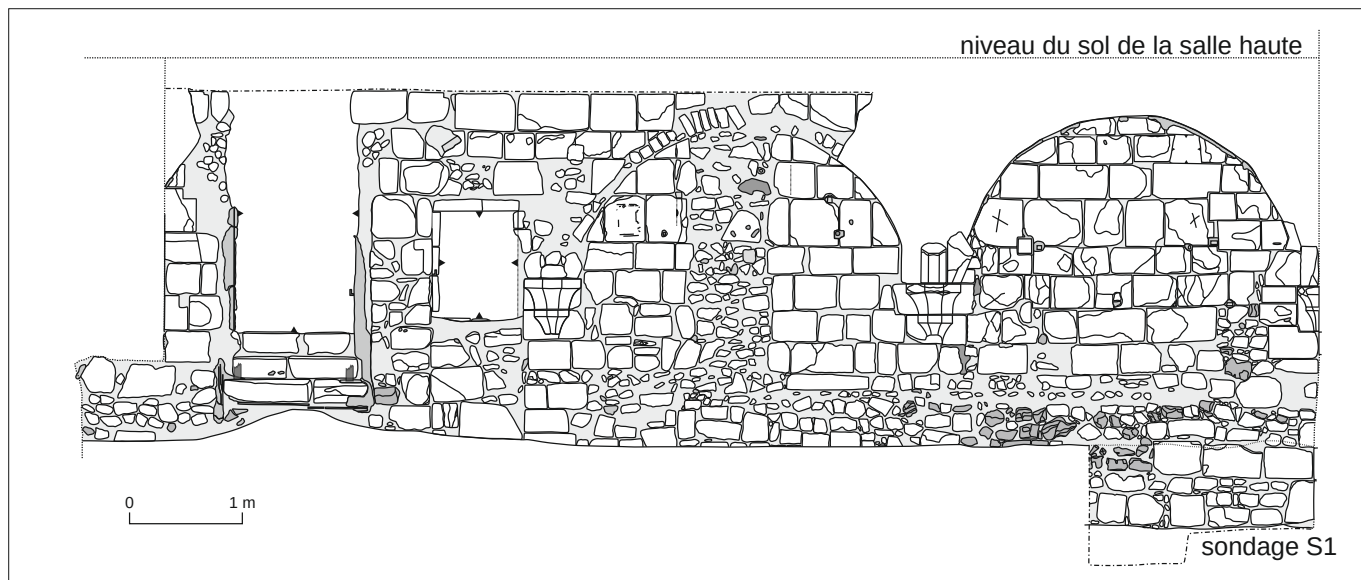
Jumièges, Abbaye : Parement de la façade ouest de l'hôtellerie, reprise en sous-oeuvre et ancrage des voûtes de la salle basse de la maison nord (relevé et mise au net G. Deshayes)
