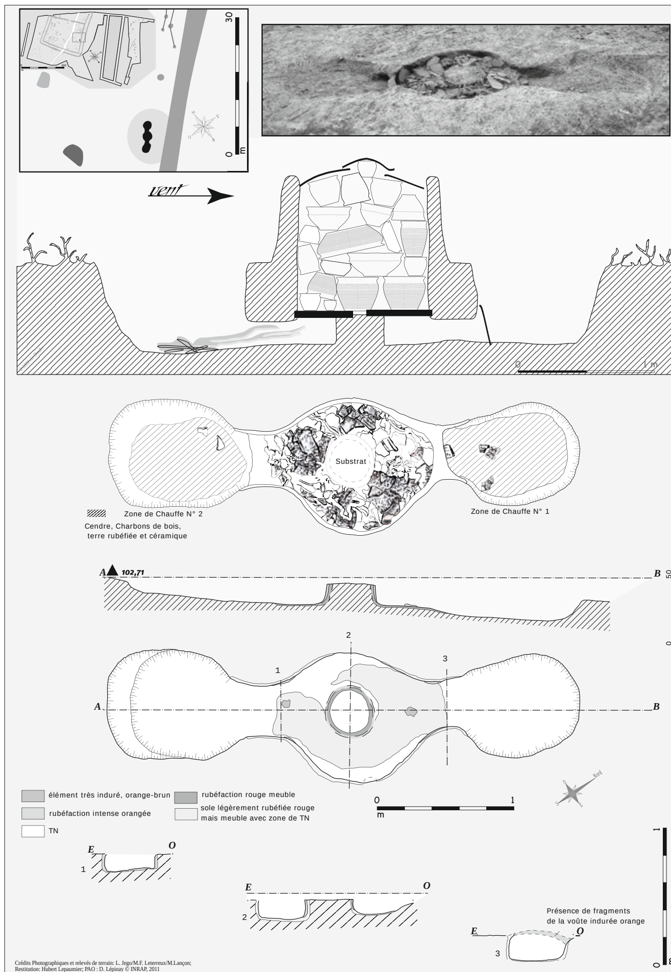
Évreux, « Zac de Cambolle – Le Golf » : Relevés et reconstitution du four de potier (M.F. Leterreux, M. Lançon, H. Lepaumier)
