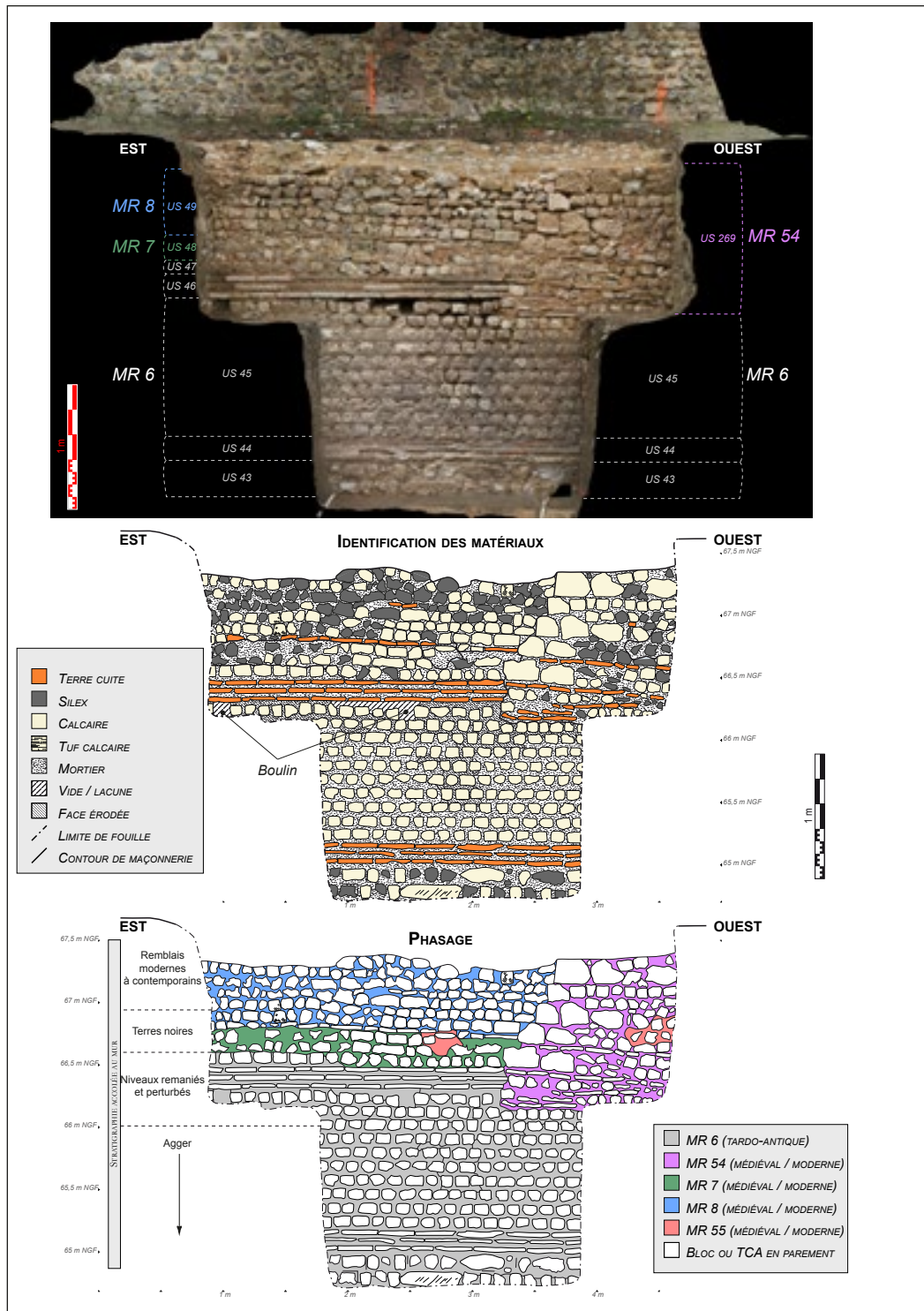
Évreux, Jardins de l'évêché : vue, relevé et étude du parement conservé du rempart mis au jour dans l'un des sondages (P. Wech).
