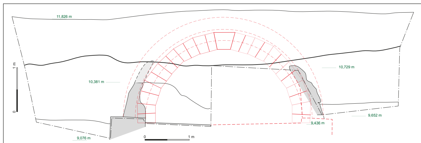
Le Vaudreuil, Le Golf, fig. 3 : relevé nord de la voûte et projection proposée (relevé topographique : S. Calduch ; DAO : N. Roudié).
