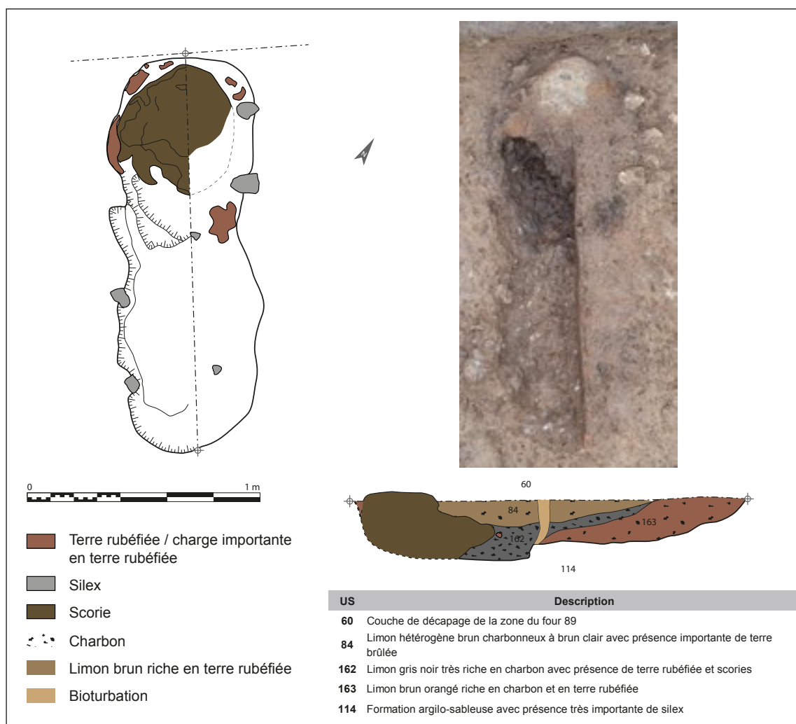
Heudebouville, Écoparc 3 : plan et coupe du four de réduction (V. Dartois).
