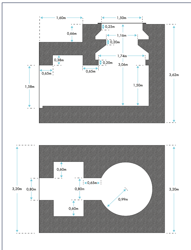
Courseulles-sur-Mer, Juno Beach: plan du Tobrouk et de l'abri (Centre Juno Beach).
