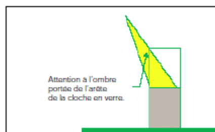
2. Eclairage extérieur d'une vitrine centrale.
