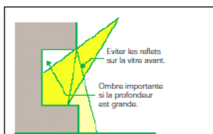
3. Eclairage extérieur d'une vitrine murale.
