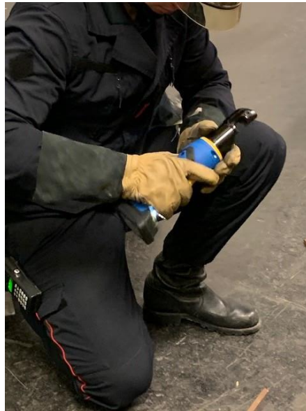
Coupe-pédale pouvant être employé pour sectionner les tringles (temps d'intervention : 5s)
