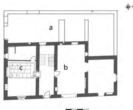
Plan de rez de chaussée. a : bâtiment primitif b : Jauregia c : fouloir pressoir.
