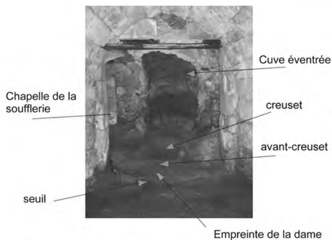
Haut-Fourneau nord, vue par la chapelle de coulée après nettoyage des déblais.
