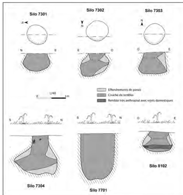
Plans et coupes des silos médiévaux.
