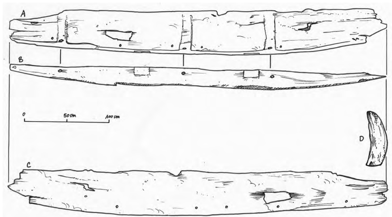
Saint-Jean-de-Marsacq - Le chaland polyxyle. Relevé du chaland.
