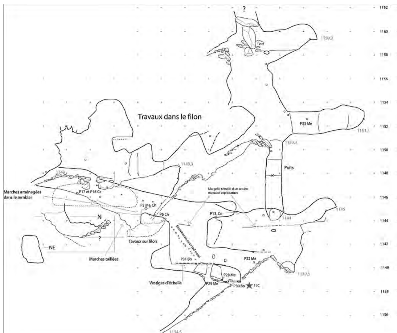
Banca - Site minier de Mehatze. Coupe de la zone complexe de chantiers superposés, dans la colonne minéralisée.
