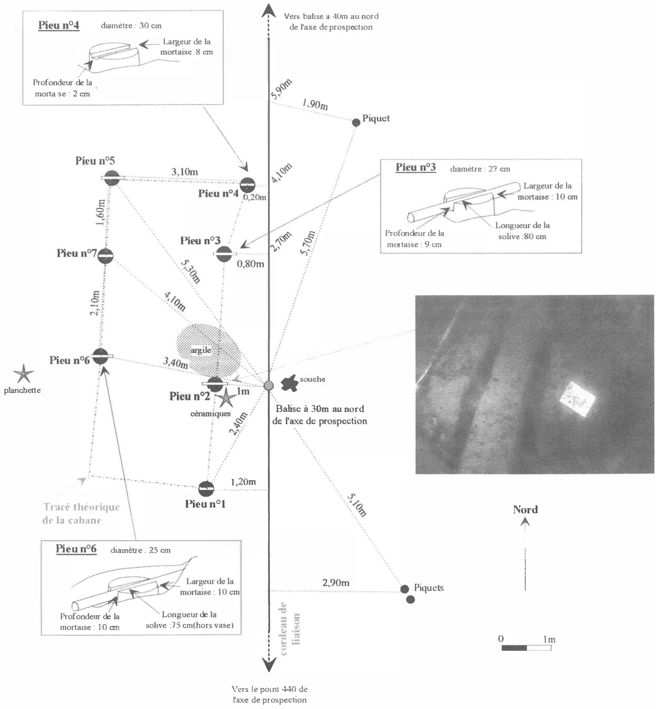
Sanguinet - Put Blanc. Relevé en plan de la cabane.
