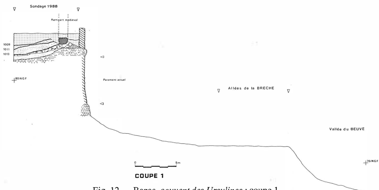
Fig. 12 — Bazas, couvent des Ursulines : coupe 1.
