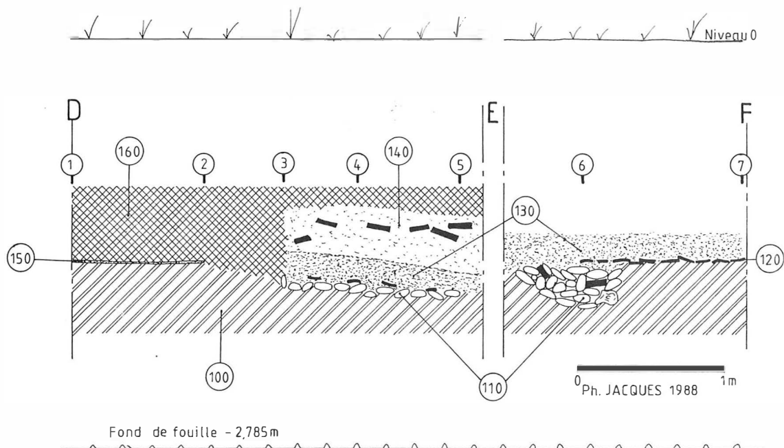
Fig. 47 — Agen, Résidence Jayan : coupe stratigraphique.
