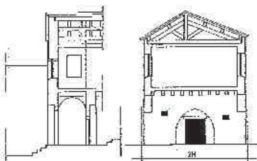
55 rue Saint-Jacques - coupe sur le pontet. L'arc brisé a été remplacé par une simple porte. A l'intérieur l'arrière-voûture domoûre.
