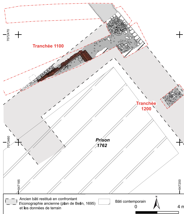
SAINT-OMER Motte Castrale Plan de synthèse des maçonneries de l'édifice castral découvertes lors du diagnostic, DAO M. Delage - CDA - CG62.
