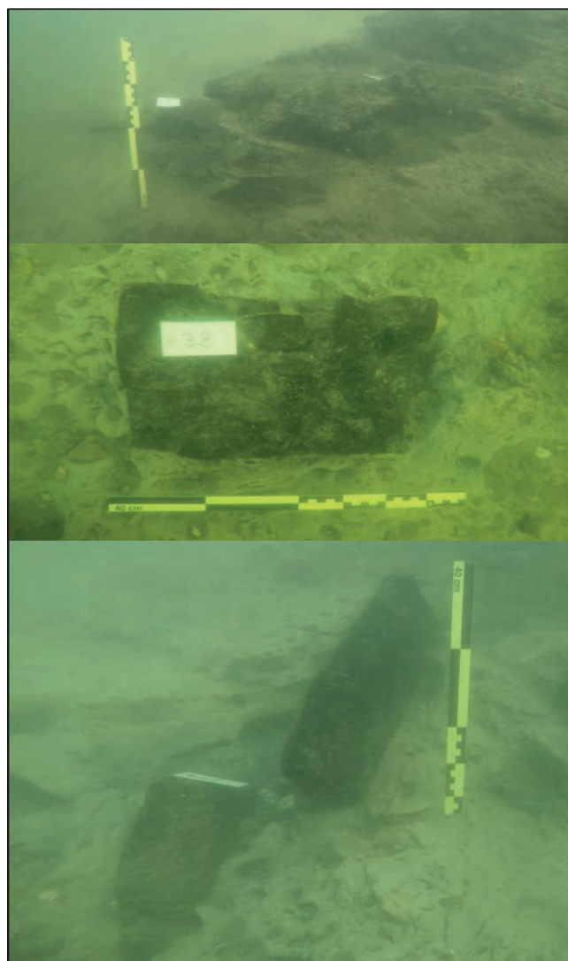
Saintes, La Prée basse, éléments de la structure : madriers horizontaux (en haut), madriers vertical (au milieu) et planches (en bas). (photos : M. Cayre).
