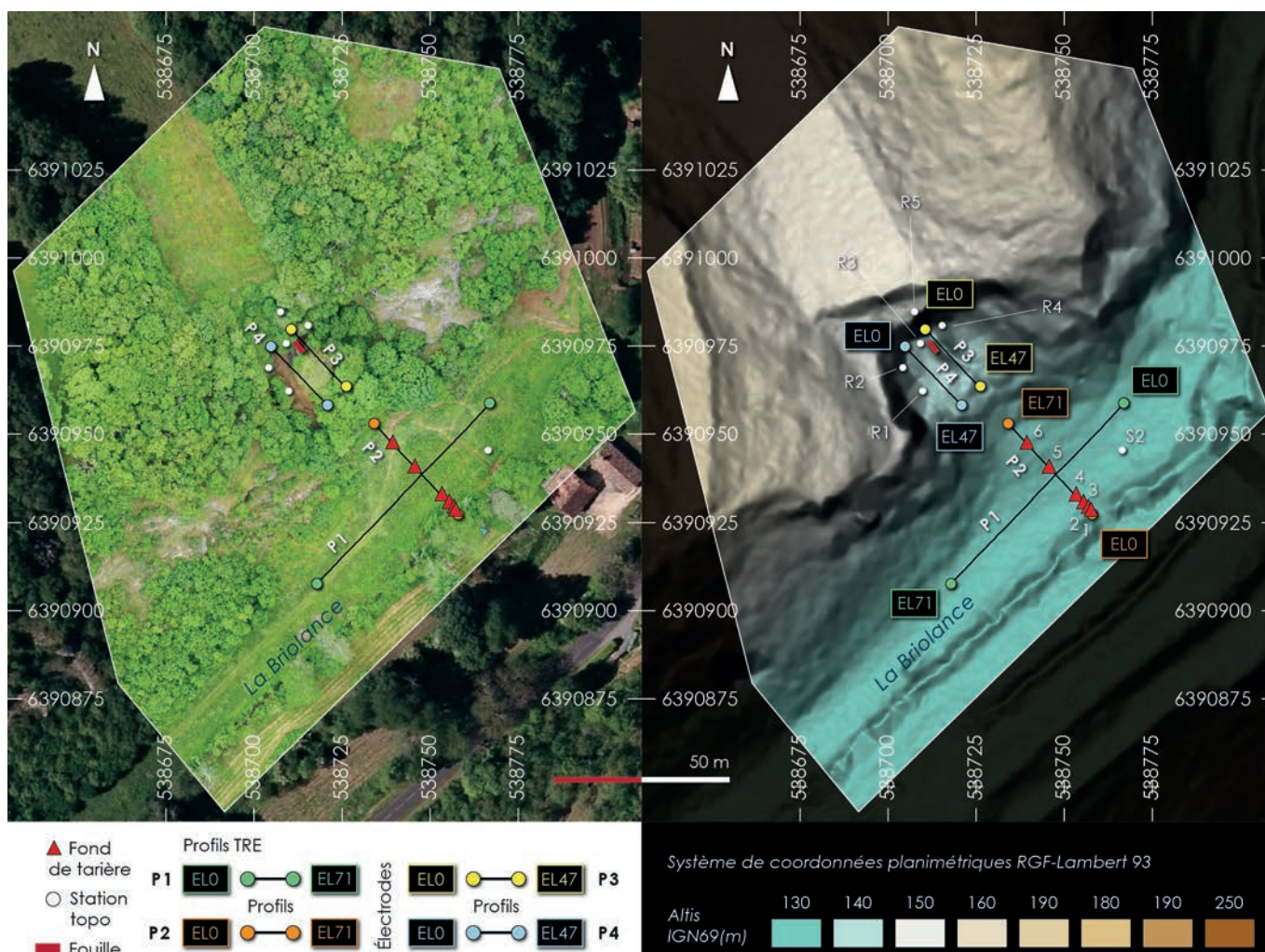
BLANQUEFORT-SUR-BRIOLANCE - La Borie del Rey. Vue nadir du gisement et de la plaine alluviale avec localisation des profils de résistivité électrique (CAO Archéosphère).
