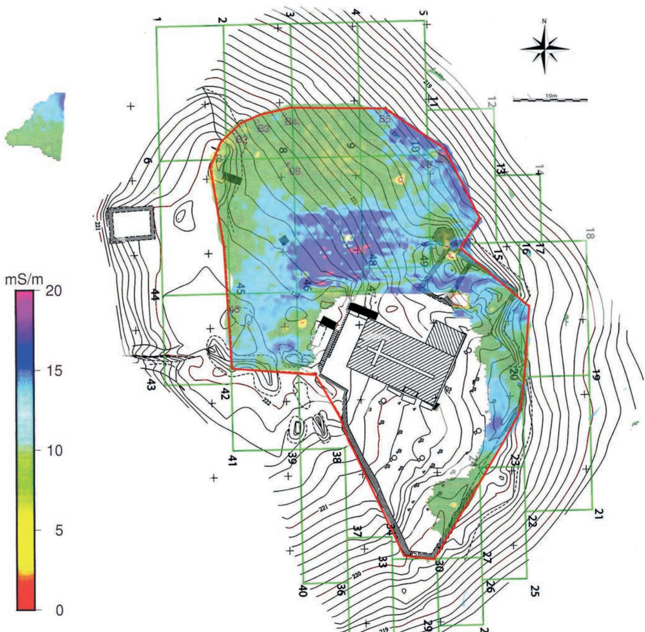
LARCEVEAU-ARROS-CIBITS - Eglise Saint Sébastien d'Arros Cartographie électromagnétique du sous-sol aux abords de l'église d'Arros. © D. Rousset et G. Sénéchal, UPPA.
