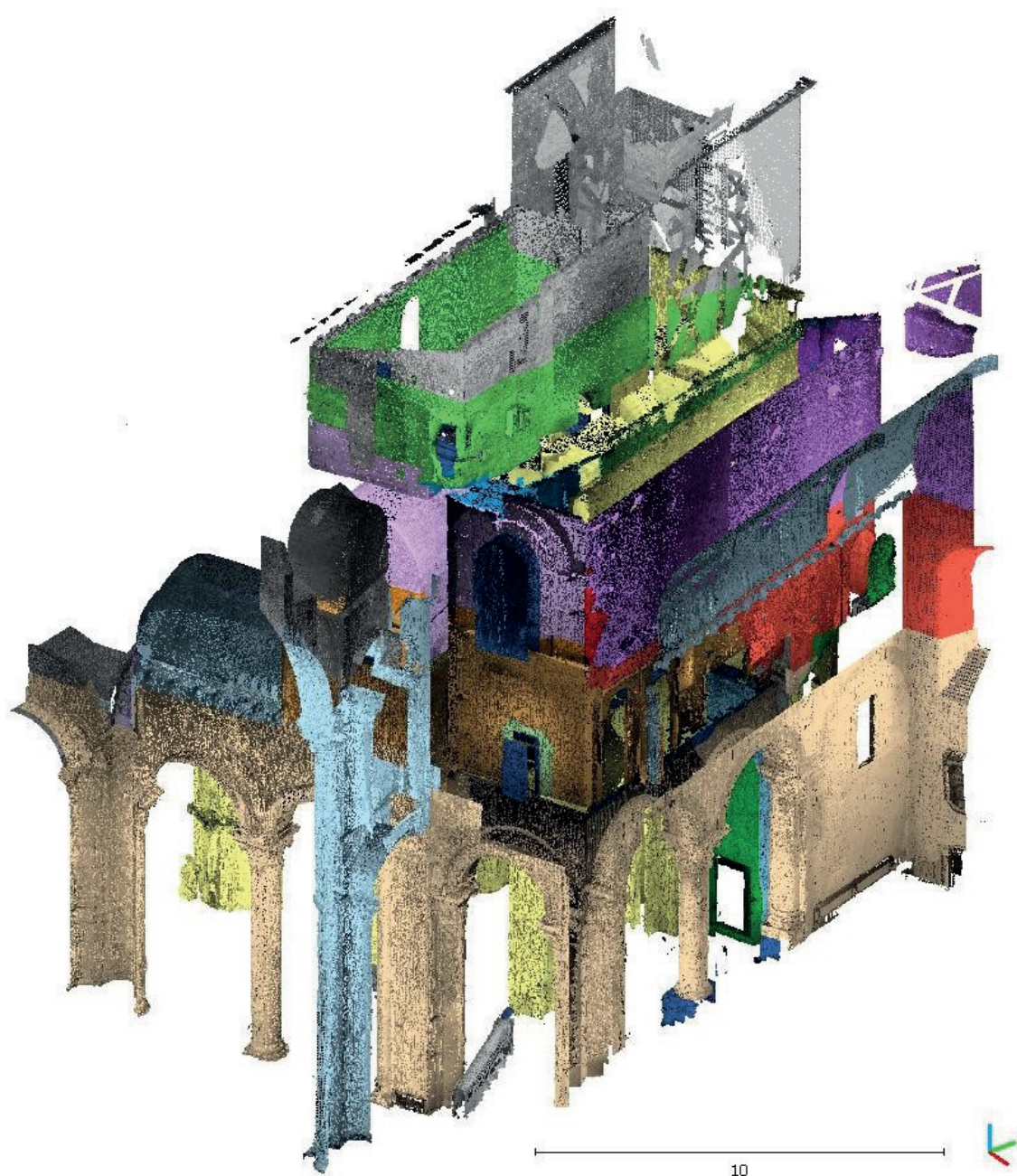
Poitiers, Saint-Hilaire-le-Grand, tour-proche et jonction nef/transept, traitement volumétrique et phasage de la construction sous CloudCompare, vue depuis le sud ouest (DAO : Pauline Bessaguet)
