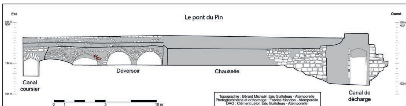
Béruges, Le pont du Pin, fig. 2 : Élévation sud du pont du Pin (DAO : C. Letor et E. Guilloteau)
