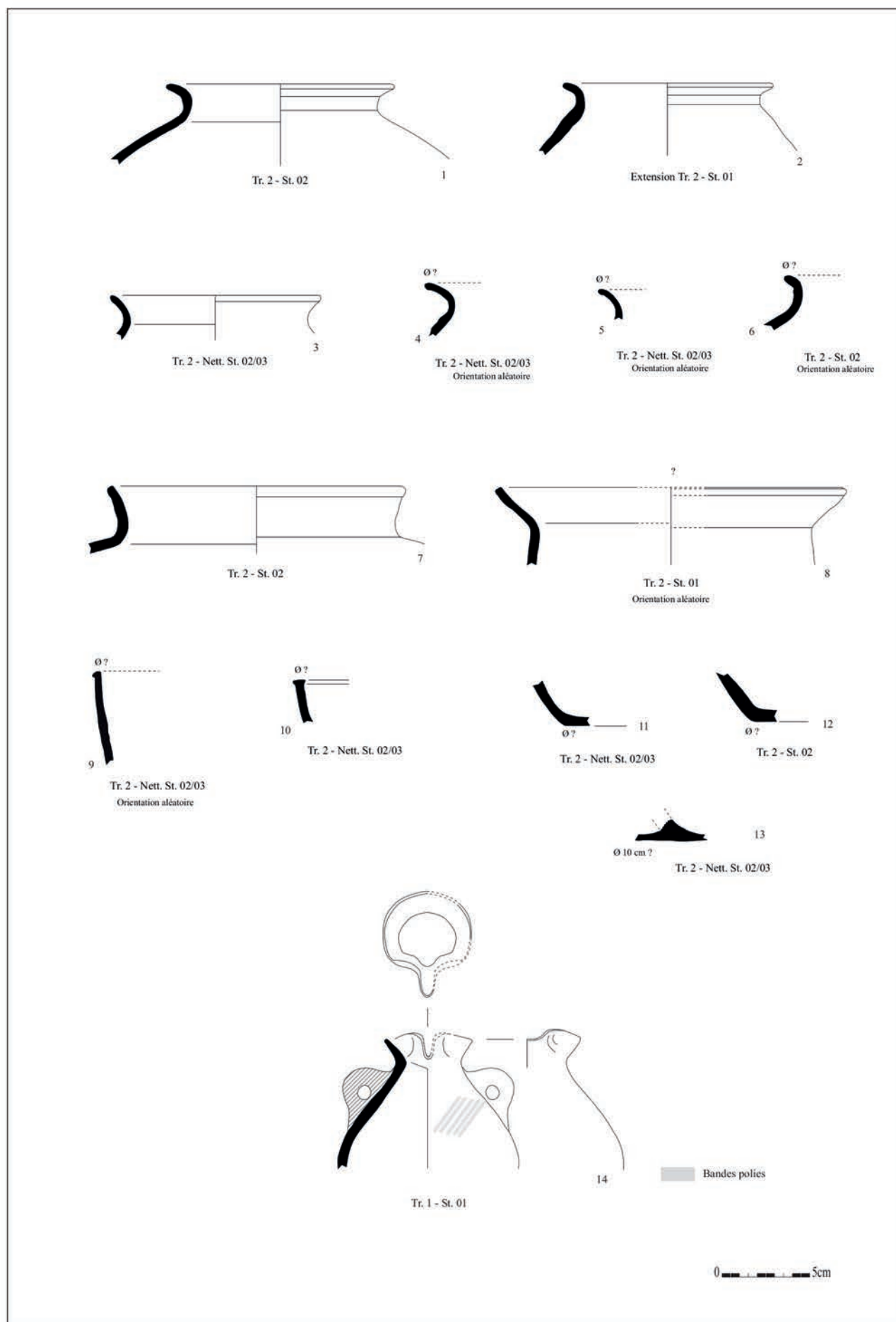
ASSON - Profils des différentes formes céramiques en pâte sableuse non tournée mises au jour lors du diagnostic (© Armelle Guériteau, INRAP).
