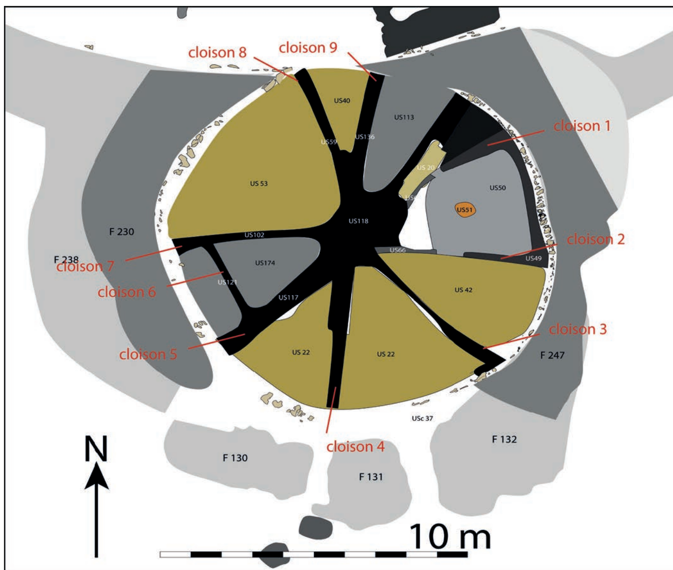
GELOUX Pouyet Sud, Figure 3 : Cloisonnement en matériau périssable de l'aire interne de la structure st1 dont le diamètre du cercle de pierre est de 13m (A. Bertaud).
