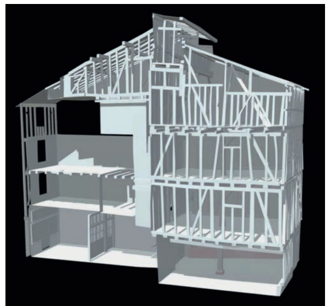
Limoges, modélisation 3D de la Maison de la Boucherie depuis le nord-ouest (P. Bessaguet, Sketchfab)
