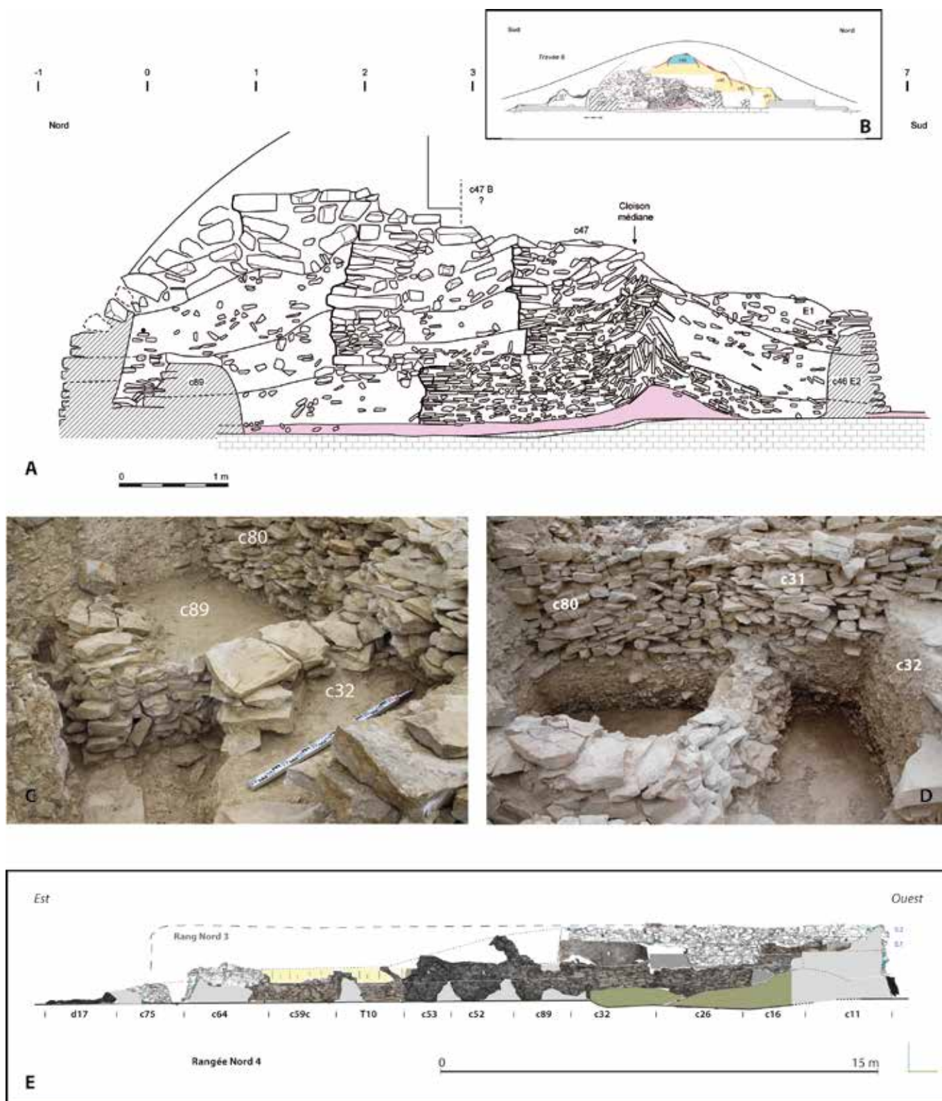
PRISSÉ-LA-CHARRIÈRE, Le tumulus C de Péré, fig. 2 : Analyse du bâti au sein du tumulus C de Péré à Prissé-la-Charrière (Plaine d'Argenson, Deux-Sèvres). A et B/ Coupe nord-sud du tumulus C, au sein de la travée 6 et pour les parties les plus profondes de la partie orientale de la masse tumulaire : à moins d'une étude ou d'un démontage attentif et détaillé du bâti dans les secteurs adjacents, l'interprétation des faits ici observés aurait pu être totalement erronée (cf. C et D). C et D/ A titre d'exemple, la présence de deux sections au sein des parois et du remplissage de l'alvéole c89, dont une seule de ces deux sections est chaînée avec d'autres constructions adjacentes, illustre cette complexité. E/ Seules de telles études du bâti permettent cependant d'identifier les éléments techniques nécessaires au chantier de construction, qui jusqu'à présent étaient largement passés inaperçus car progressivement intégrés au sein des structures qui assurent le maintien de la masse tumulaire : pour exemple, un plan incliné qui donne accès à une plateforme plus élevée, au sein de différentes rangées d'alvéoles, au nord. (DAO : L. Quesnel, clichés et photogrammétries : L. Laporte)
