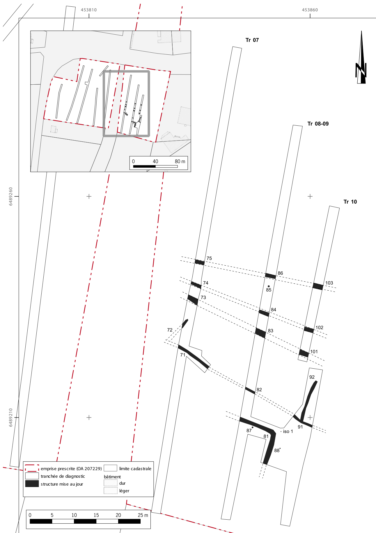
Barbezieux - Les Terres du Maine Neuf Fig. 1 : plan des structures archéologiques sur fond cadastral (cadastre : Direction générale des Finances Publiques ; relevé topographique P. Texier ; cartographie SIG : B. Moutarde).
