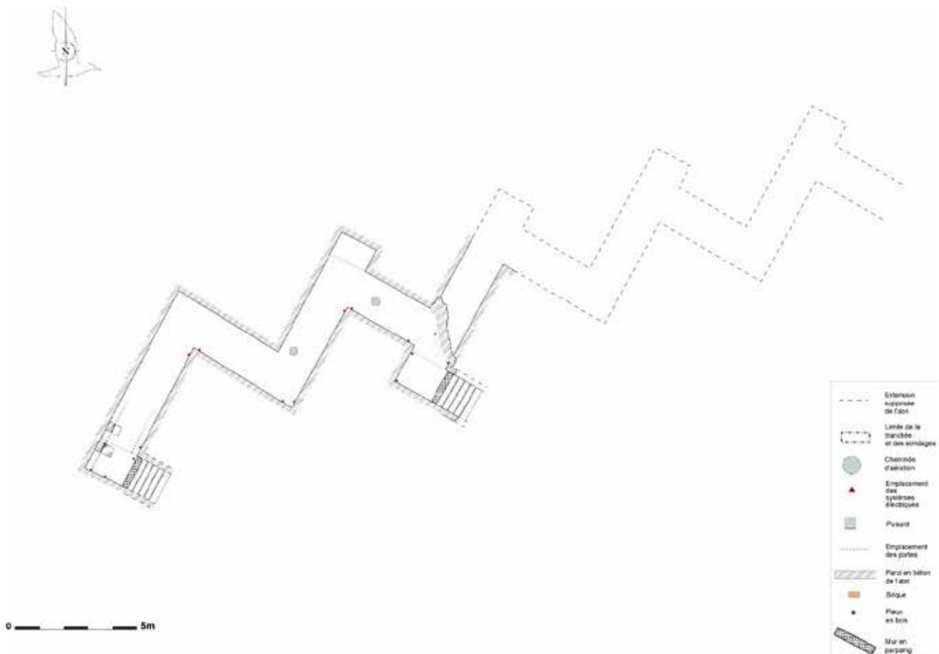
ROYAN, rue du Champ des Oiseaux, plan de l'abri de la Défense Passive (Dessin : Gay C.)
