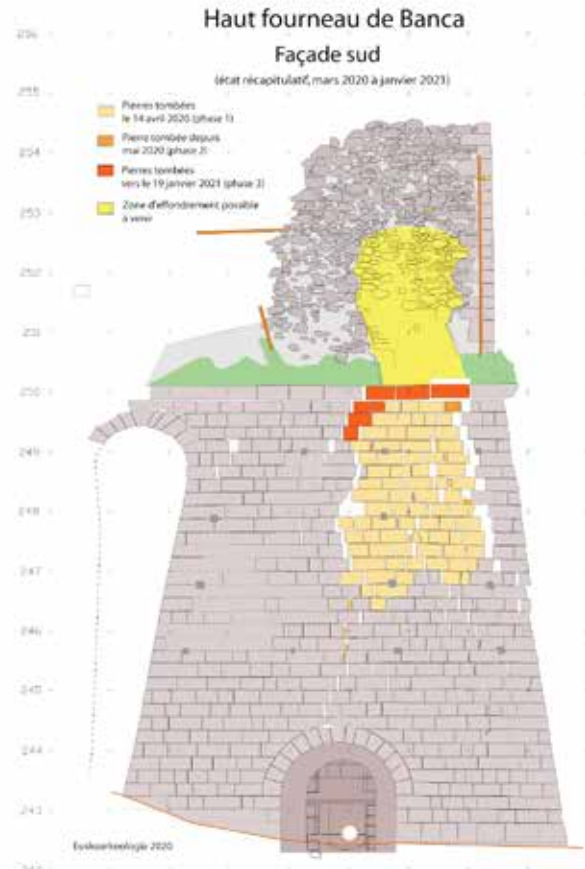
Haut-fourneau de Banca : à gauche : relevé de l'élévation de la façade est ; à droite : relevé de l'élévation de la façade sud (relevés : G. Parent, EuskoArkeologia)
