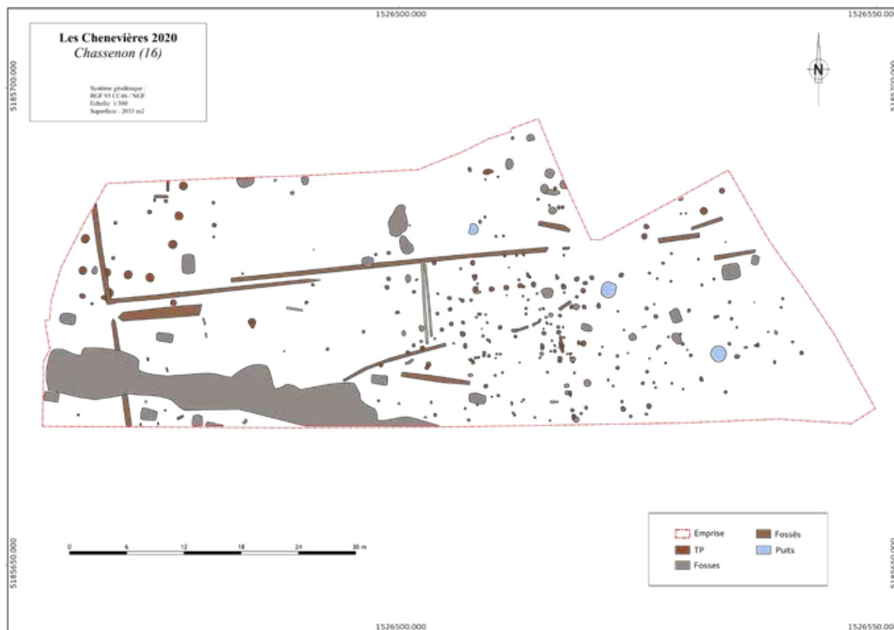
Chassenon - Les Chenevières : plan général des vestiges (topo et DAO : A. Dimeglio)
