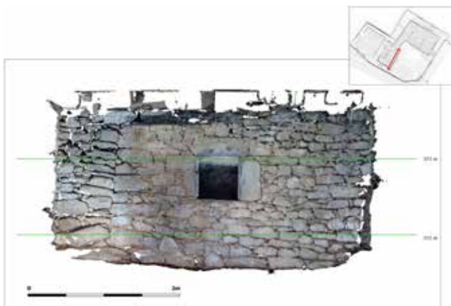
Photogrammétrie de l'une des parois de la cave de la dernière maison à gauche : probable accès à la surface, muré (Archéa-Archéo/Scan)
