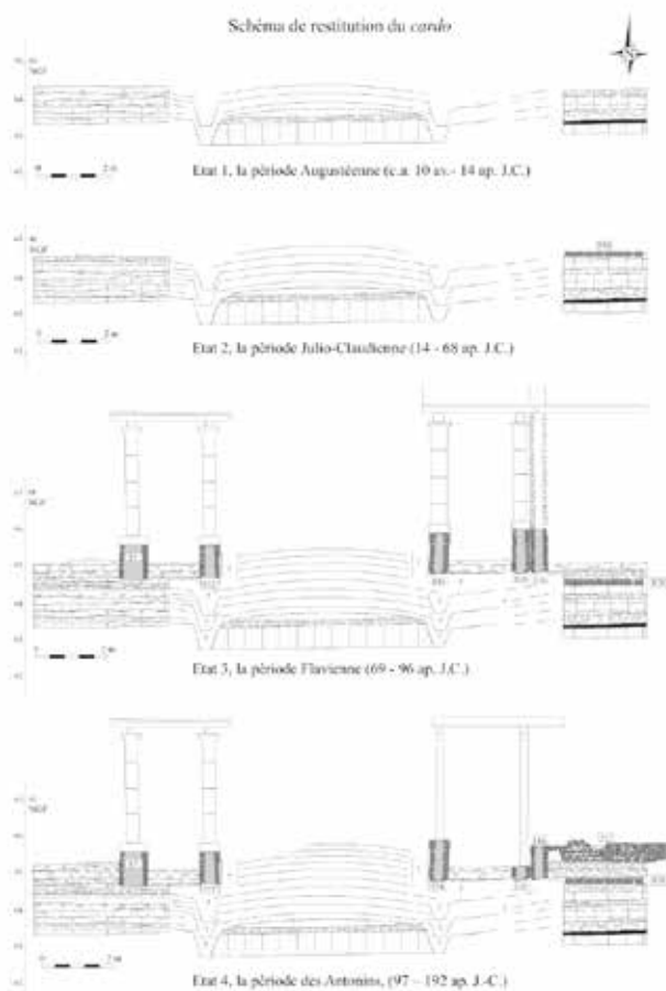
Agen - Fig.2 : schéma de restitution du cardo (cl. : W. Migeon, Inrap)
