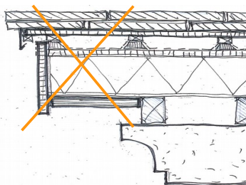
Tuile de rive à rabat non traditionnelle
