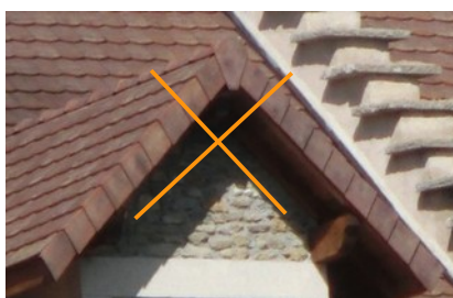
Surépaisseur en débord de toiture formant caisson
