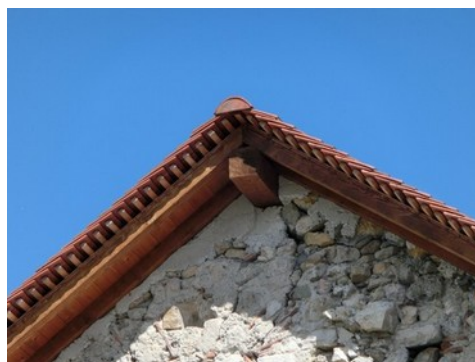
Avant-Pays savoyard Détail de toiture en pignon Rive avec tuiles saillantes sans zinguerie
