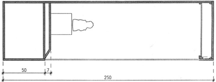
COUPE
