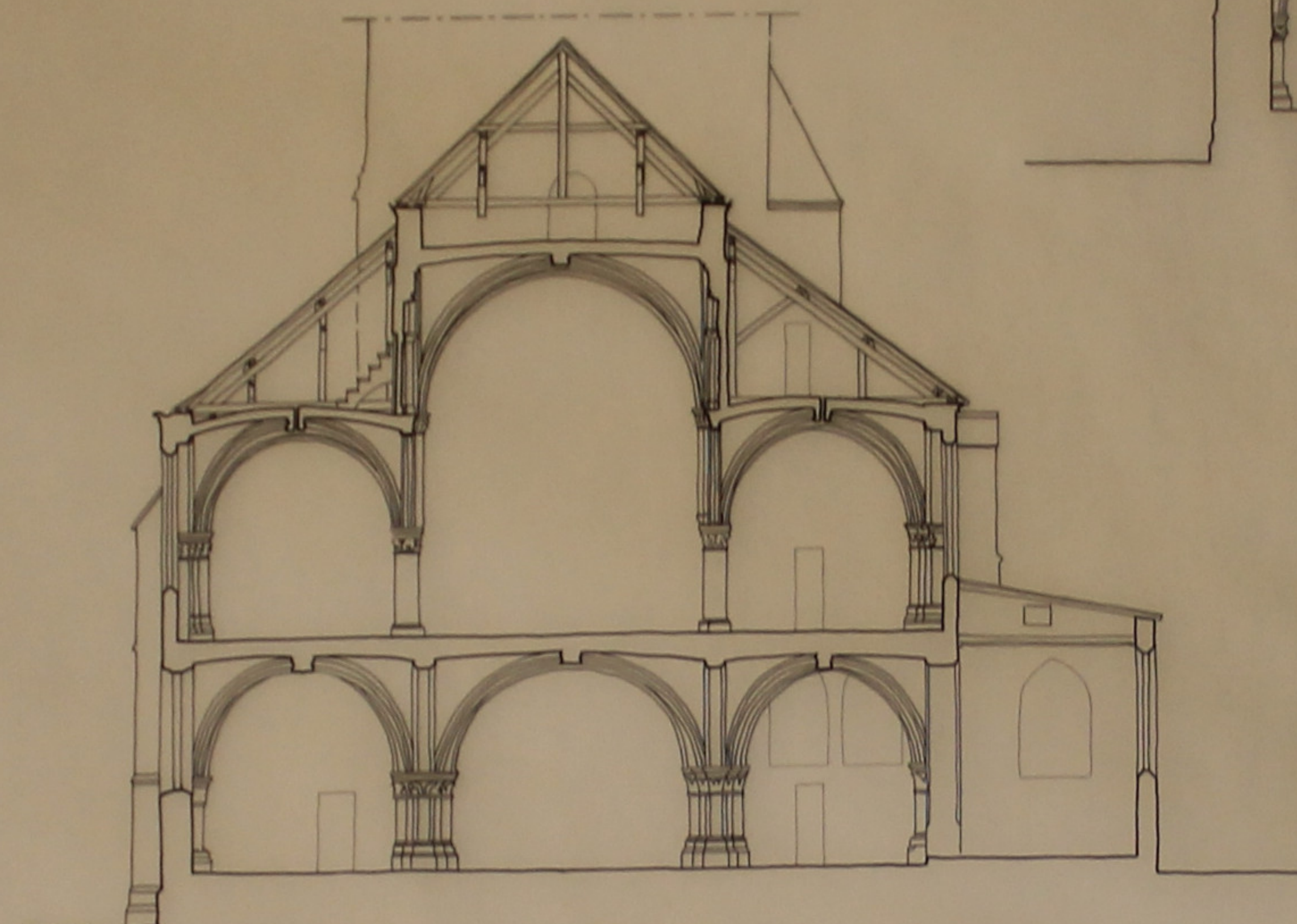
COUPE B-B
