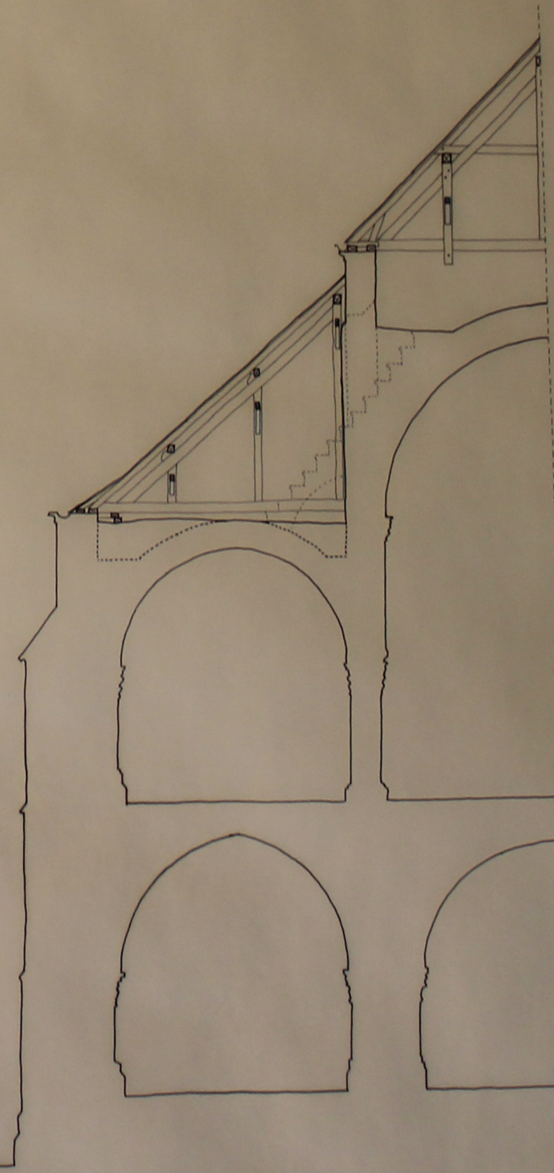
COUPE C-C
