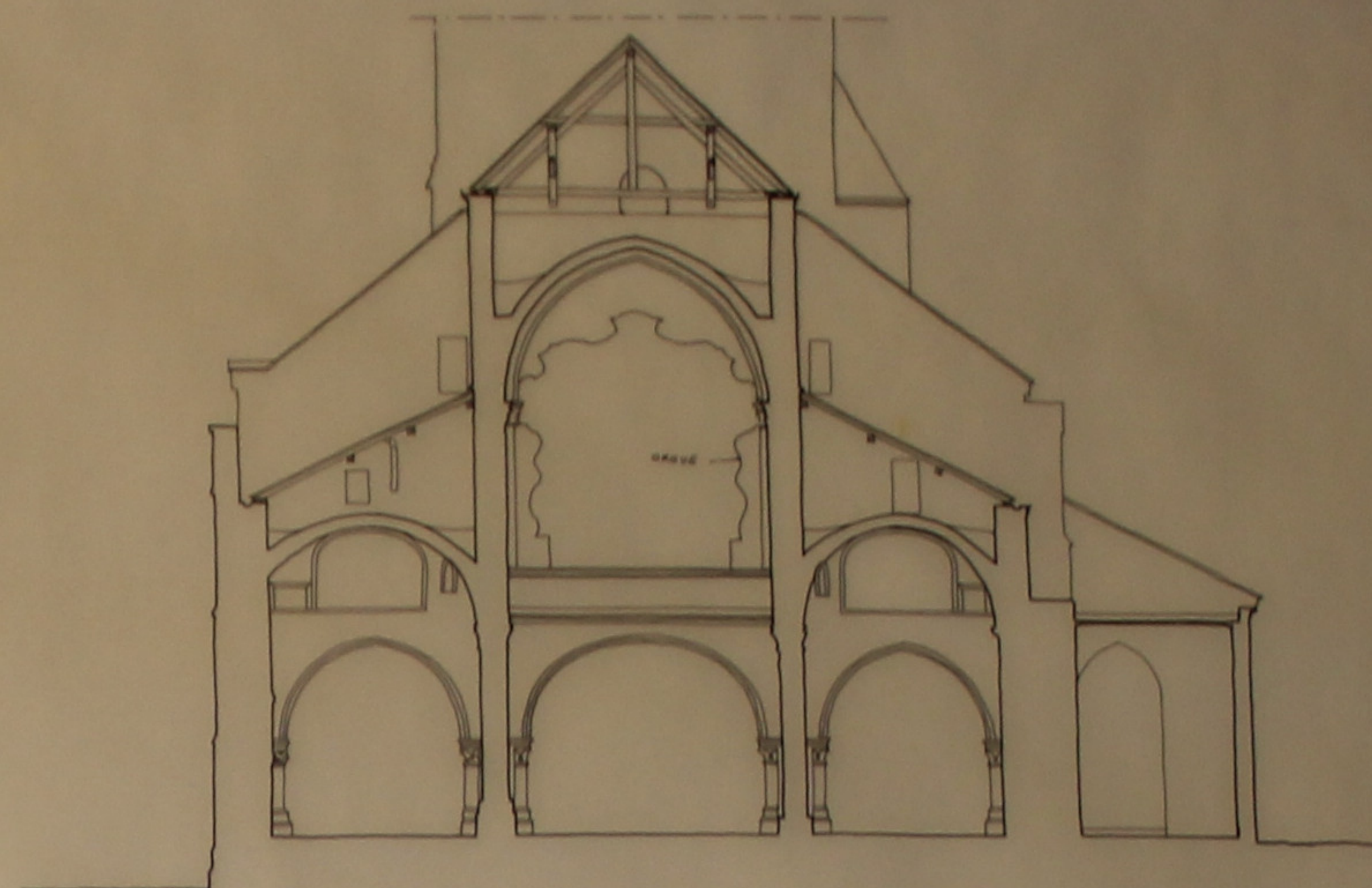
COUPE A-A
