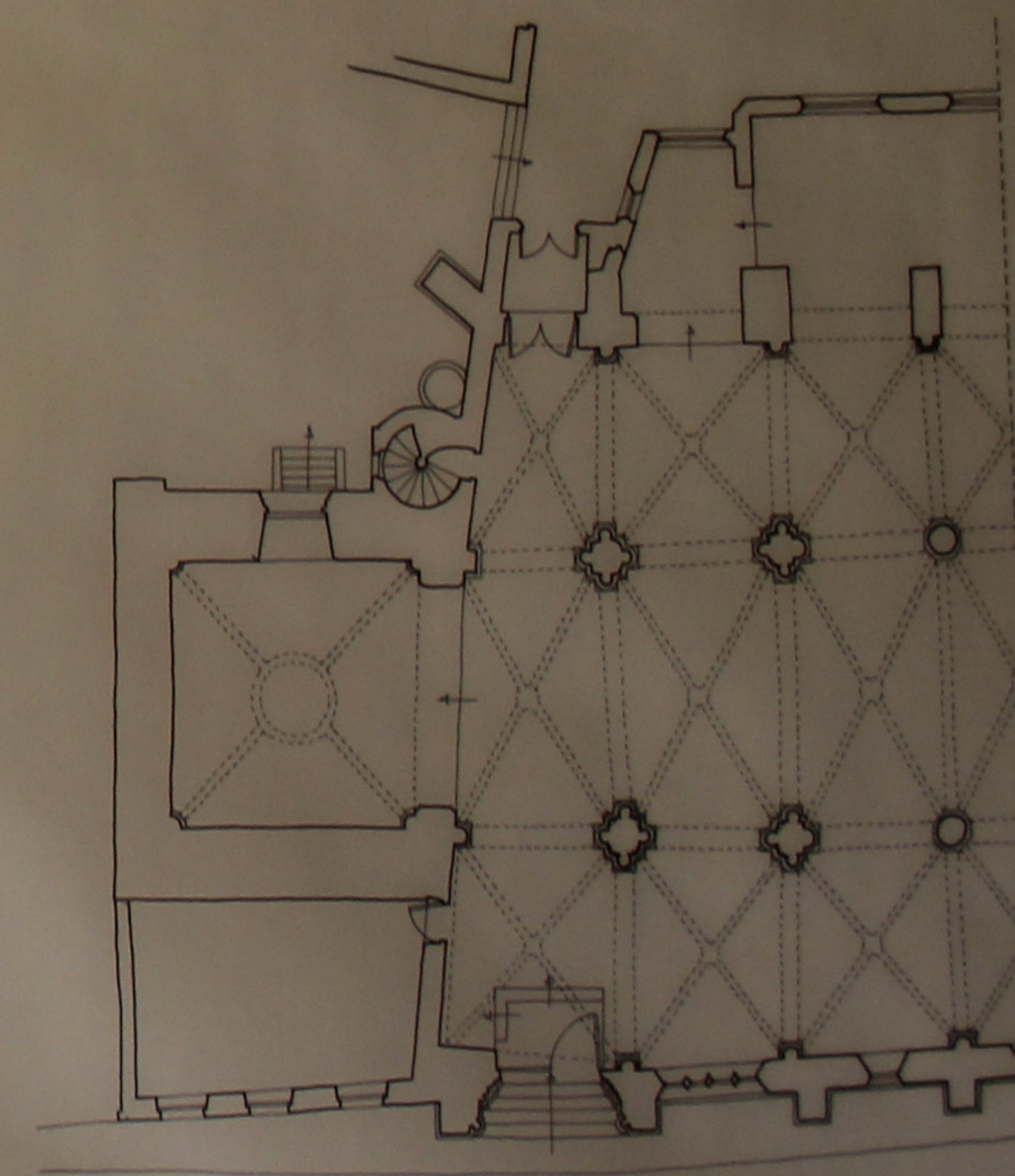
NIVEAU SOL
