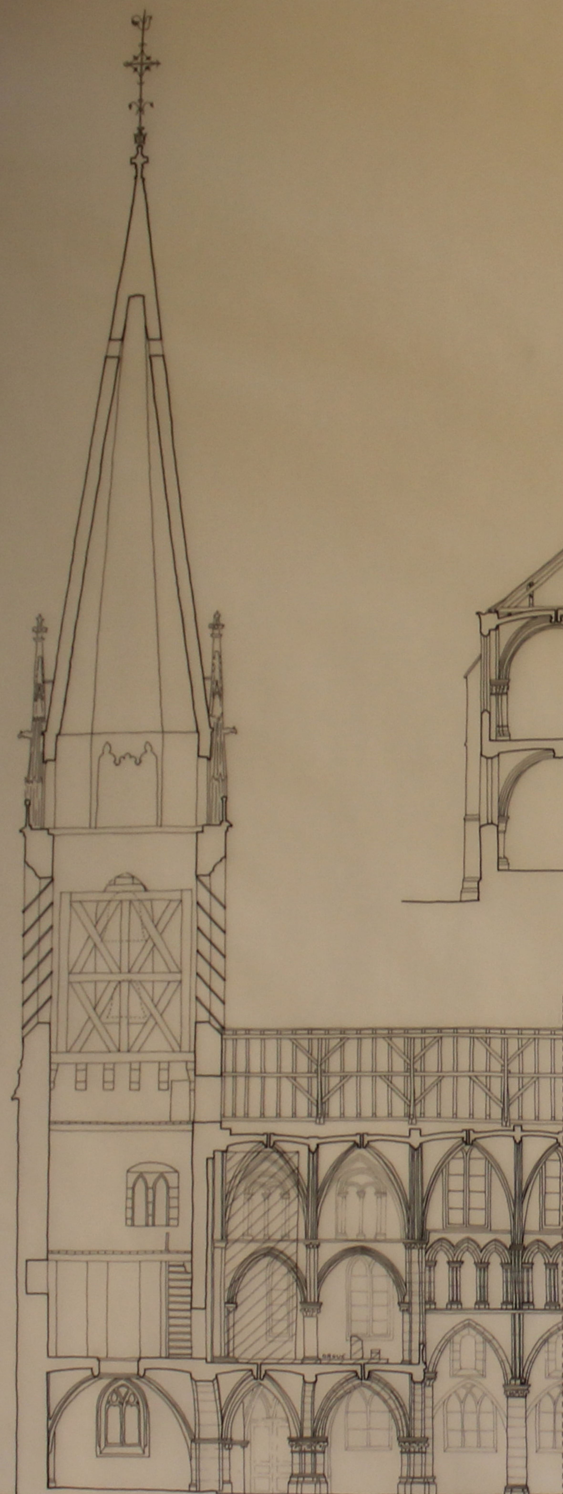
COUPE D-D
