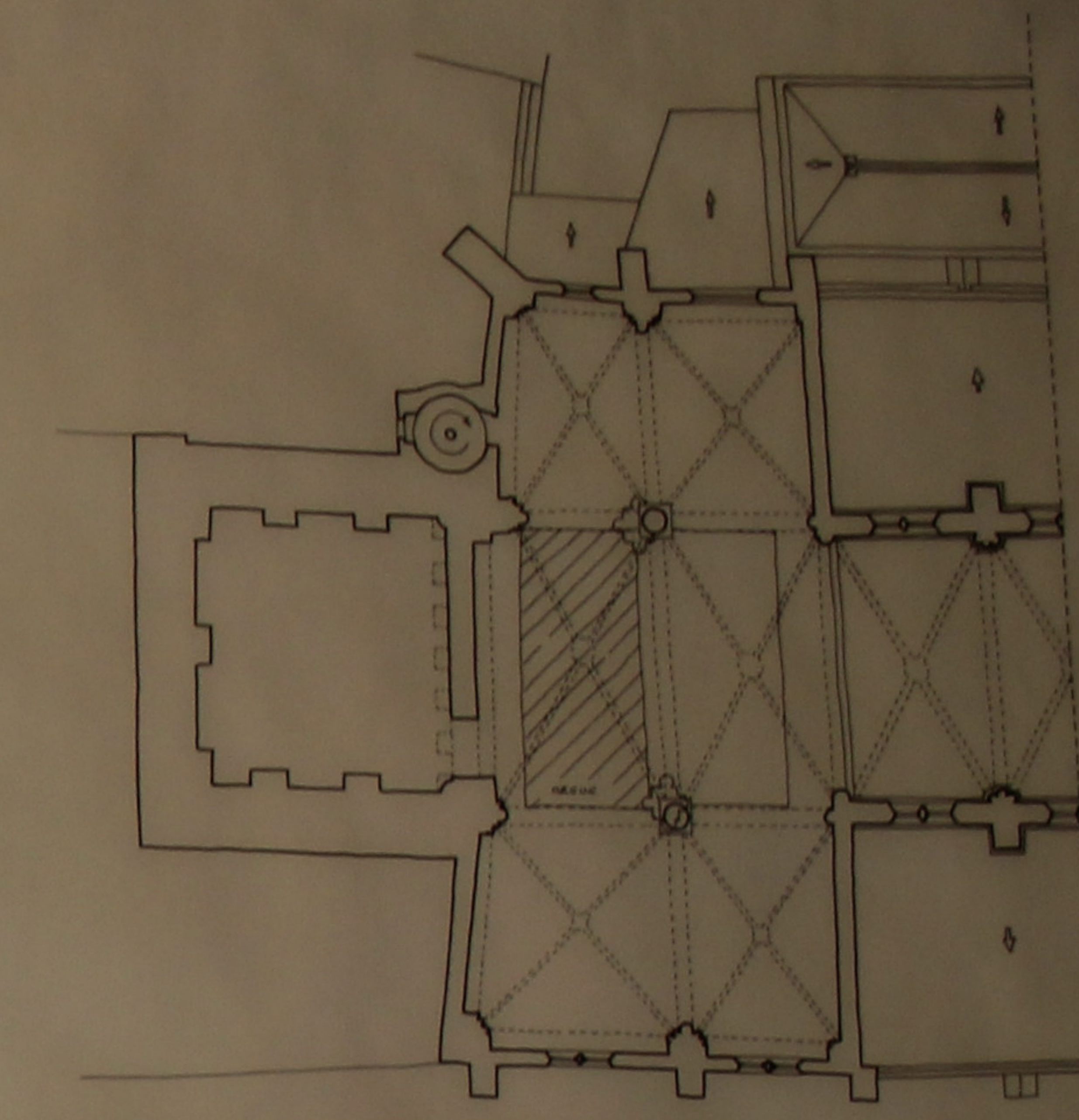
NIVEAU TRIBUNE
