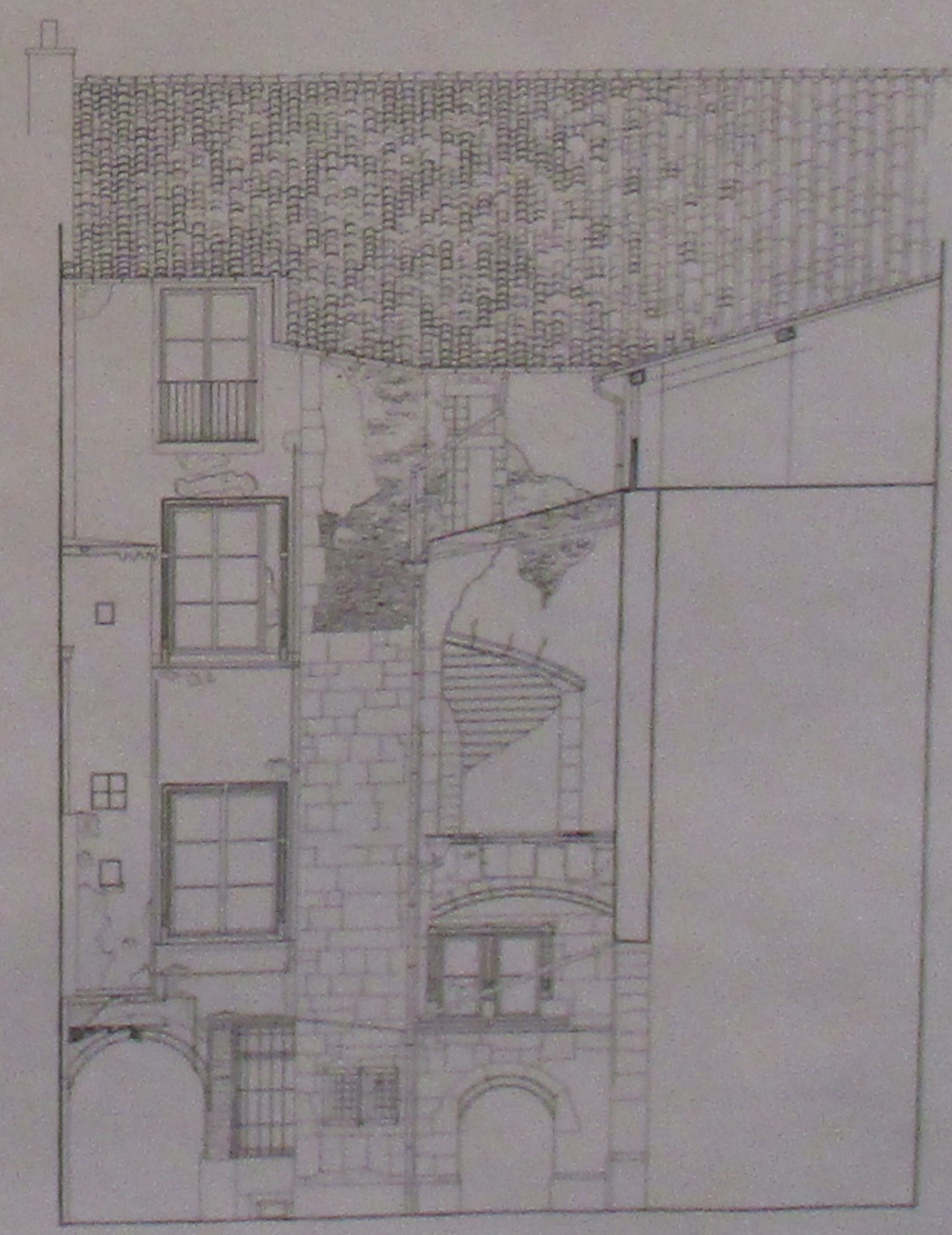
Élévation Est du Logis principal
