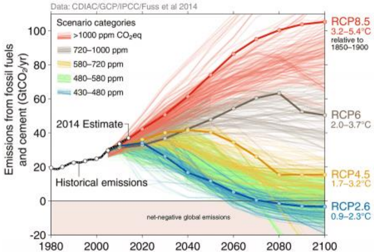
Projection du GIEC, 4 hypothèses, déc 2020
