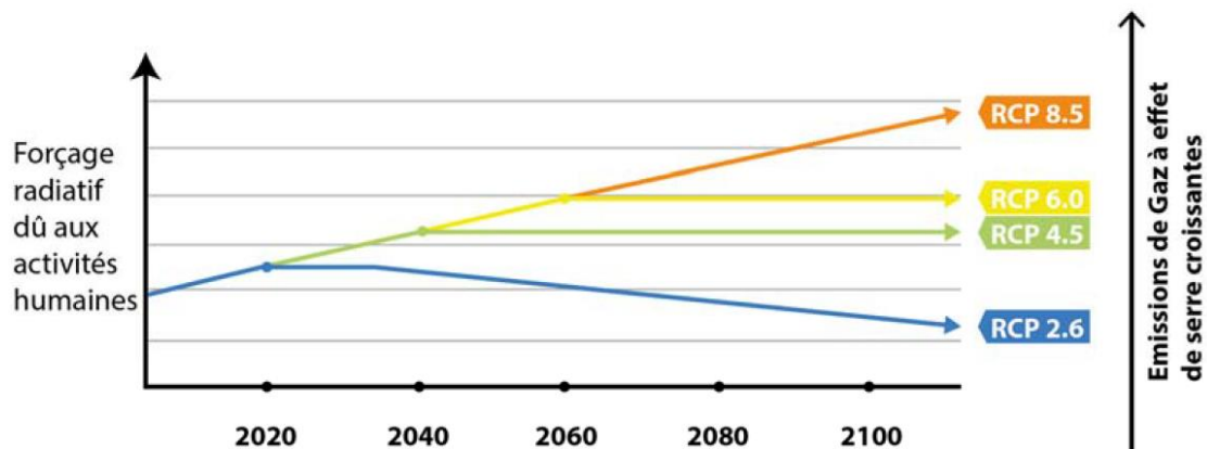
Projection du GIEC, 4 hypothèses, déc 2020
