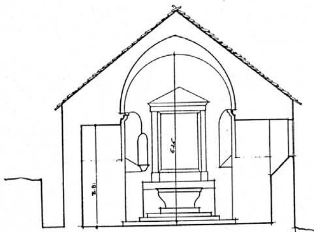
COUPE A.A
