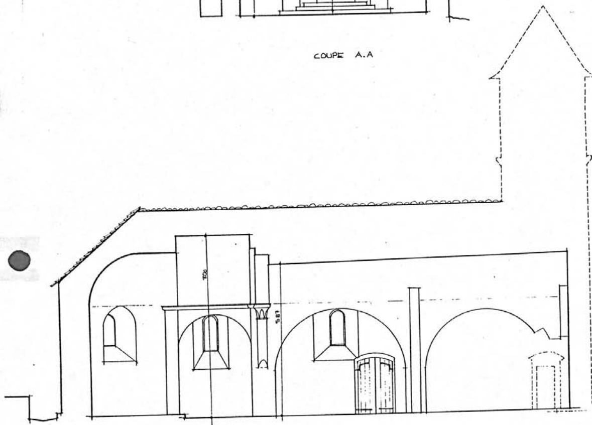
COUPE B.B
